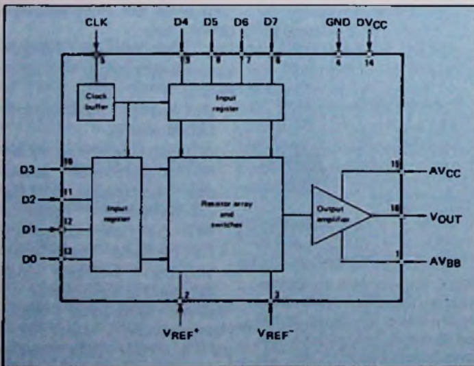
Bild 2: Blockschaltung des D/A-Wandlers
