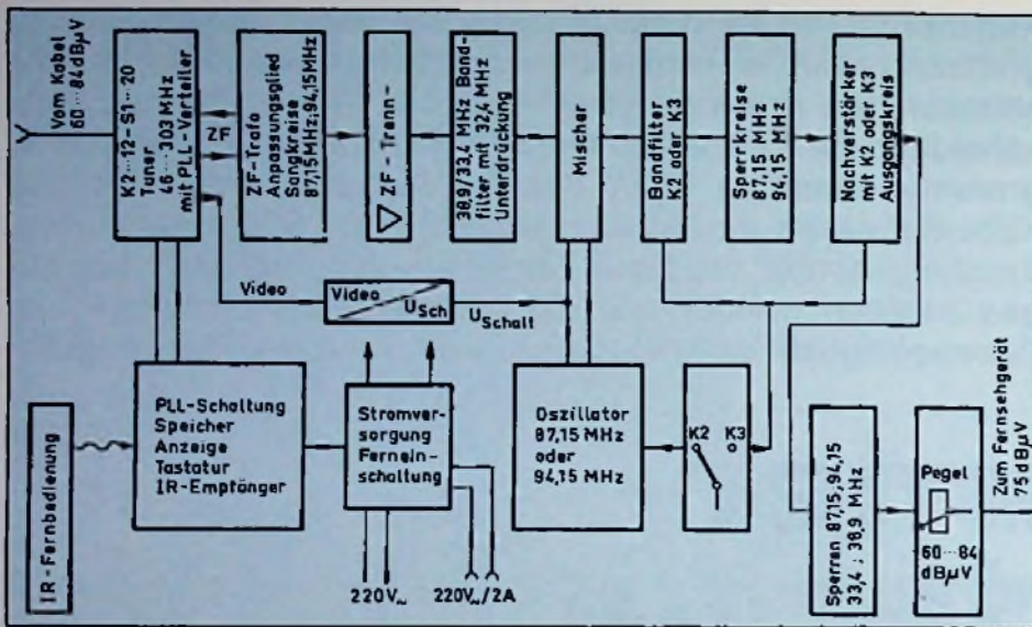
Bild 1: Blockschaubild des Teilnehmer-Konverters TK 02
