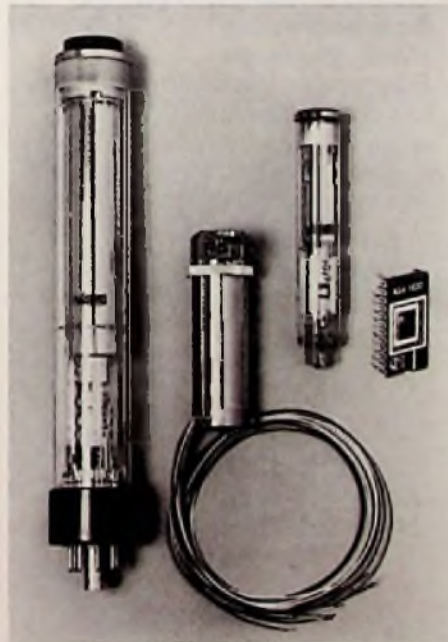
Bild 11: Bildwandler im Generationswechsel: Links ¾-Inch-Plumbicon, daneben ein ½-Inch-Vidikon mit Ablenkjoch, ein ¾-Inch-Newvicon und ein Halbleiterbildwandler (Valvo-Pressbild)
