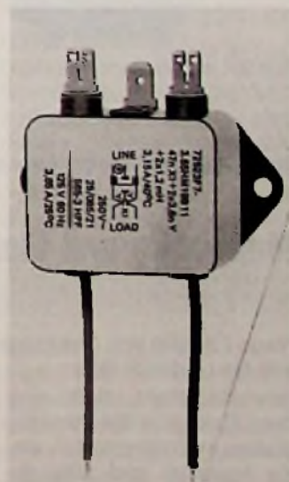
Bild 1: Netzfilter mit hoher Spitzenspannungsfestigkeit (Condensateurs Fribourg-Pressbild)
