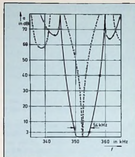
Bild 6: Dämpfungsverlauf des abstimmbaren Doppelquarzfilters im Mittelwellen-Empfänger „C“
