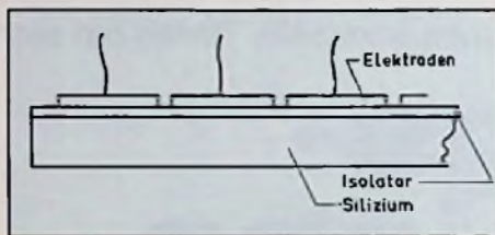
Bild 4: Zellaufbau eines CCD
