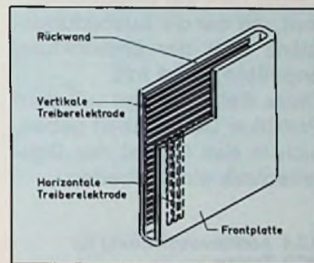
Bild 2: Herkömmliche Matrix-Treiber-Methode
