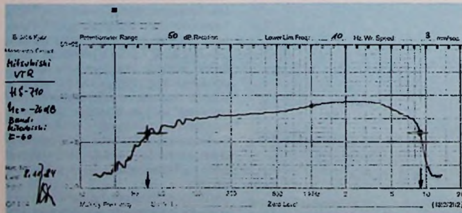
Bild 5: Übertragungsbereich und Frequenzgang (-26 dB) des Audiolotells
