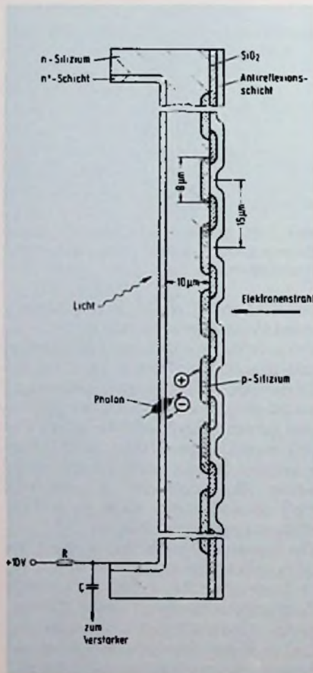
Bild 10: Das Target des Silizium-Multidioden-Vidikons besteht aus einer Million Silizium-Planar-Dioden, die voneinander isoliert sind
