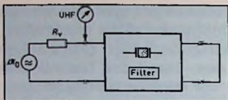
Bild 2: Schaltung für den Filterabgleich; Ausgangskreis kurzgeschlossen
