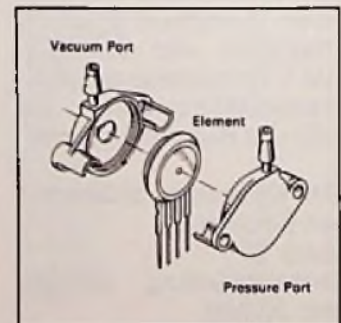
Bild 1: Innenaufbau der Druck- und Differenzdrucksensoren von Motorola
