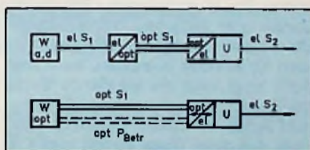
Bild 1: Ein normaler analoger (a) oder digitaler (d) Wandler (W) liefert ein elektrisches Signal, das für faseroptische Übertragung in ein optisches Signal gewandelt werden muß. Ein optischer (opt) Wandler, der gegebenenfalls mit optischer Betriebsleistung versorgt wird, liefert ein solches Signal direkt
