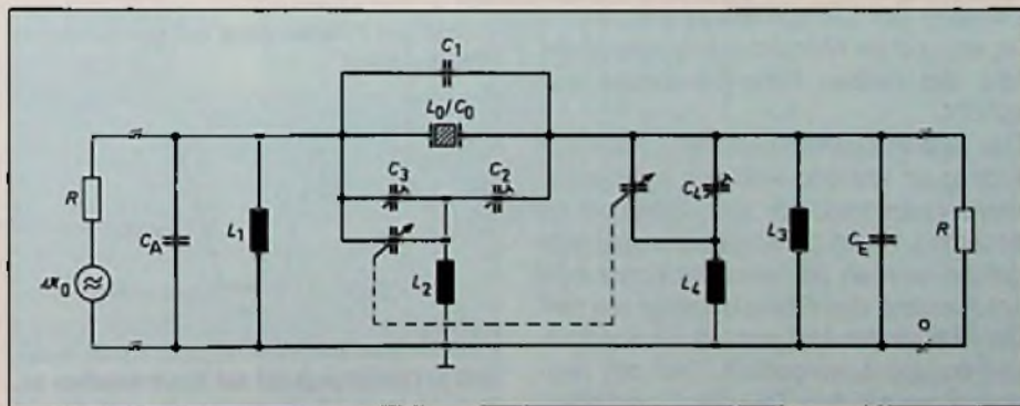
Bild 1: Abstimmbares Quarzfilter mit Gegenspannungs-Neutralisation
