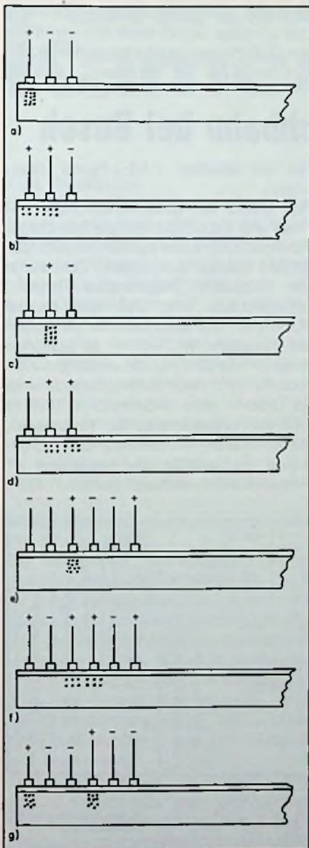
Bild 9: Polaritätsverteilung zwischen den Speicherzellen bei verschiedenen Schiebepulsen
