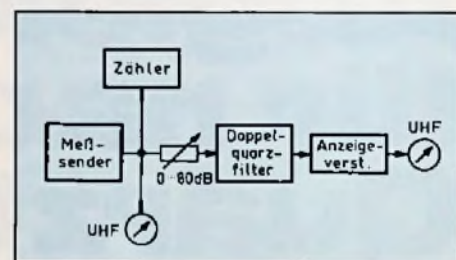
Bild 7: Meßaufbau für Dämpfungsmessungen an einem Doppelquarzfilter
