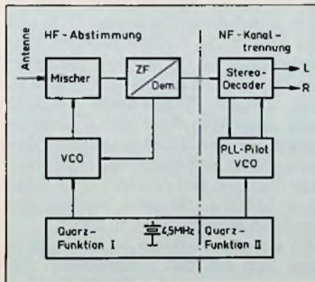
Bild 2: Das Technics Doppel-Quarz-System
