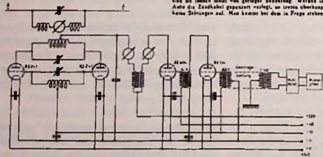
Abb. 1. Der T-Sender.
