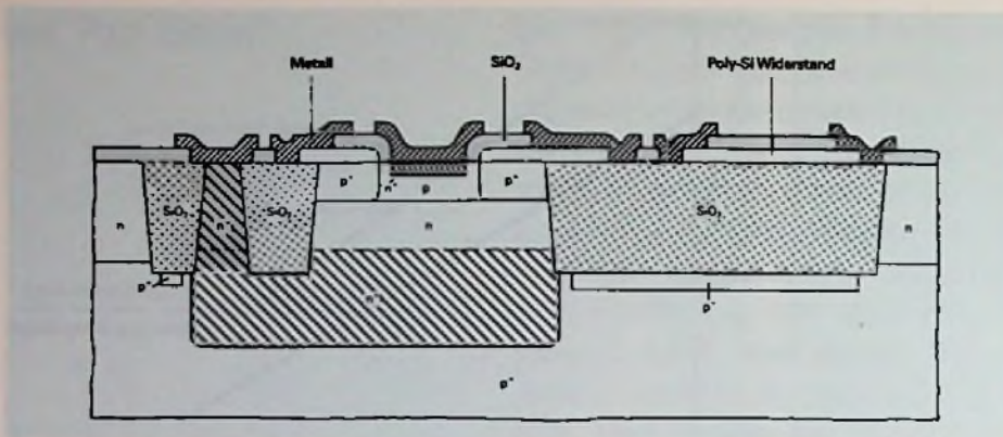
Bild 5: Zellaufbau bei integrierten Schaltungen in UHF-Bipolartechnologie mit Oxidisololation
