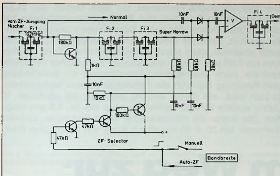
Bild 9: Elektronische ZF-Filter-Umschaltung Normal/Super Narrow
