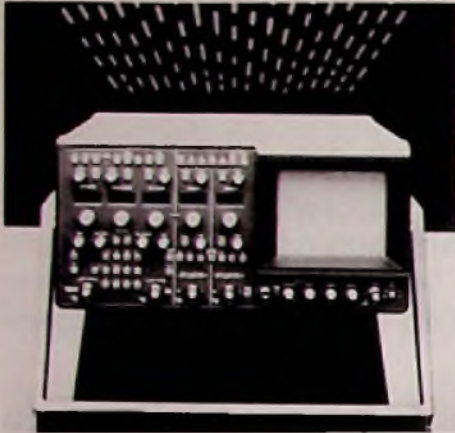
Bild 3: Schnelles Hochfrequenz-Oszilloskop PM 3295 (Philips-Presebild)
