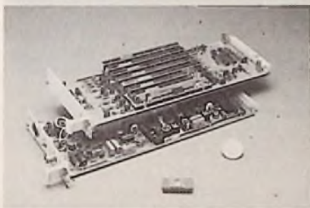
Bild 4: ZF- und NF-Teil des Peilers Telegon 8 als Beispiel für die Reduzierung des Hardware-Aufwandes gegenüber der unten dargestellten herkömmlichen Ausführung mit mechanischen Filtern
