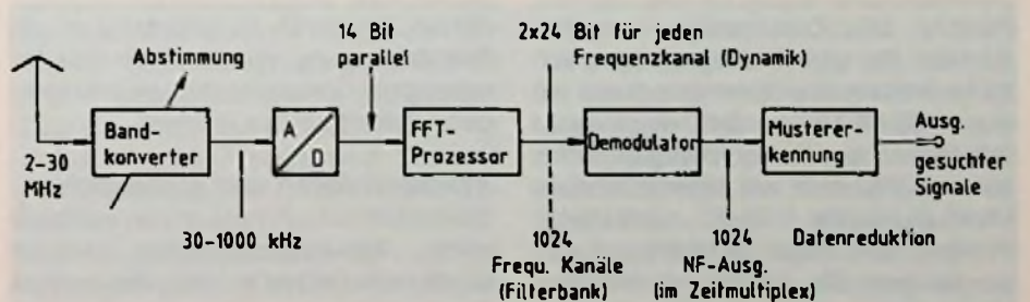
Bild 6: Vielkanal-Parallelempfangsanlage mit schneller Fourier-Transformation
