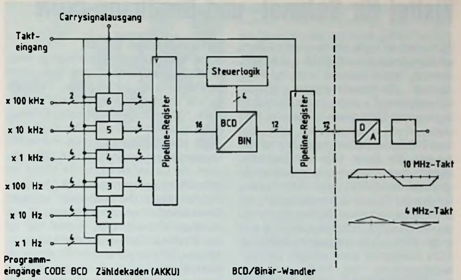
Bild 5: Digitaler Synthesizer 40-60 kHz
