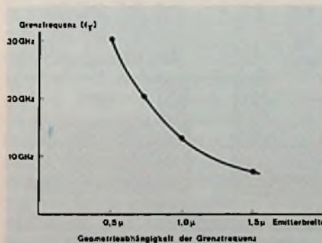
Bild 4: Abhängigkeit der Grenzfrequenz von der Emitterbreite in Halbleiterstrukturen
