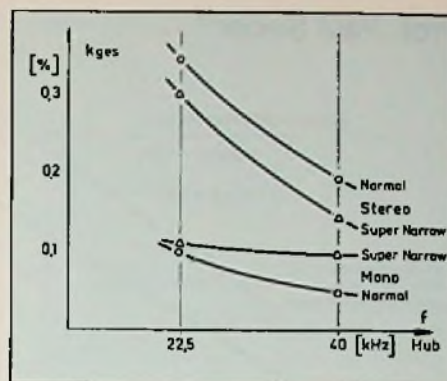
Bild 10: Klirrfaktoren in Abhängigkeit vom Hub bei normaler und begrenzter ZF-Bandbreite
