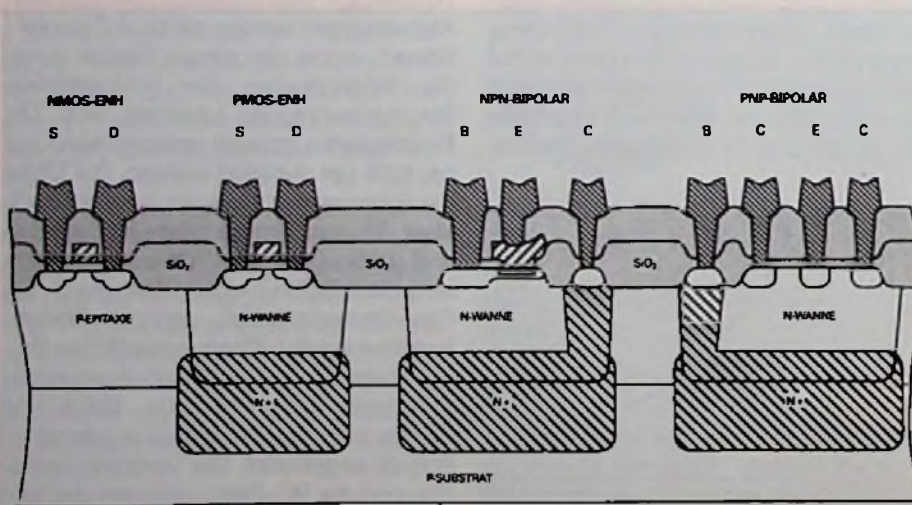
Bild 7: Die BICMOS-Technologie vereint Bipolar- und CMOS-Technik auf einem Chip
