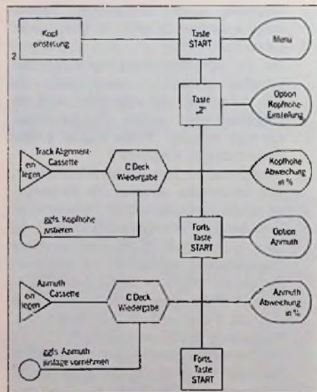
Bild 6: Programmablauf bei der Kopfeinstellung
