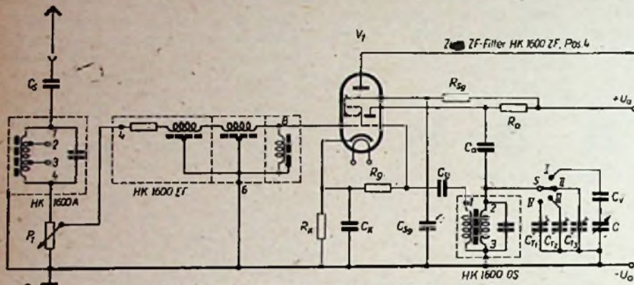
Abb. 1. Mischstufe der Einbereich Superheli.
