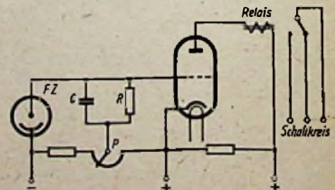
Abb. 4. Schaltrelais mit Fotozelle. Gesteuerte Ausfallzeit. Zeichnungen: Frester
