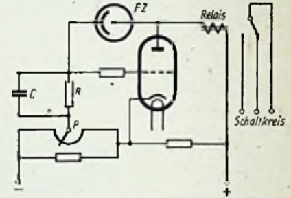
Abb. 3. Schaltrelais mit Fotozelle. Gesteuerte Einfallzeit
