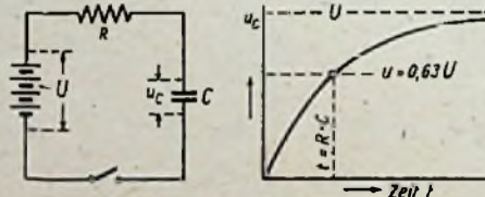
Abb. 1. Aufladen eines Kondensators durch eine Gleichstromquelle. Links: Anordnung. Rechts: Ladecharakteristik
