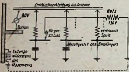
Abb. 4. Verschleppte Berührungsspannungen an Balkonblechen durch schadhaften Rundfunkempfänger
