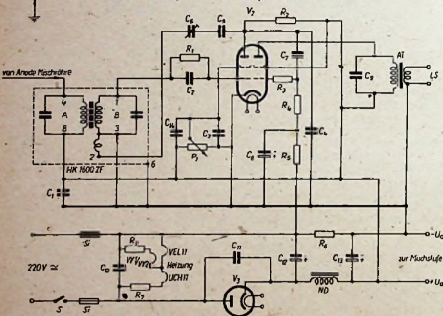
Abb. 2 ZF-, NF- und Netzteil der Allstromausführung
