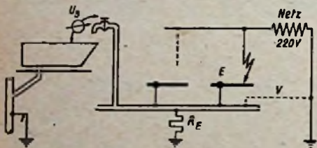
Abb. 5. Verschleppte Berührungsspannung an den Badeeinrichtungen durch vermüllig schadhafte Rundfunkempfänger
