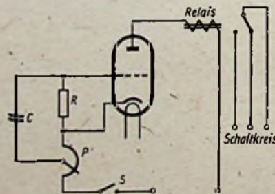
Abb. 2. Mit Verzug schaltendes Relais einfachster Form
