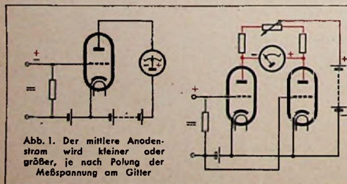
Links: Abb. 2. Durch eine Brückenschaltung mit einer zweiten Röhre werden Speisespannungsschwankungen unwirksam und das Anzeigementromlos
