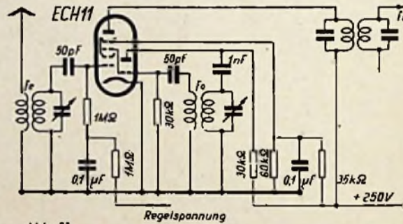
Abb. 21. Mischstufe mit Triode — Hexode, Regelspannung direkt am Gitter
