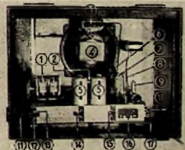
① Drehkondensator, ② UCH 11 und UBF 11, ③ Ausgangstransformator, ④ Lautsprecher, ⑤ Bandfilter, ⑥ UCL 11, ⑦ UY 11, ⑧ U- dox 24 P 10, ⑨ Heizwiderstand, ⑩ Achse der Tonblende, ⑪ Wellenschalterachse, ⑫ Erdan- schluß, ⑬ Antennenanschluß, ⑭ Tonabnehmer- anschluß, ⑮ Anschluß für zweiten Lautsprecher, ⑯ Netz-Umschaltplatte, ⑰ Sicherung
