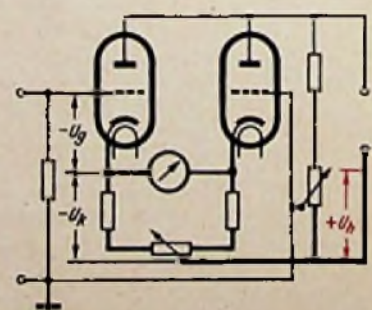
Rechts: Abb. 3. Bei Verlegung der ohmschen Brückenarme in die Katodenleitungen entsteht eine Gegenkopplung und verbessert die Schaltung
