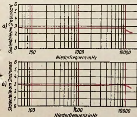
Abb. 3. Niederfrequenzgang
