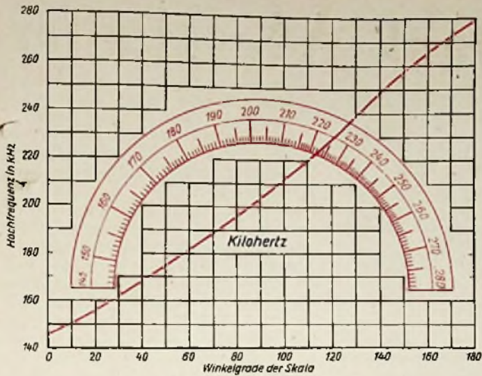
Abb. 2. Hochfrequenzzeichnung
