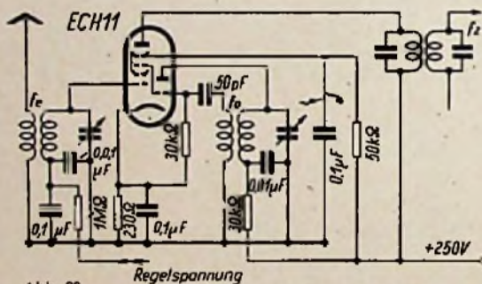
Abb. 20. Mischstufe mit Triode — Hexode, Regelspannung über Schwingkreis
