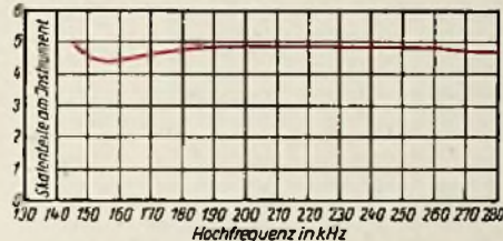
Abb. 4. Hochfrequenzgang
