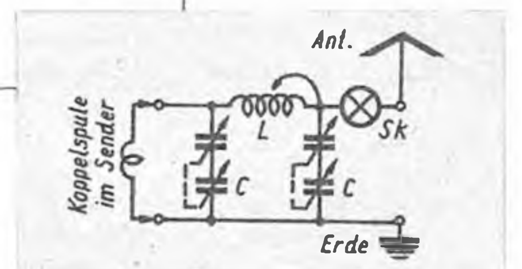
Abb. 1. Schaltbild des zweistufigen Kleinsenders L_1 = 42 Wdg. 0,8 CuL 35 mm \varnothing ; L_2 = 35 Wdg. 0,8 CuL 35 mm \varnothing ; beide dicht gewickelt. L_3 = 10 Wdg. 1,0 CuL 20 mm \varnothing , innerhalb von L_2 im Spulenkörper eingeklemmt
