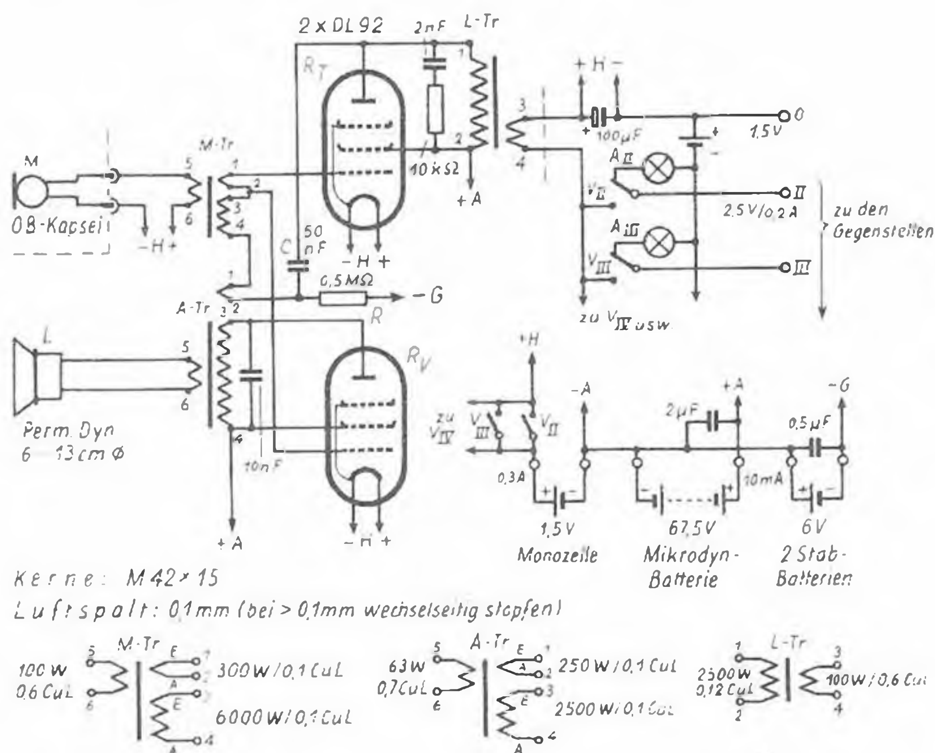
Abb. 2. Laut-Telefonverstärker
