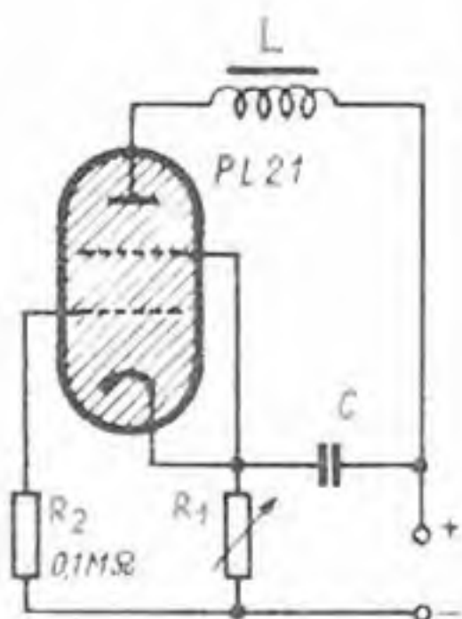
Abb. 5. Einfache Zeitgeber-schaltung mit periodischen, gleichen Zeitintervallen. Abb. 6 (unten). Zeitgeber-schaltung mit zwei periodischen, aufeinanderfolgenden beliebigen Zeiten
