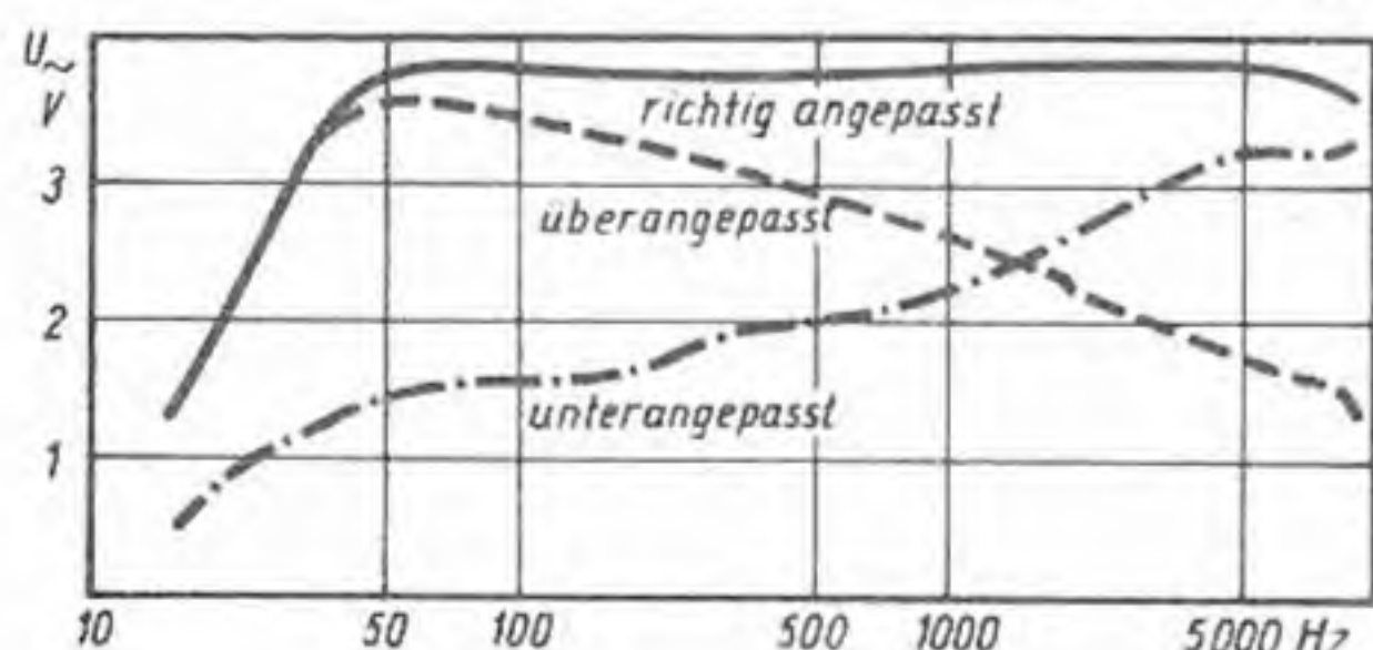
Abb. 2. Abhängigkeit der Schwingspulen - Spannung von der Frequenz bei richtiger und falscher Anpassung der Schwingspule
