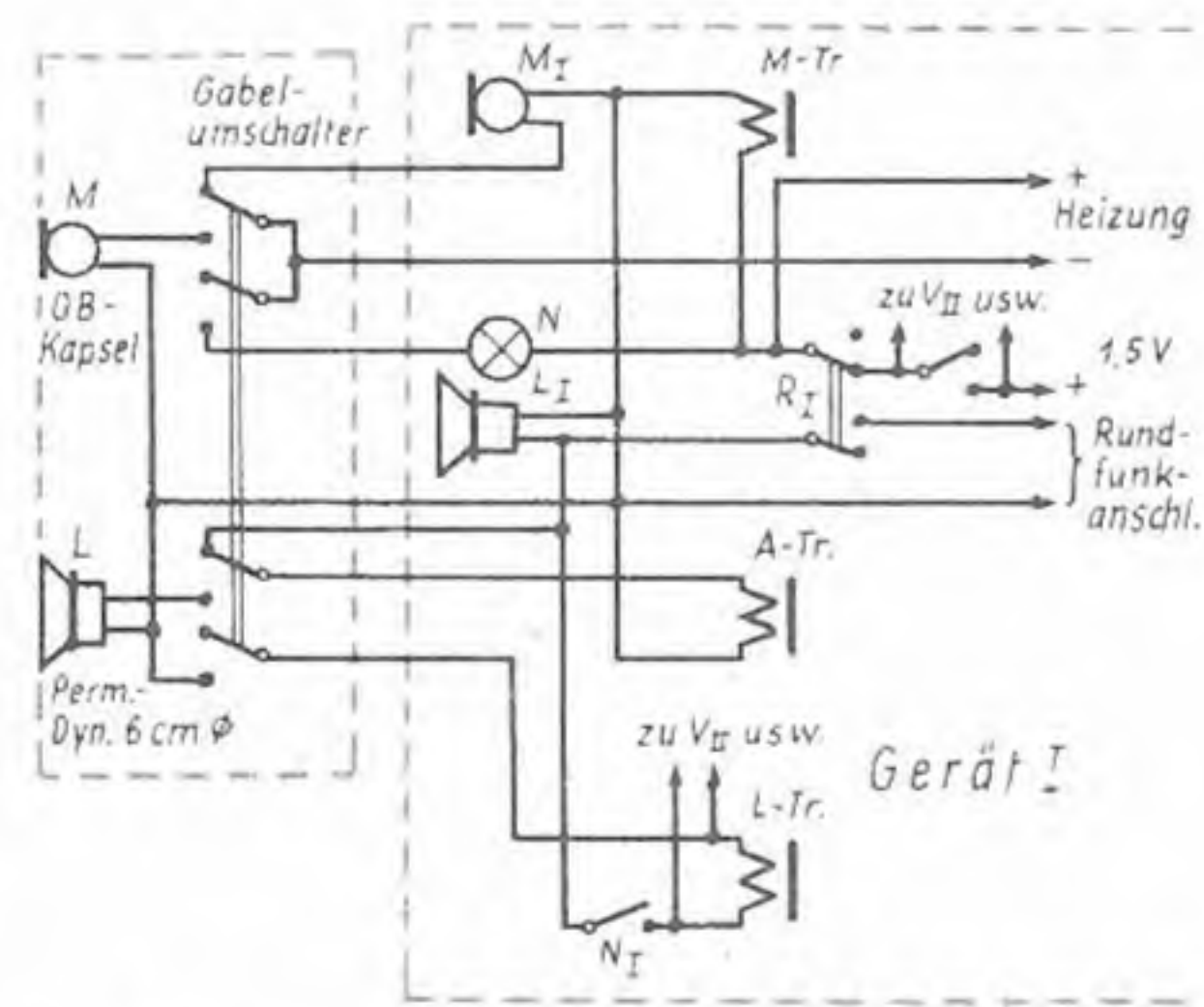
Abb. 6. Fernsprechzusatz
