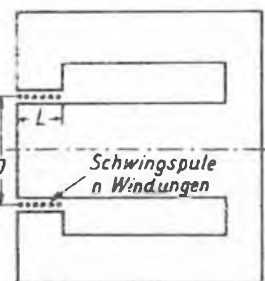
Abb. 1. Querschnitt durch ein Lautsprechersystem
