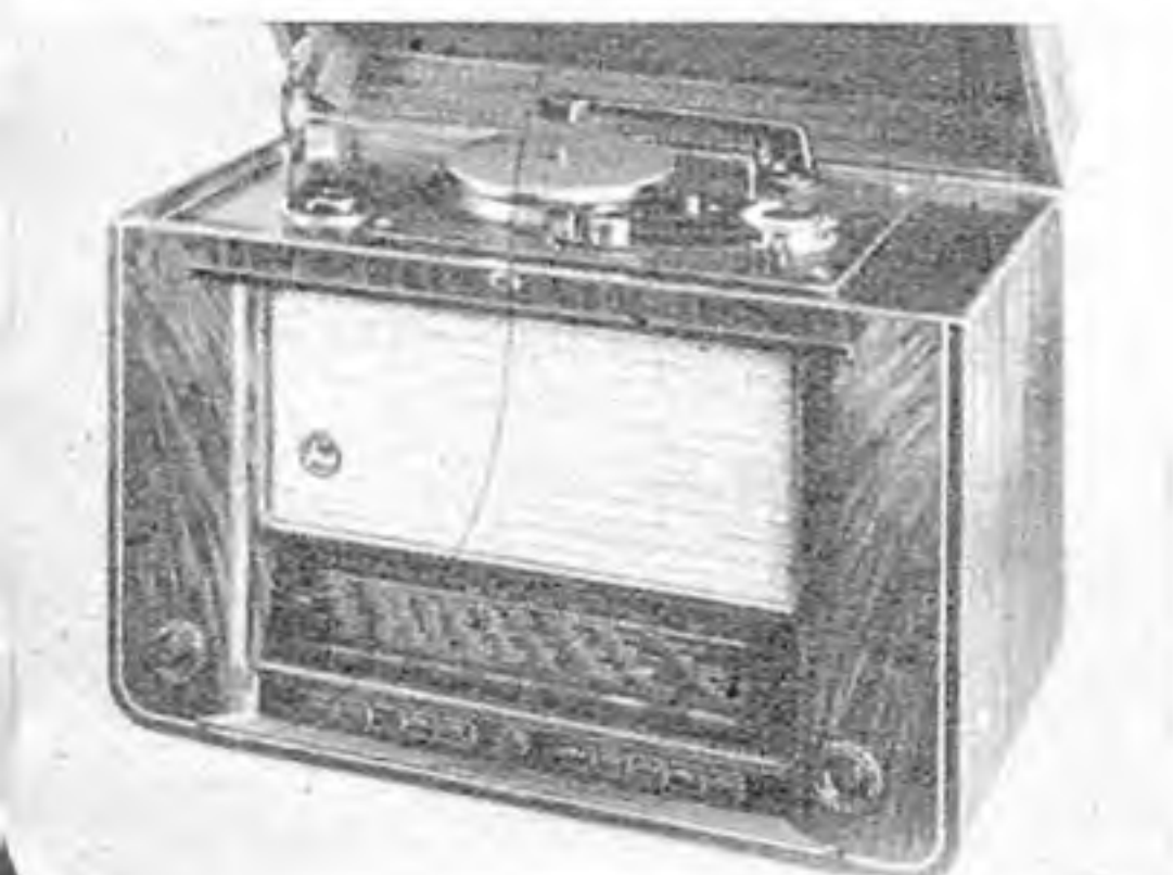
Schaub „Pirolette-Super“, 4 AM-Kreise
