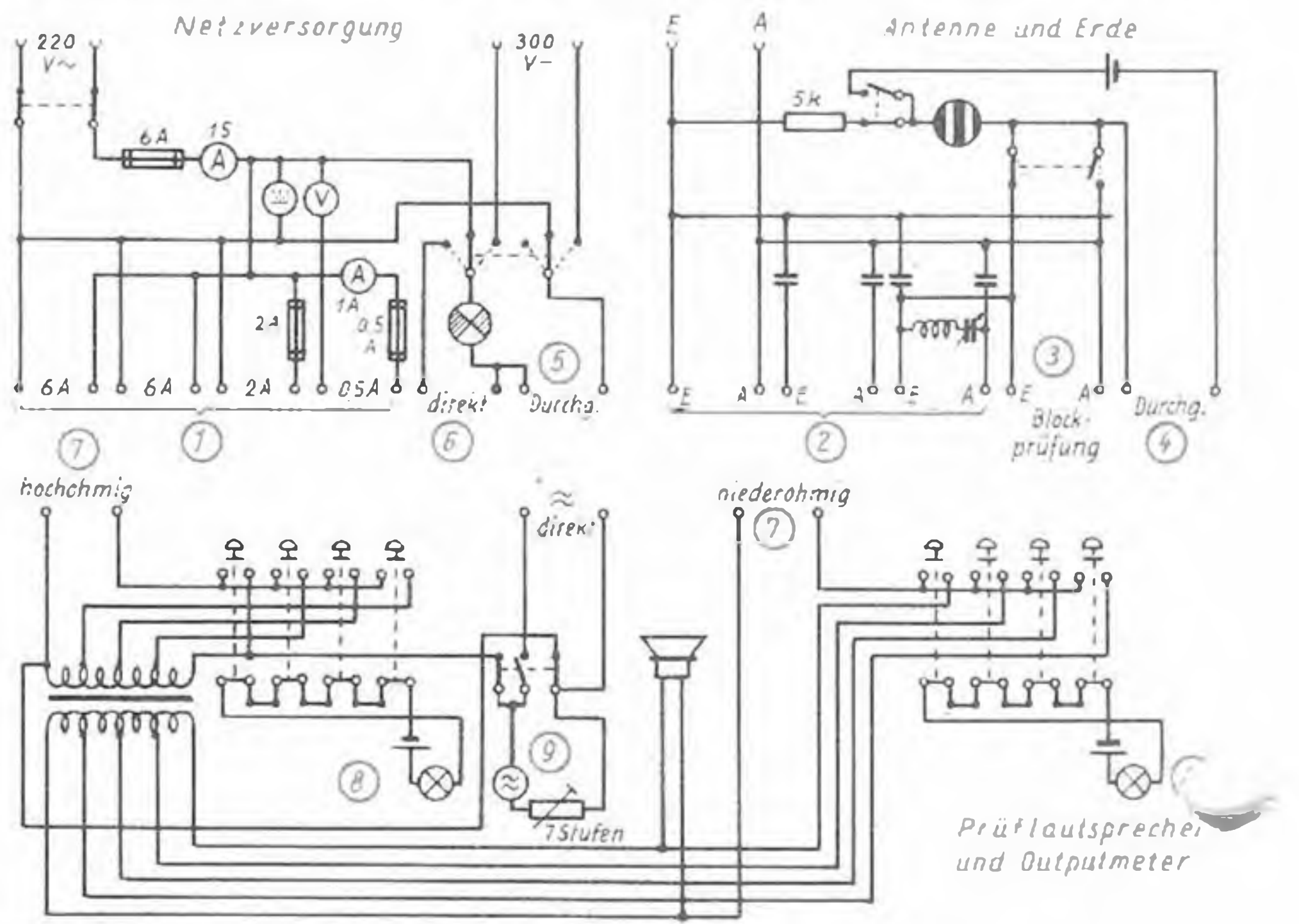
Vorderansicht und Schaltbild der Prüfeinrichtung
