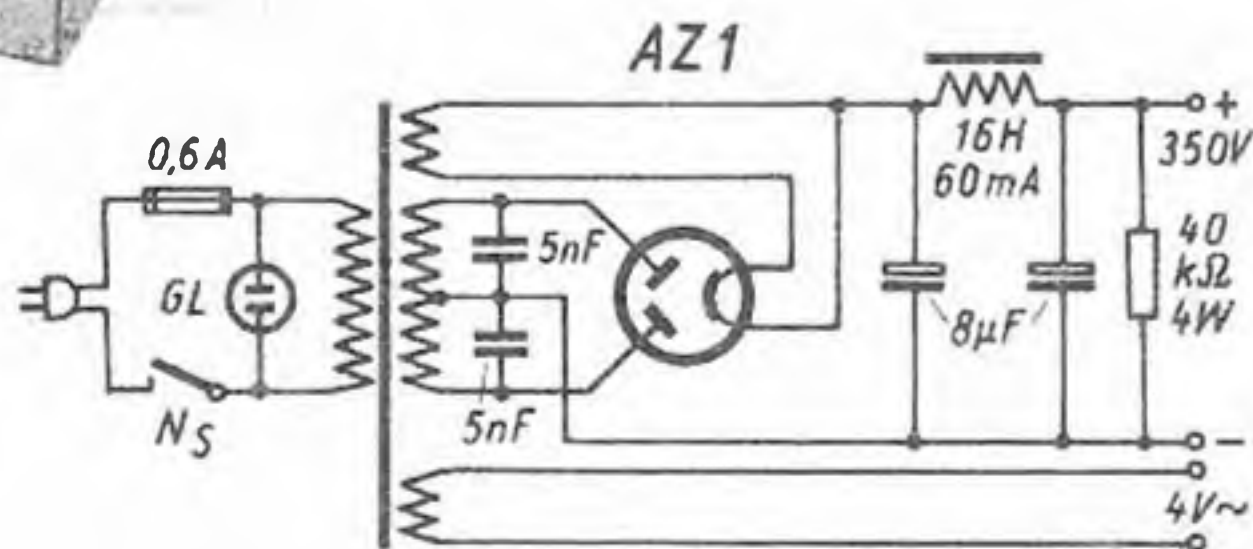
Abb. 6 (unten). Schaltbild des Netzgerätes, das durch den getrennten Aufbau gegebenenfalls auch zur Stromversorgung des Empfängers benutzbar ist
