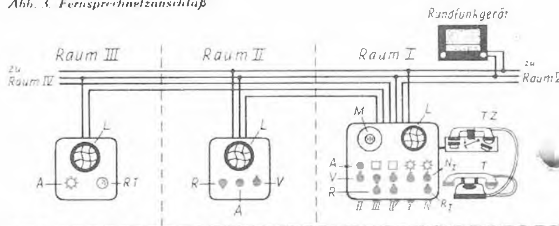
Abb. 3. Fernsprechnetztanschluß
