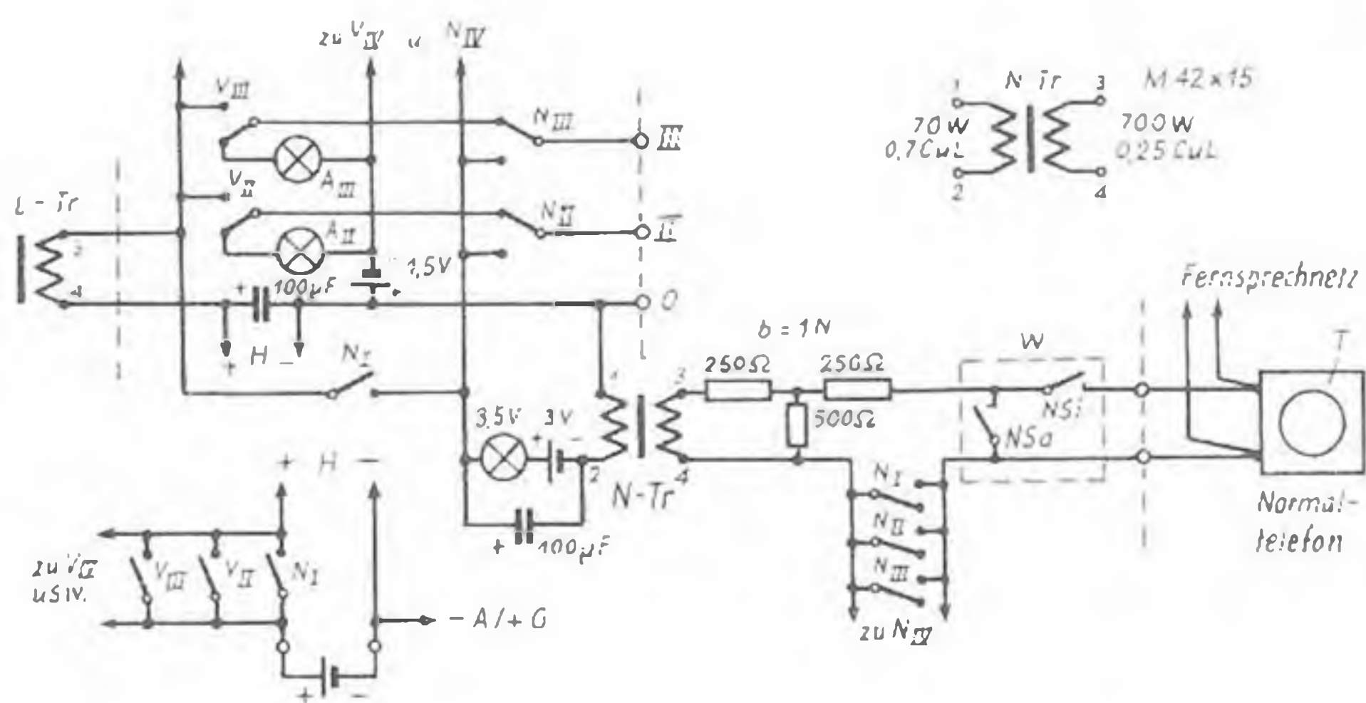
Abb. 3. Fernsprechnetztanschluß
