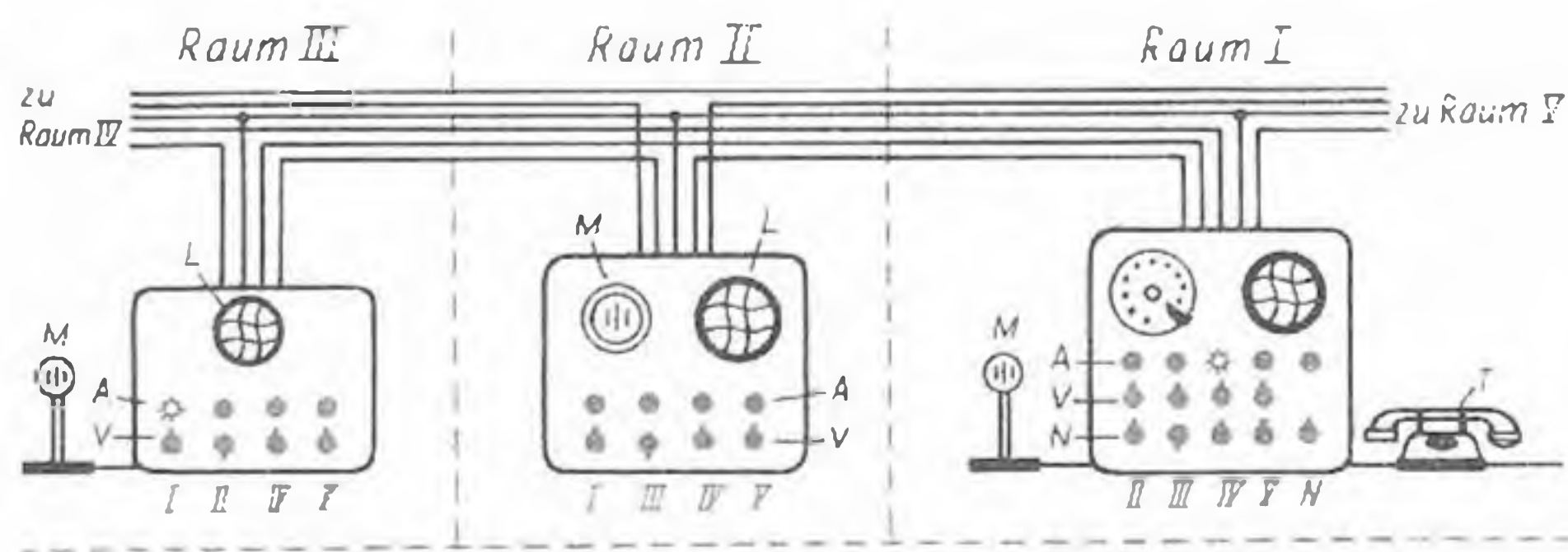
Abb. 1. Haus-Lauttelefon-Anlage
