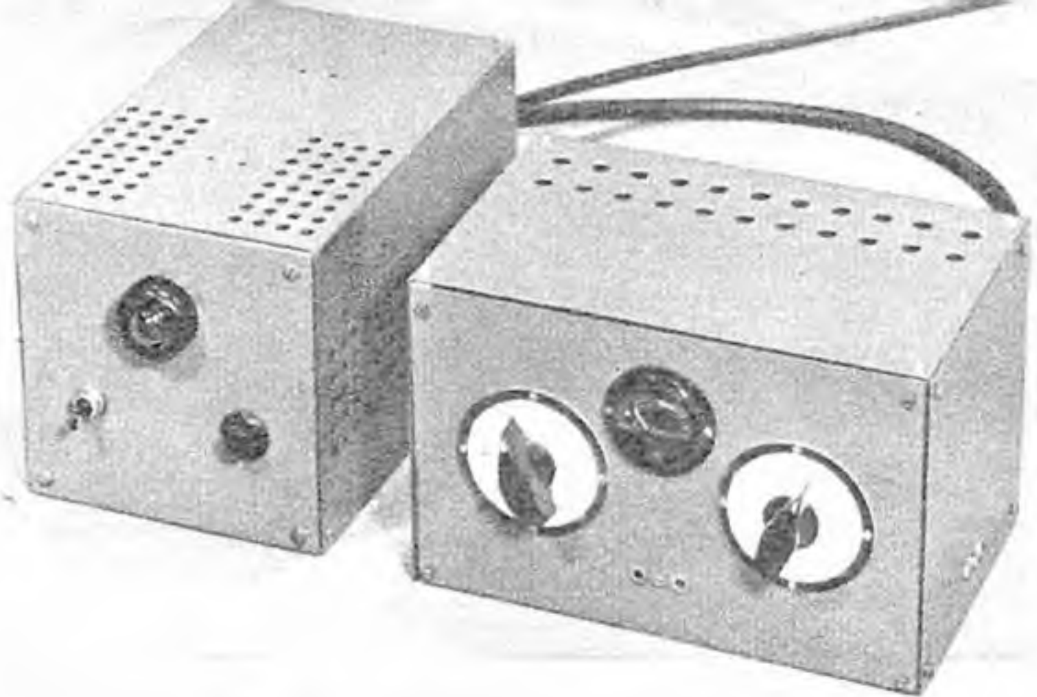
Abb. 5. Ansicht des fertigen Kleinsenders; links das getrennt aufgebaute Netzgerät. Als Abstimmskalen am Sender dienen die bekannten Kreisskalen mit 100"-Teilung und 70 mm \varnothing . Das Buchsenpaar in der Mitte unten ist der Tastanschluß
