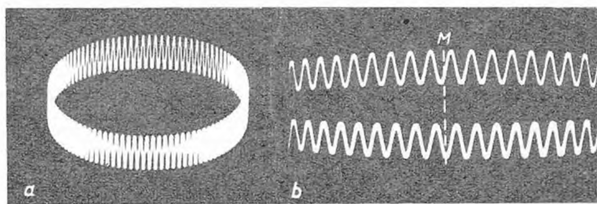
Abb. 14. Bestimmung der Frequenzdifferenz bei großen Unterschieden durch Vergrößerung der X-Spannung
