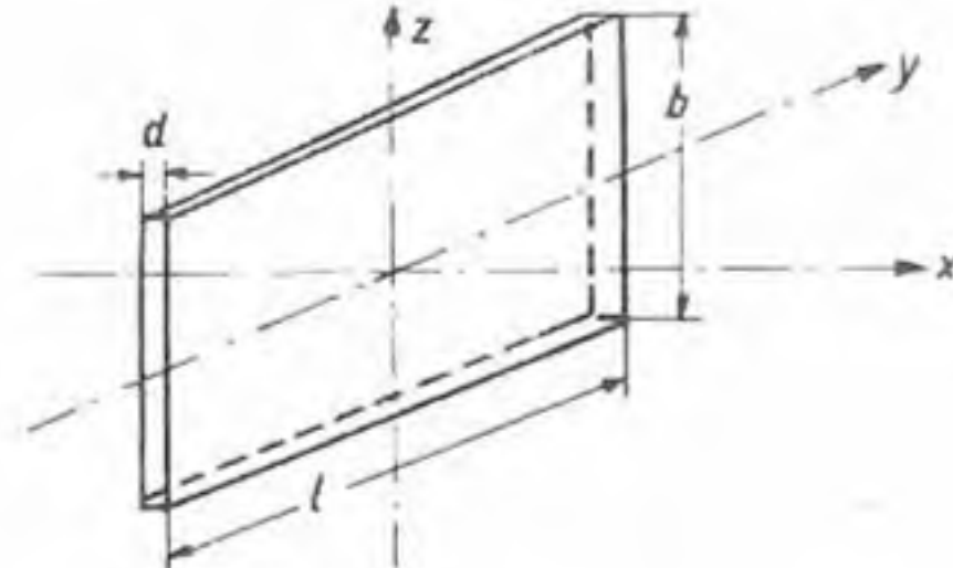
Die 3 Achsen des Quarzkristalles
