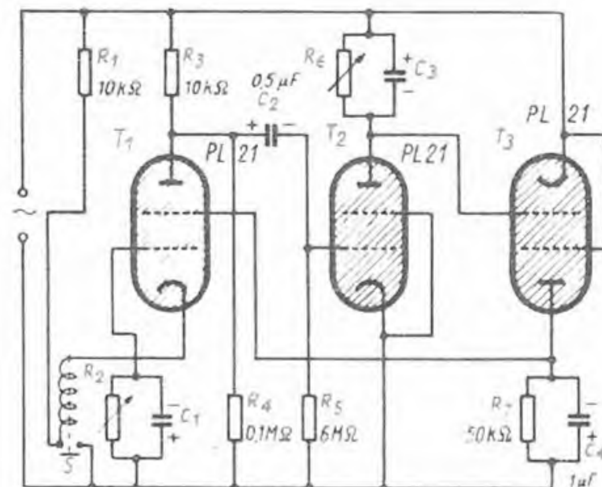
Abb. 4. Zeitgeberschaltung mit zwei aufeinanderfolgenden und unabhängig voneinander einstellbaren Zeiten
