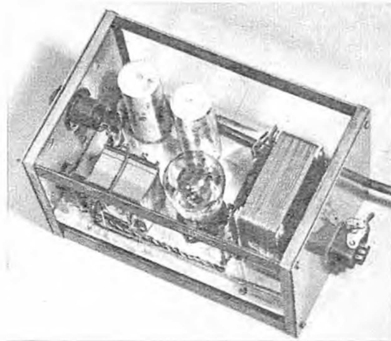
Abb. 7. Auch das Netzgerät ist mit normalen Einzelteilen in einen ebensolchen Blechkasten wie der Sender eingebaut. An der Vorderseite befindet sich der Netzschalter, das Sicherungselement und die Signallämpfchen, während ein Mehrfachstecker hinten für den Anschluß des Vierfachkabels zum wie beschrieben aufgebauten Sender vorgesehen ist
