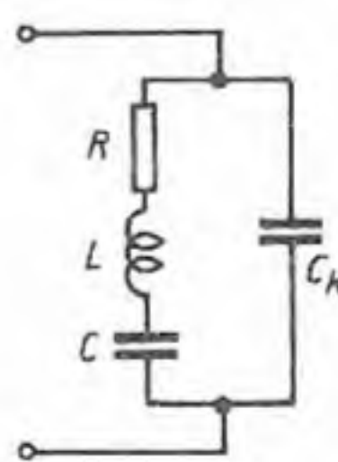
Schwingquarz-Ersatzschema
