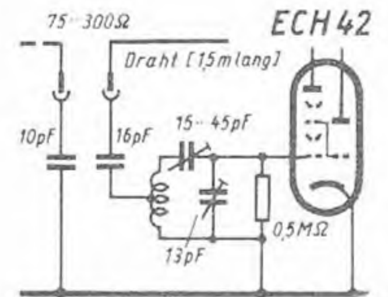
Unsymmetrischer Antenneneingang bei UKW im Nord-Mende 186 WU
