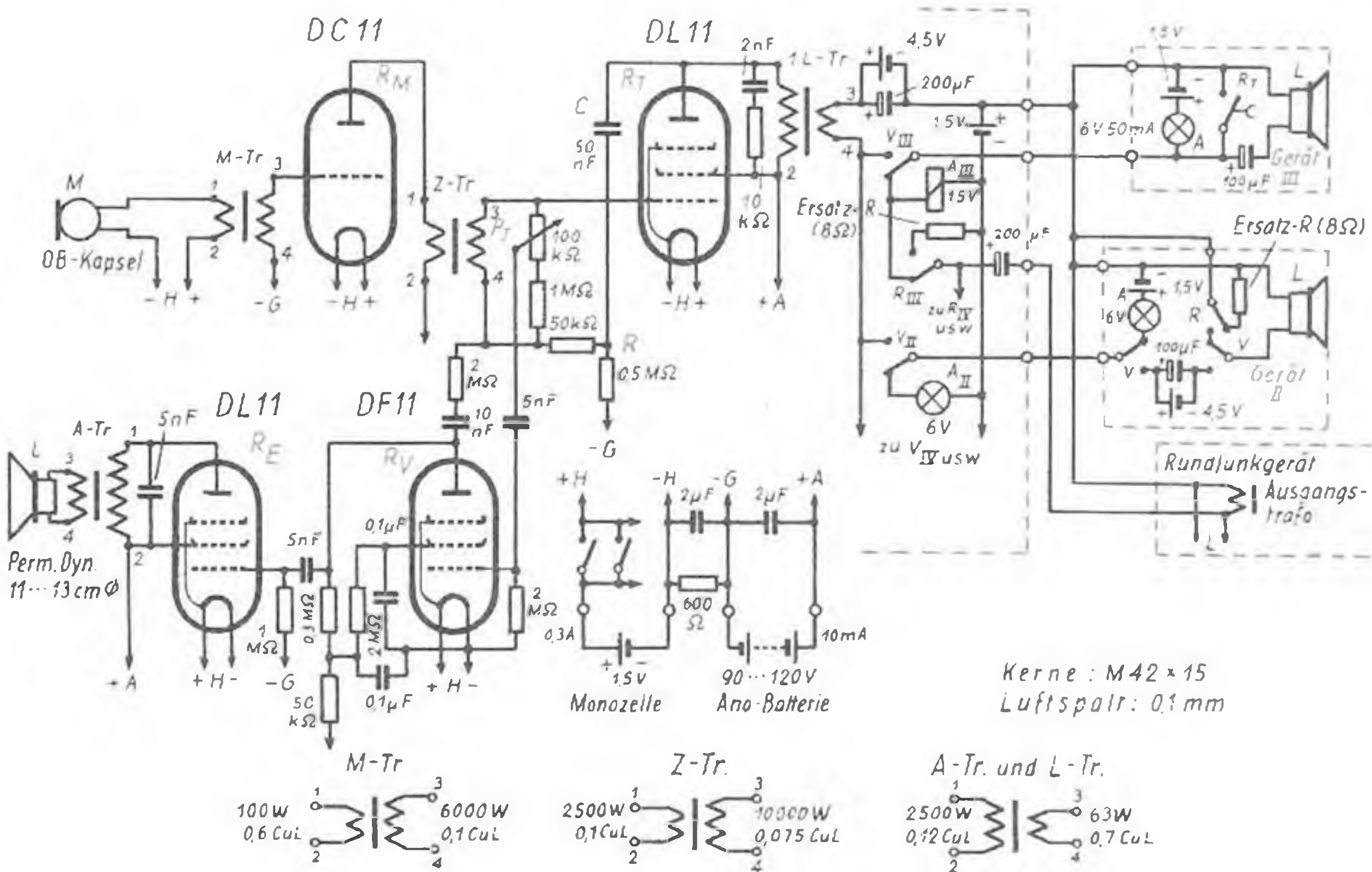
Abb. 5. Nebenstellen-Verstärker
