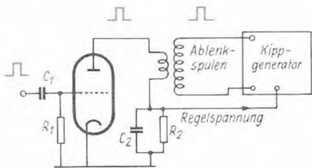
Abb. 9. Prinzip der Regelsynchronisierung
