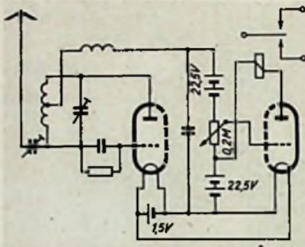
Abb. 7. Pendelaudio mit nachgeschaltetem Gleichstromverstärker
