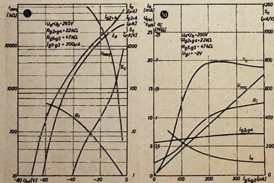
Abb. 5c u. d. ECH 81, UCH 81. Heptodenkennlinien für den Einsatz als Mischröhre: c) I_a , I_{g2+4} , S_c und r_{aec} in Abhängigkeit von U_{gl} ; d) S_c , U_{osc} , R_i , I_{g2+4} und I_a in Abhängigkeit von I_{g1+3}
