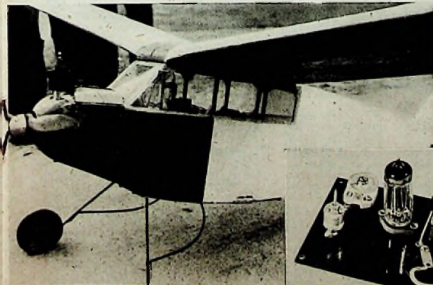
Abb. 5. Aufbau eines Pendelaudions auf einem kleinen Perlinaxbrettchen (Ober- und Untersicht). Im Flugzeugmodell ist der Empfänger, wie an der herausragenden Röhre erkennbar, hinter der Windschutzscheibe an elastisch verspannten Gummifäden aufgehängt. Größe der Platte etwa 6 x 13 cm
