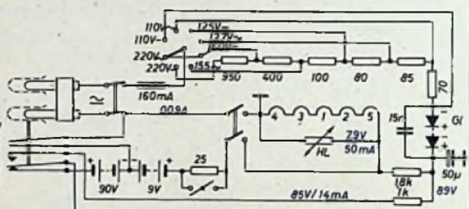
Ströme und Spannungen mit UVA 833 \Omega/V bei 220 V ~ gemessen
