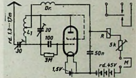
Abb. 4. Empfängerschaltung mit Pendelaudion. L_1 = 8 Wdg., 1,5 Cu, 20 mm \Phi , Mittelabgriff. Dr = 60 Wdg., 0,8 CuL, 7 mm \Phi
