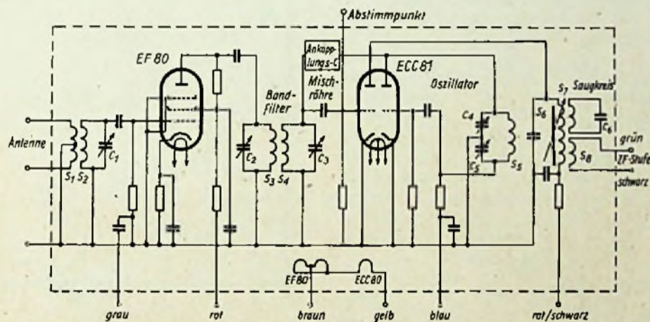
Abb. 3 (links). Schaltung des Kanalwählers. Abb. 4 (oben). Feinabstimmung; (a) 1. ZF-Filter (Bild-ZF 21,5 MHz, Ton-ZF 18 MHz), (b) EF 80, (c) ECC 81 (unter Abschirmung)
