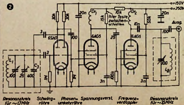
Abb. 2. Vollständiges Schaltbild eines abstimmbaren Franklin-Oszil- lators für das 3,5-MHz-Band. C_1 = keram. Kondensator mit nega- tivem TK; D_{r1} und D_{r2} = HF- Drosseln 2,5 mH; L_1 = 50 Wdg. 0,5 mm \Phi auf 15 mm \Phi ; L_2 = 45 Wdg. 0,5 mm \Phi auf 18 mm \Phi
