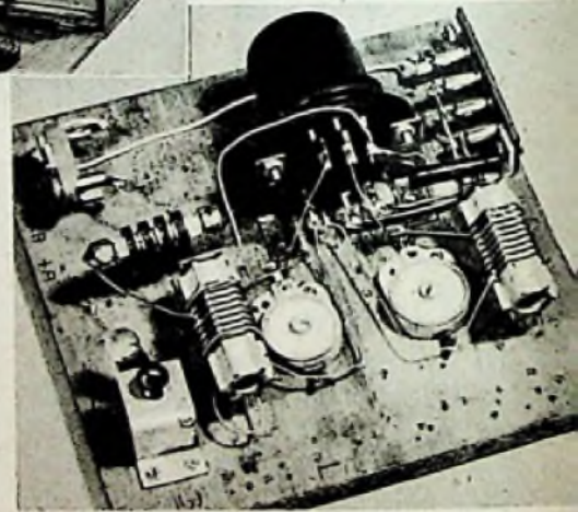
Abb. 2. Schaltung eines Huth-Kühn-Gegentaktsenders. R je nach Röhren und Anodenspannung 2...10 kOhm. L_2 = 9 Wdg., 1,0 Cu; 20 mm \Phi ; 2 mm lang. L_3, L_4 je eine Wdg. an den Enden von L_2 . Links endgültiger Aufbau eines tragbaren Senders mit 2 x RL 4,2 P6 und eingebauten Trockenbatterien. Unten Versuchsaufbau mit EDD 11 für Zerkhaderbetrieb
