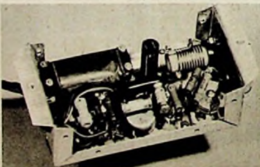
Abb. 10. Für Modellsteuerung geeignete Relais. Links außen polarisierte Ausführung, von denen für Steuerzwecke T. rls 64 b bzw. 67 b geeignet sind. Ersteres ermöglicht einen einstellbaren Ruhestromkreis. Als Wicklung wäre die T. Bv 3302/16 vorzuschlagen. Daneben ein Klappankerrelais kommerzieller Herkunft ( R_i = 15 kOhm) und vorn T. rls 151a von Siemens
