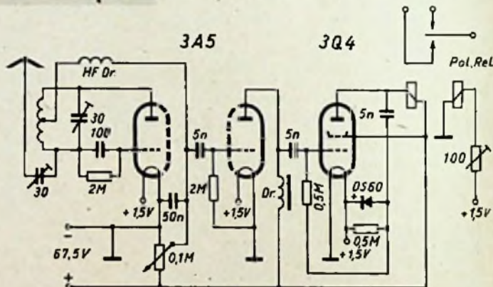
Abb. 7. Pendelaudio mit nachgeschaltetem Gleichstromverstärker
