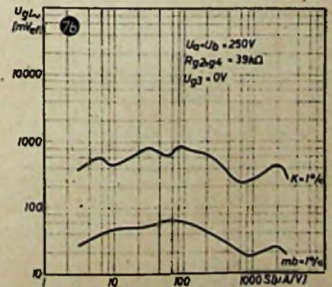
Abb. 7a u. b. ECH 81, UCH 81. a) Kreuz- und Brummodulation bei Verwendung als Mischröhre, b) desgl. als HF- oder ZF-Verstärker
