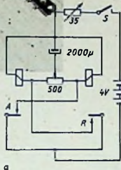
Abb. 3. Elektrisches Tastgerät mit zwei 4-Volt-Relais. Arbeitskontakte zur Senderlastung nicht gezeichnet. Oben: Versuchsaufbau. Rechts: Darstellung des Tastverhältnisses zur Proportionalsteuerung
