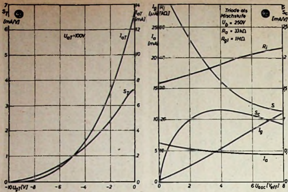
Abb. 4b u. c. ECH 81, UCH 81. Triodenkennlinien: b) Anodenstrom und Steilheit in Abhängigkeit von der Gittervorspannung; c) Kennlinien der Triode als Mischstufe
