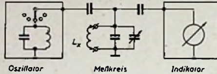
Abb. 1. Das Prinzip der L-Meßschaltung
