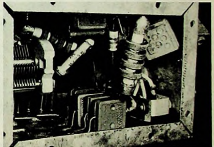
Abb. 11. Verdrahtungsansicht von rechts
