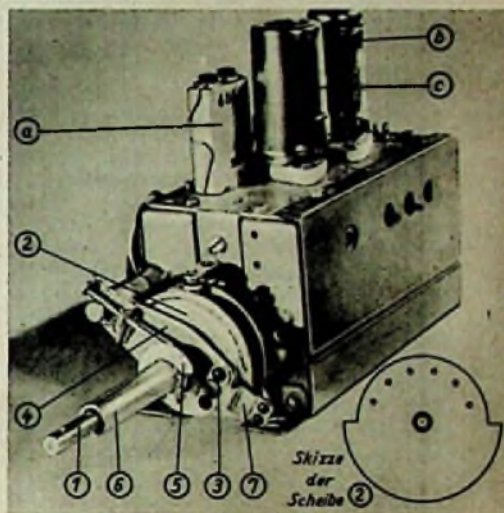
Abb. 3 (links). Schaltung des Kanalwählers. Abb. 4 (oben). Feinabstimmung; (a) 1. ZF-Filter (Bild-ZF 21,5 MHz, Ton-ZF 18 MHz), (b) EF 80, (c) ECC 81 (unter Abschirmung)
