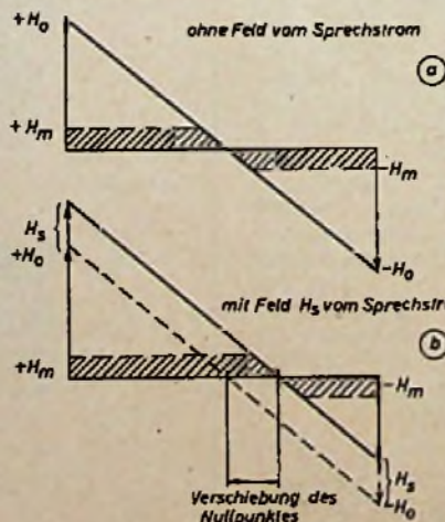
Abb. 3. Die Arbeitsweise des Schreibkopfes für die Aufnahme von Zackschrift
