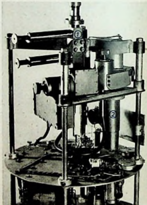
Abb. 4. Empfänger mit Eingangskreis; 1. Oszillator, Mischdiode und 1. ZF-Verstärker; ② 1/4 Transformator mit Sticheleitungen, ① Oszillator
