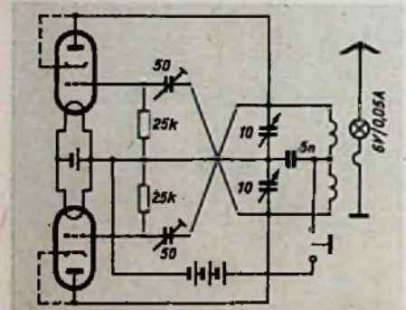
Abb. 1. Selbstregierter Gegentaktsender für Röhren 3 A 5, 2 x DL 94 usw. Abstimmspule 2 x 4 Wdg., 2,0 Cu, 25 mm \Phi , 20 mm lang; Antennenspule 2 Wdg. dazwischen
