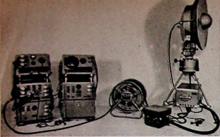
Senderseile der Fernseh-Dezi-Übertragungsanlage „T 44/2“ der Deutschen Werke Kiel. V. l. n. r.: Bedienungsgerät mit Netzgeräten; Kontrollgerät; Kabeltrommel; Gebläse; Parabolspiegel, darunter Dezi-Sender
