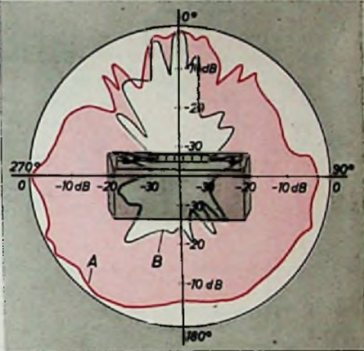
Rechts: Der Vergleich der Abstrahlungskurven eines Rundfunkempfängers mit Lautsprechern nach vorn (Kurve B) und der neuen Blaupunkt-Empfänger nach dem „3-D-Ton Raumlautsystem“ mit zusätzlichen seitlichen Hochtonlautsprechern (Kurve A) zeigt deutlich die gewünschte ungerichtete Abstrahlung hoher Frequenzen (8000 Hz)
