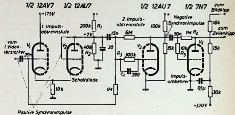
Abb. 1. Störspannungsbegrenzer von Philco mit Schaltdiode V_2
