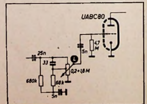
Lautstärkeregelung in der „Philatta“ (BD 234 U-L)
