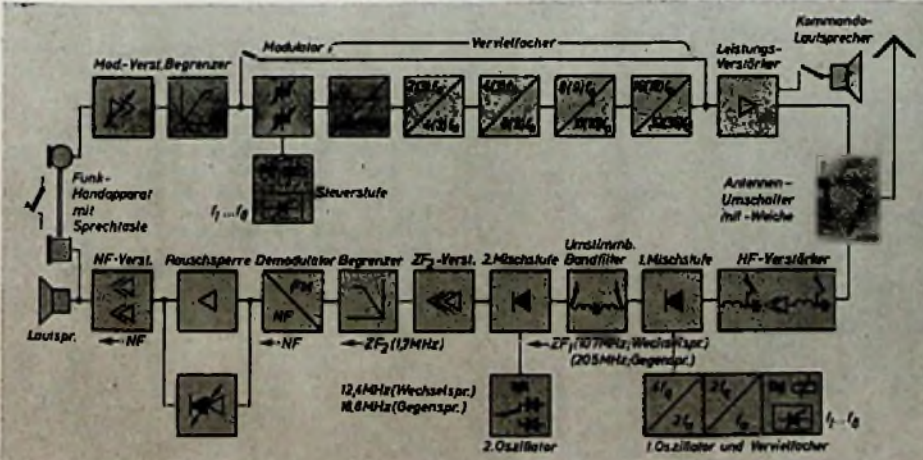
Übersichtsschaltbild der UKW-Funkfernprechanlage „ Funk 516 Y 333 “ (Siemens & Halske AG.)
