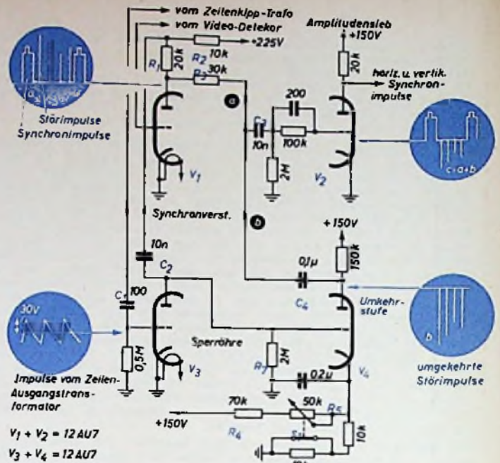
Abb. 4. Schaltung zur Kompensation der Störimpulse in der Synchronspannung im Emerson-Fernsehempfänger „120 174 B“ durch Vorzeichenumkehr
