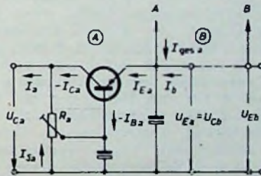
Bild 26. Prinzipschaltung eines Siebgliebes
