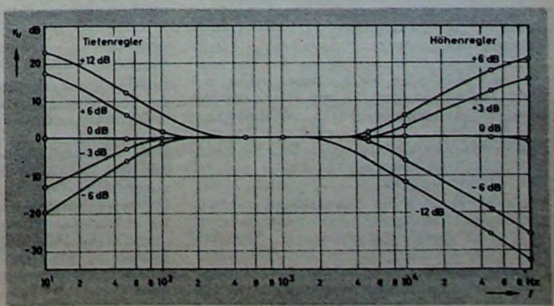
Bild 25. Frequenzgänge für verschiedene Stellungen des Klangreglers
