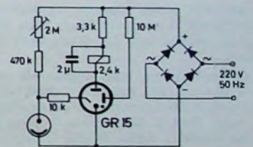
Bild 2. Dunkelschaltung mit Relaisröhre
