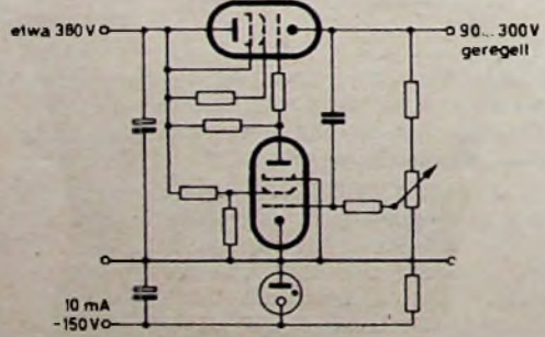
Bild 2 (oben). Elektronisch geregeltes Netzgerät mit getrenntem Gleichrichter für den Stabi
