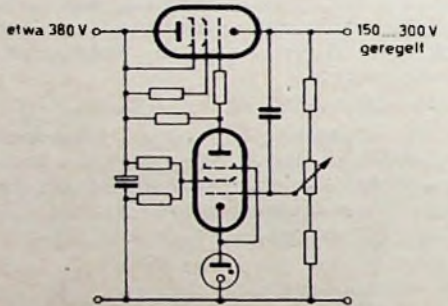
Bild 1. Übliche Schaltung eines elektronisch geregelten Netzgerätes
