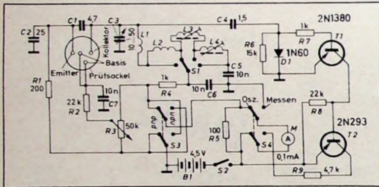
Bild 1. Vollständige Schaltung mit Daten eines einfachen Prüfgerätes zur Bestimmung der oberen Grenzfrequenz von Transistoren. L 1 = 1 Wdg., Draht Nr. 14 (1,63 mm \varnothing ) verzinkt, \frac{3}{8} " Windungsdurchmesser (9,5 mm), \frac{3}{8} " (19 mm) Zuleitungen; L 2 = 5 Wdg., Draht Nr. 18 (1 mm \varnothing ) verzinkt, \frac{3}{8} " (15,8 mm) Windungsdurchmesser, Abstand gleich Drahdurchmesser; L 3 = 9 Wdg., Draht Nr. 22 (0,64 mm \varnothing ) lackiert, \frac{3}{8} " Windungsdurchmesser (9,5 mm), enggewickelt auf Spulenkörper mit HF-Kern; L 4 = 25 Wdg., Draht Nr. 28 (0,32 mm \varnothing ) lackiert, \frac{3}{8} " Windungsdurchmesser (9,5 mm), enggewickelt auf Spulenkörper mit HF-Kern
