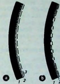
Bild 13. Ladungsverteilung und Deformation der Ölschicht für großen und kleinen Elektronenfleck. a) Fleckdurchmesser entspricht dem Zeilenabstand (glatte Oberfläche), b) Fleckdurchmesser kleiner als Zeilenabstand (zeilenförmige Deformationen der Oberfläche); 1 Hohlspiegel, 2 Ölschicht, 3 Ladungsverteilung
