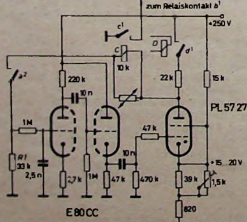
Bild 5. Steuer- und Regelkreis
