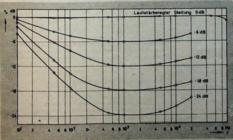
Bild 24. Frequenzgänge für verschiedene Stellungen des Lautstärkereglers
