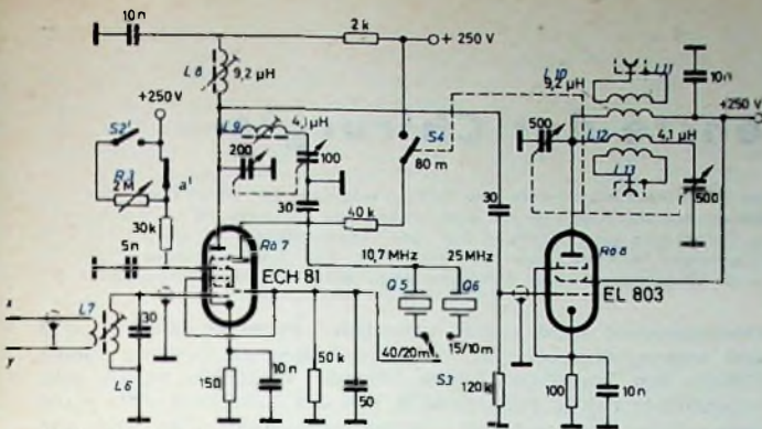
Bild 2. Schaltung Bandmischer, Endstufe und Netzteil
