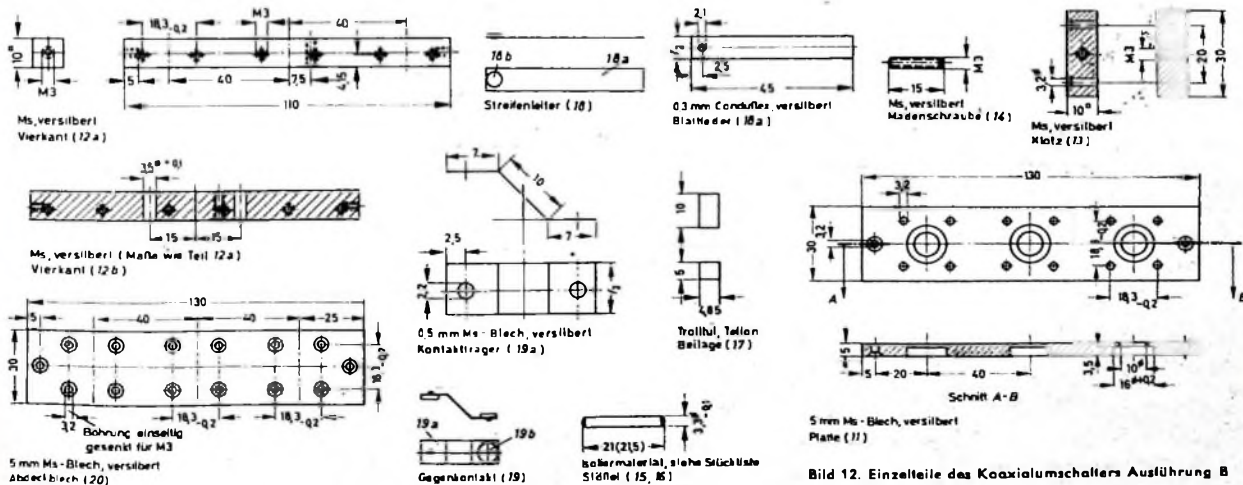
Bild 12 Einzelteile des Koaxialumschalters Ausführung B
