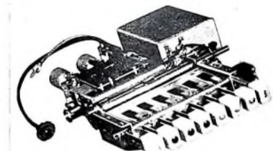
Bild 13. Programm- und Stations-Schnellwahlaggregat für je drei VHF- und UHF-Sender der Nordmende-Fernsehgeräte „Diplomat“ und „Kommodore“
