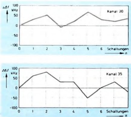
Bild 16. Wiederkehrgenauigkeit der 40fach-UHF-Memomatic, oben: Kanal 20; unten: Kanal 35
