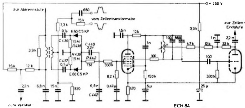
Bild 22. Schaltung der Zeilenausomatik in den Telefunken-Fernsehgeräten
