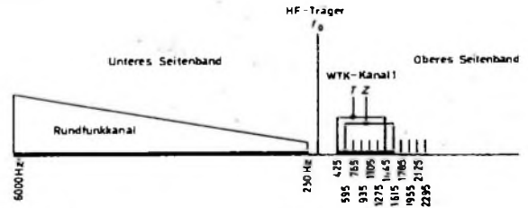
Bild 4. Modulationsschema für den Einseitenbandsender in Santiago
