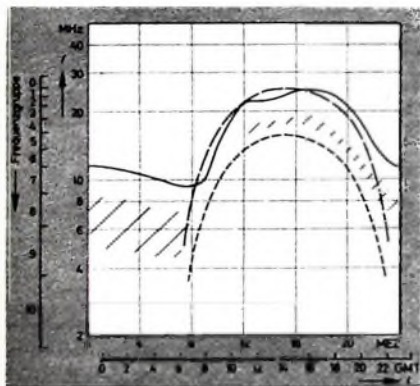
Bild 1 Funkprognose für den Monat März 1962 für die Verbindung mit Santiago. Die Prognosen gelten gleichmäßig in beiden Richtungen. (—) Median-MUF; (---) Median-LUF für P_{\text{eff}} = 100 \text{ kW} ; (- · - · -) Median-LUF für P_{\text{eff}} = 100 \text{ W} ; (.....) Median-FOT; (////) Median-FOT mittl. Sonnenfleckenrelativzahl A = 33
