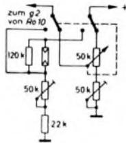
Bild 17. Schaltung der Kontrastautomatik von Philips
