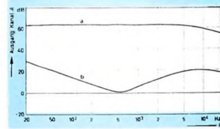
Bild 4. Frequenzgang (a) und Verlauf der Übersprechdämpfung (b) in Stellung „Mikrofon“ (Eingangsspannung 4 mV \pm 0 dB, Brummabstand 68,3 dB)
