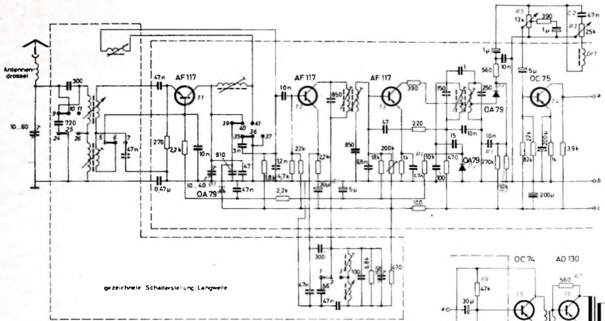
Bild 2. Schaltung des Autoempfängers „Hamburg ATR“ mit Eintakt-A-Endstufe (Blaupunkt)
