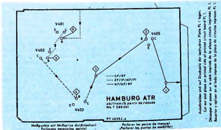
Bild 4: Messschablone für den „Hamburg ATR“
