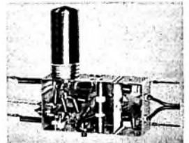
Wobbeloszillator (Innenansicht)
