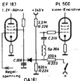
Bild 23. Prinzipschaltung der automatischen Rauschunterdrückung im „FE 252“ (Telefunken)
