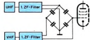
Bild 3. Kapselung der Mischbrücke für die VHF- und UHF-ZF-Einspeisung in den ZF-Verstärker
