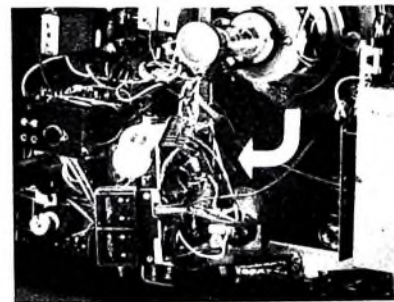
Bild 14. Für Servicezwecke lassen sich die Baugruppen der Nordmende-Fernsehchassis in betriebsfähigem Zustand abklappen oder herauschwenken
