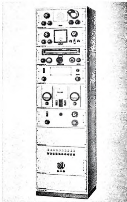
Bild 2 Einseitenbandempfänger für den kommerziellen Übersee-Telefonieverkehr (Siemens & Halske)
