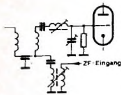
Bild 5. Einspeisung der UHF-Zwischenfrequenz in die VHF-Mischröhre
