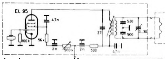
Bild 11. Schaltung des Wobbeloszillators zur Beseitigung der Zeilenstruktur (Metz)
