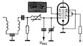
Bild 5. Einspeisung der UHF-Zwischenfrequenz in die VHF-Mischröhre
