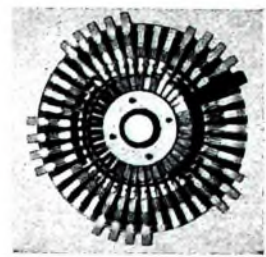
Bild 19. Schaltkranz des UHF-Tabulators (Philips)
