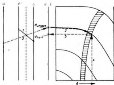
Bild 4. Zur Berechnung von d und I mit dem Nomogramm nach Bild 3. Bekannte Werte von F (Wickelraum) und S (mittlerer Umlang einer Windung) durch Linie 1 verbinden; Schnittpunkt (Zapfenpunkt) auf der gestrichelten Mittellinie mit bekanntem Wert auf der U -Leiter durch Linie 2 verbinden, Verlängerung von 2 schneidet 4. Leiter mit gesuchten Werten von d und I , die jedoch nur für blanken Draht gelten ( d_{\text{unkorr}} beziehungsweise I_{\text{unkorr}} ). Die Isolationsdicke \delta des Drahtes läßt sich unter Zuhilfenahme des rechten Teils des Nomogramms berücksichtigen (Schritte 3, 4 und 5 oder 3 und 5), so daß sich schließlich die korrigierten Werte d_{\text{korr}} beziehungsweise I_{\text{korr}} ergeben.
