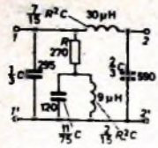
Bild 60. Schaltung und Dimensionierung eines Dietsold-Netzwerkes für die Bandbegrenzung der Farbdifferenzsignale
