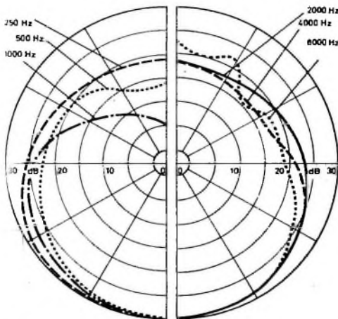
Dynamisches Mikrofon „D 9 D“ (AKG)
