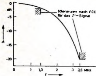
Bild 61. Amplitudenfrequenzgang des Dietsold-Netzwerkes nach Bild 60 im Toleranzschema für das I'-Signal
