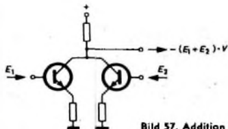
Bild 57. Addition mit Hilfe von aktiven Bauelementen
