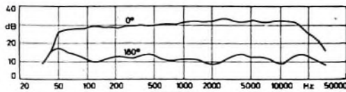
Dynamisches Bändchenmikrofon „MD 420“ (Mikrofonbau-Vertrieb) und Frequenzkurven des Mikrofrons
