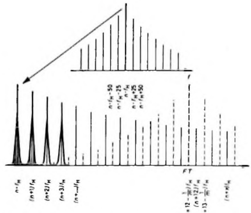
Bild 55. Spektralverklemmung: Frequenzspektrum des Leuchtdichtesignals E_Y' mit eingeschaltetem Farbtträger FT ( f_H in Hz, f_H = 15,625 kHz, n = 1, 2, \dots, m = 2, 3, \dots )
