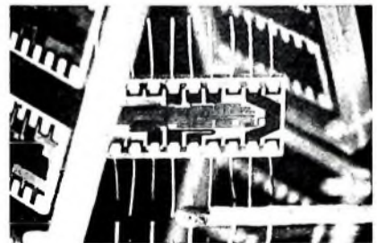
Bild 5. AC-Netzwerk für PCM-System von Siemens in Tantal-Dünnschichttechnik
