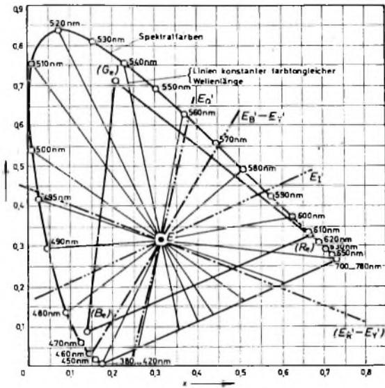
Bild 56. Lage der Farbdifferenzsignale im Farbdreieck ( y = 1 )
