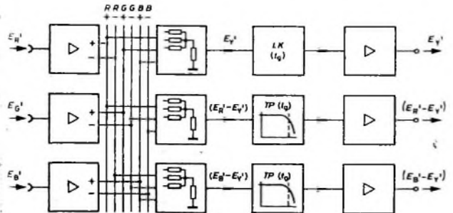
Bild 65. Codierung der Farbwertsignale und Blockschaltbild für einen PAL-Coder
