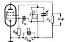
Bild 18 ECO-Schaltung (elektronengekoppelter Oszillator)
