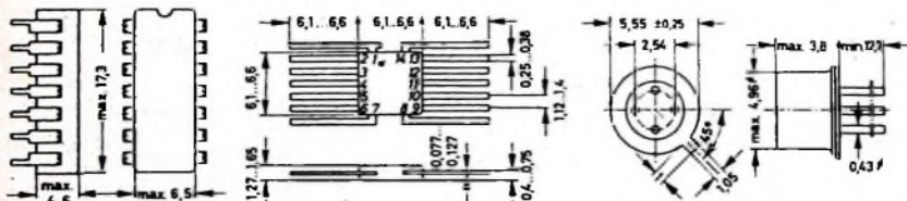
Bild 1. Verschiedene Gehäuseformen für integrierte Schaltkreise; a) D-1-Gehäuse, b) „flat-pack“, c) TO-5-Gehäuse
