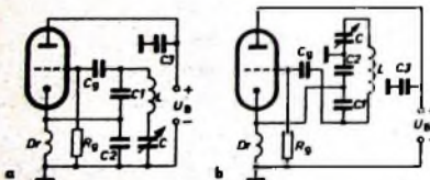
Bild 15. Der Clapp-Oszillator: a) übliche Darstellungswiese; b) Umkehrung von a) zur Erläuterung der kapazitiven Spannungsteilung
