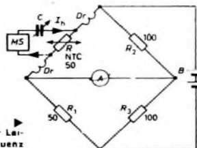
Bild 59. Schaltung eines Röhrenwattmeters
