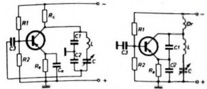
Bild 16 (links) Clapp-Oszillator mit Transistor in Emitterschaltung; Bild 17 (rechts) Clapp-Oszillator mit Transistor in Basisschaltung
