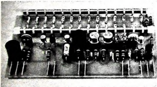
Bild 64. Praktische Ausführung einer LC-Laufzeitkette im Leuchtdichtekanal eines Coders
