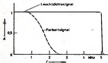
Bild 54. Verhältnis der Bandbreiten von Leuchtdichte- und Farbartsignal
