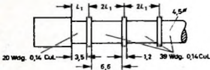
Bild 63. Dimensionierungsbeispiel für den induktiven Teil einer Laufzeitkette mit m-Gliedern ( L = 3,55 \mu\text{H} , m = 1,27 )
