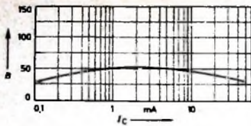
Bild 10. Stromverstärkung \beta des BFY 90 von Valvo in Abhängigkeit vom Kollektorstrom I_c
