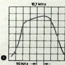
Bild 6. ZF-Durchlaßkurve eines herkömmlichen Transistor-Empfängers bei kleinem Eingangssignal (a) und bei großem Eingangssignal (b)
