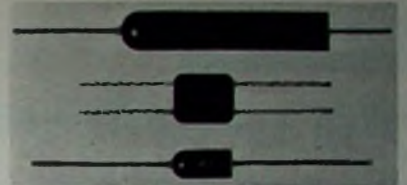
Valvo-Gleichrichter-Dioda BY 140, Brückenschaltung BY 123 und Gleichrichterzelle BY 138 mit kontrollier-tem Durchbruchverhalten
