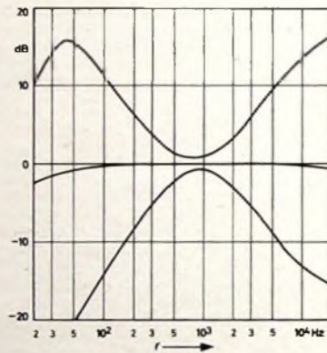
Bild 3. Einstellbare Frequenzgänge des Verstärkers
