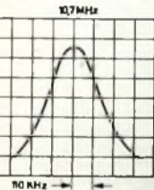
Bild 6. ZF-Durchlaßkurve eines herkömmlichen Transistor-Empfängers bei kleinem Eingangssignal (a) und bei großem Eingangssignal (b)
