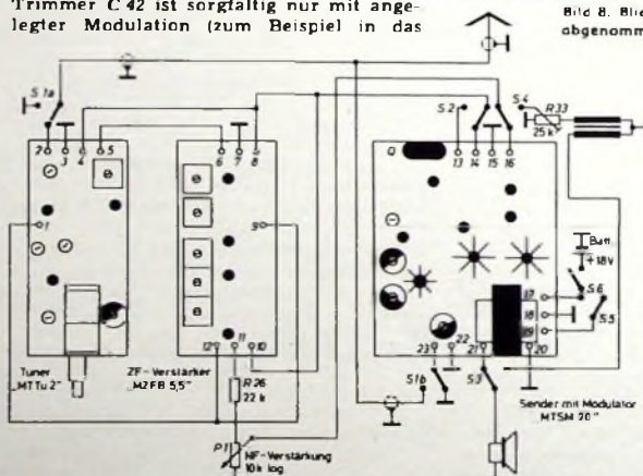
Bild 9. Verdrahtungsplan der einzelnen Bausteine
