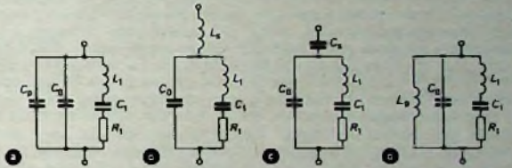
Bild 14. Nachträgliches Verändern der Schwingfrequenz des Quarzes („Ziehen“ der Frequenz) durch eine Parallelkapazität C_D (a), eine Serieninduktivität L_s (b), eine Serienkapazität C_s (c) und durch eine Parallelinduktivität L_p (d)
