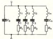
Bild 11. Ersatzschaltbild eines Quarzes mit Nebenresonanzen
