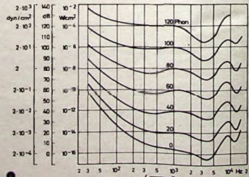
Bild 4. Kurven gleicher Lautstärke nach Fletcher und Munson (a) und Kurven gleicher Lautstärke nach ISO-Empfehlung
