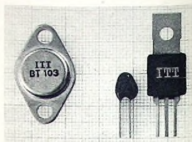
Thyristoren von Intermetall in Plastik- und Metallgehäusen
