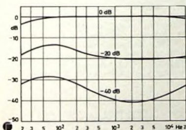
Bild 6 Mit einmal angezapftem Lautstärkesteller erreichte Kurven (a) und mit dreimal angezapftem Lautstärkesteller erreichte Kurven (b); für die gestrichelten Kurven gelten die im Bild 2 eingeklammerten Werte der Beschaltungswiderstände und -kondensatoren
