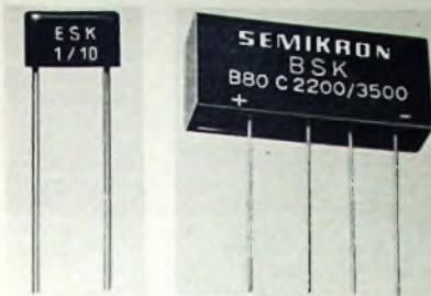
Gleichrichter der Reihe ESK 1 (links) und Gleichrichter der Reihe BSK von Semikron
