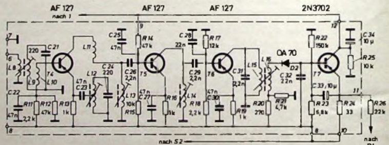
Bild 3. Schaltung des ZF-Teils
