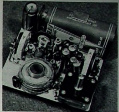
Bild 4. Blick auf den Transistor-Einkreiser
