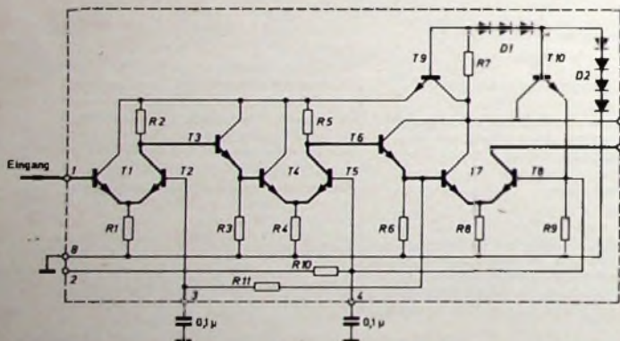
Bild 2. Schaltbild der Halbleiterschaltkreise CA 3011 und CA 3012
