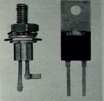
Valvo-Thyristoren im Plastik- und Metallgehäuse BT 100/500 (rechts) und BT 101/500 (links)
