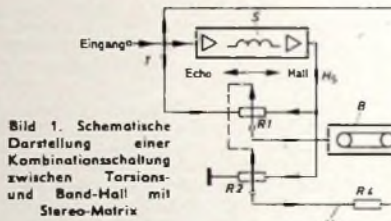
Bild 1. Schematische Darstellung einer Kombinationschaltung zwischen Torsions- und Band-Hall mit Stereo-Matrix
