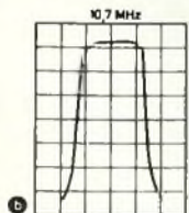
Bild 5. ZF-Durchlaßkurve des „AR-15“ mit kleinem Eingangssignal (a) und mit großem Eingangssignal (b)
