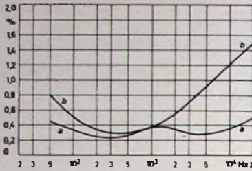
Bild 8 Klirrfaktor des Verstärkers; Frequenzgang linear (a), Höhen und Tiefen angehoben (b)
