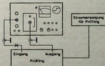
Bild 6. Meßschaltung für Rauschmessungen an einem Fernseh-Tuner; an der Stelle x ist bei Bedarf ein Symmetrierglied einzulügen
