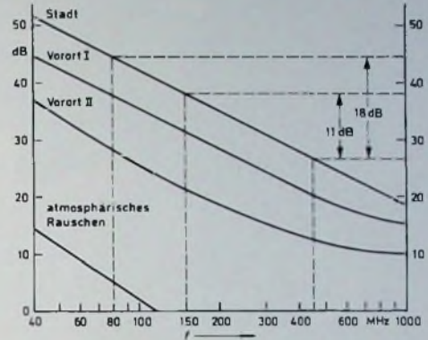
Bild 5. Störpegelspektrum bei verschiedenen Sprechfunkfrequenzen
