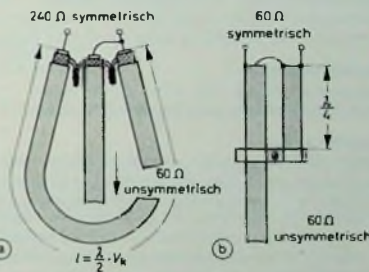
Bild 2. a) \lambda/2 -Umwegleitung zur Symmetrierung und Impedanztransformation. b) Symmetrieranordnung ohne Impedanztransformation
