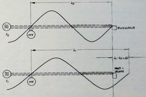
Bild 1. Meßaufbau
