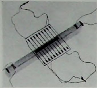
Bild 8. Akustischer Verstärker mit unterteilter Beschleunigungszone [10]
