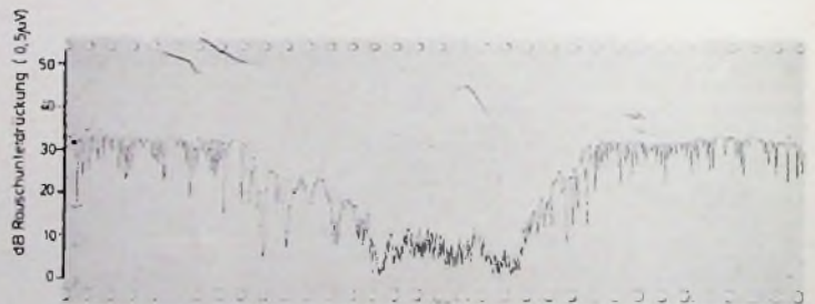
Bild 2a VHF-Feldstärkediagramm, gemessen mit einem Fahrzeugfunksprengerät, KF 160 00 , Frequenz 147,83 MHz, 5/8-λ-Antenne; die Feldstärke sinkt in Tunnelmitte bis auf 0 dB ab
