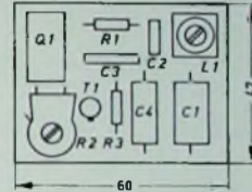
Bild 3. Anordnung der Bauteile auf der Resopalplatte
