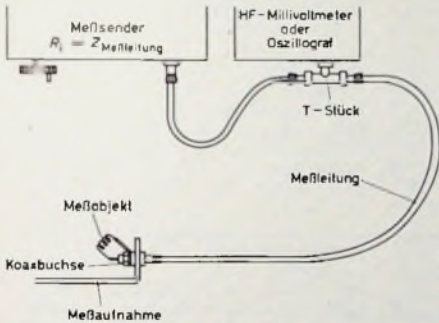
Bild 1. Meßaufbau
