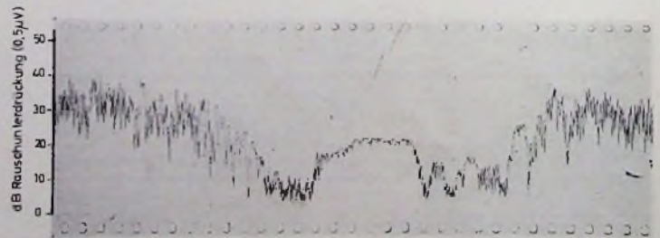
Bild 2b UHF-Feldstärkediagramm, gemessen mit einem Fahrzeugfunksprengerät, KF 450 00 , Frequenz 459,55 MHz, \lambda/4 -Antenne; die Feldstärke steigt in Tunnelmitte an, Sprechverbindung ist ab 5 dB Rauschunterdrückung möglich
