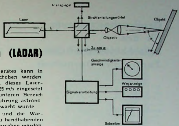
Bild 1. Prinzip des Laser-Dopplersystems (LADAR)
