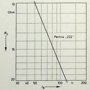
Bild 3. Zusammenhang zwischen der Lebensdauer t_B (Mittelwert) von Trockenbatterien (bei täglich vierstündigem Betrieb sowie einem Absinken der Zellenspannung bis auf 0,75 V) und dem Belastungswiderstand R_Z je Zelle
