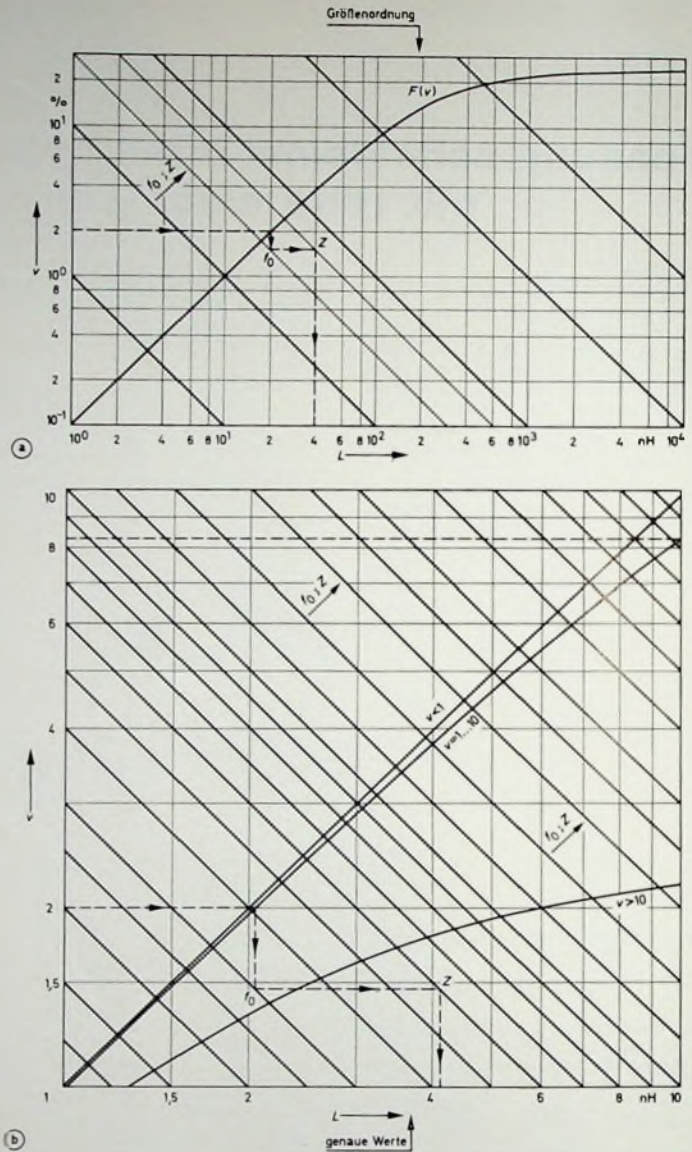
Bild 3 Zusammenhang zwischen Verstimmung v , Kurzschluß- Resonanzfrequenz f_0 , Wellenwiderstand Z und Abschlußreaktanz L
