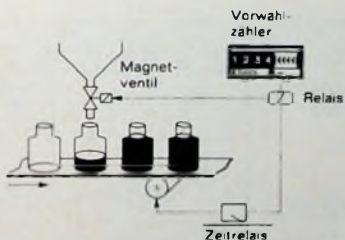
Bild 69 Flüssigkeitsdosierung mit Hilfe eines Vorwahlzählers (Elesta)
