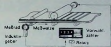
Bild 70 Steuerung einer Abschneidemaschine mit einem Vorwahlzähler (Elesta)
