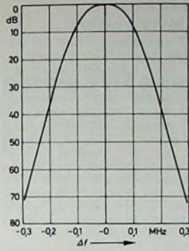
Bild 4 (oben) FM-ZF-Durchlaßkurve
