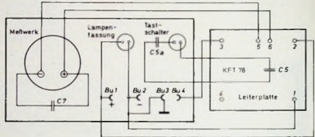
Bild 8 Verdrahtungsplan der Frontplatte (von hinten gesehen) mit der bestückten Leiterplatte
