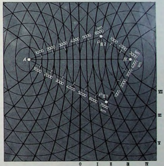
Bild 1. Grundprinzip der Hyperbelnavigation
