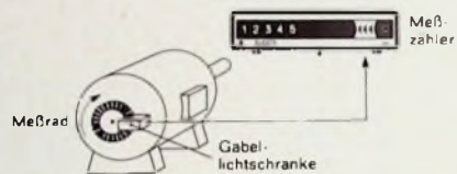
Bild 73 Schlupfmessung an einem Asynchronmotor mit Hilfe eines Meßzählers (Elasta)
