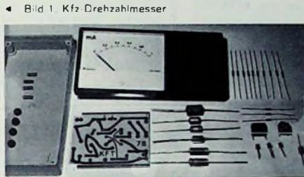
Bild 1: Kfz-Drehzahlmesser
