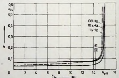
Bild 12. Klirrfaktor k in Abhängigkeit von der Ausgangsspannung U_a
