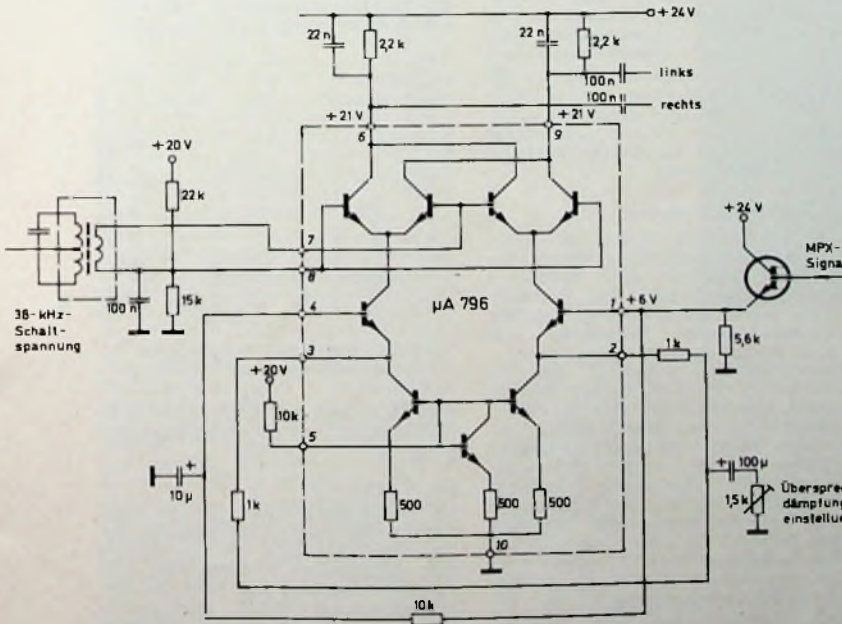
Bild 8. Symmetrischer Schaldemodulator des Multiplex-Decoders
