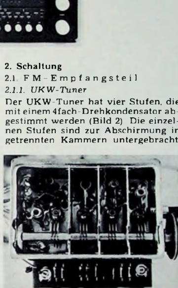
Bild 2 Innenansicht des UKW-Tuners
