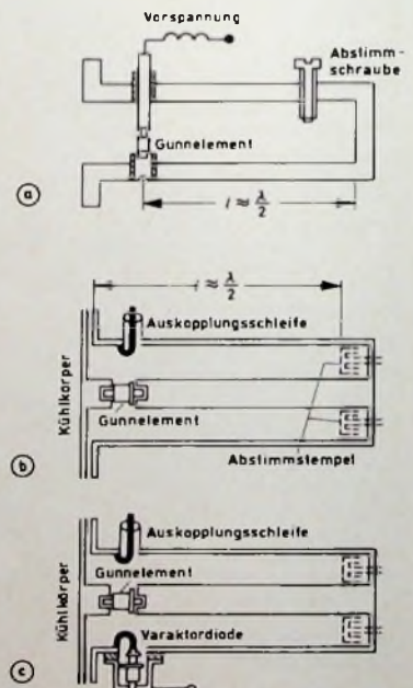
Bild 4. Typische Einbaumöglichkeiten eines Gunnoszillators in: a) Rechteck-Hohlleiterresonator, b) Koaxialresonator abstimmbare, c) Koaxialresonator mit Varaktordiode abstimmbare
