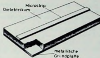
Bild 7. Flachleiter-Microstrip
