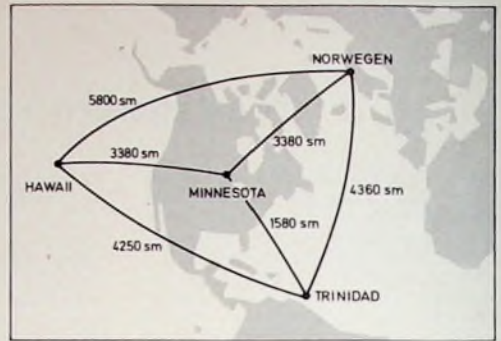
Bild 2. Bedeckung der vier gegenwärtig im Betrieb befindlichen Versuchsstationen des „Omega“-Systems [3]
