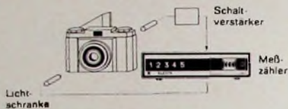
Bild 72 Messen der Verschlusszeiten eines Fotoapparates mit Hilfe eines Meßzählers (Elasta)
