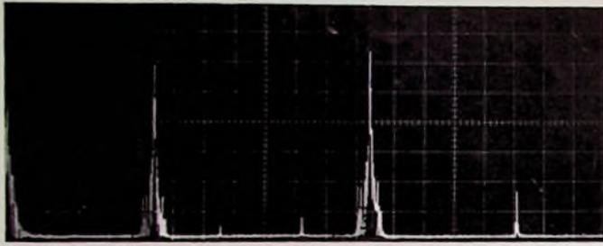
Bild 3 Spektren von Hochtonlautsprechern. Oben: hochwertiger Hornlautsprecher; die Seitenbänder liegen 50 und 45 dB unter dem Wert von f_2 . Unten: Ionen-Lautsprecher; die Seitenbänder liegen 10 und 25 dB unter dem Wert von f_2 ( f_1 = 5 kHz, f_2 = 125 kHz, jeweils 0,5 V. Vertikalachse 10 dB/Rastertig. ◀ Horizontalachse etwa 1 kHz/Rastertig)
