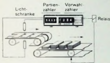
Bild 68 Steuerung des Stapelns von Papierbögen oder Zeitungen durch einen Vorwahlzähler und Zählen der Stapel durch einen Partienzähler (Elesta)
