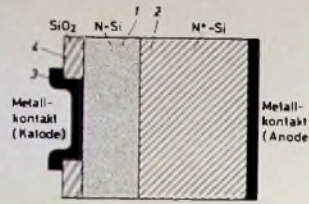
Bild 9 (oben) Aufbau einer Epitaxial-Planar-Schottky-Diode für das X-Band (AEG-Telefunken)
