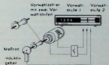
Bild 71 Steuerung einer Wickelmaschine mit einem Vorwahlzähler mit zwei Vorwahlstufen (Elesta)
