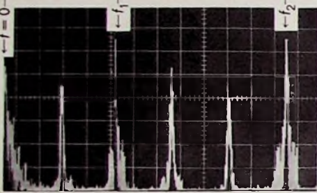
Bild 3 Spektren von Hochtonlautsprechern. Oben: hochwertiger Hornlautsprecher; die Seitenbänder liegen 50 und 45 dB unter dem Wert von f_2 . Unten: Ionen-Lautsprecher; die Seitenbänder liegen 10 und 25 dB unter dem Wert von f_2 ( f_1 = 5 kHz, f_2 = 125 kHz, jeweils 0,5 V. Vertikalachse 10 dB/Rastertig. ◀ Horizontalachse etwa 1 kHz/Rastertig)
