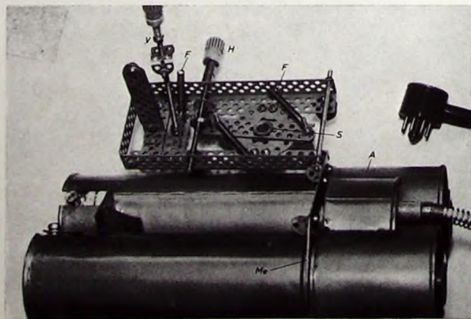
Bild 4. Blick in den hochgeklappten Grundrahmen (V, H Gewindespindel für vertikale und horizontale Verstellung; F Vorspannfedern; S Stativgewinde; Me Messinggrundplatte; A Abdeckhaube)
