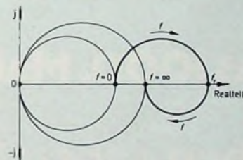
Bild 3 Allgemeine Ortskurve des Gesamtstromes für die Schaltungen nach Bild 2 und 8 bei R_1 \neq R_2
