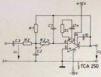
Bild 7 Aktiver Tiefpaß zweiter Ordnung mit dem integrierten Zweifach-Filterverstärker TCA 250
