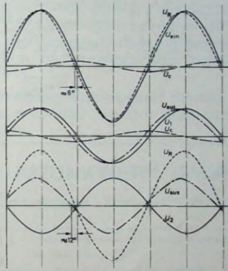
Bild 15. a) Vektordarstellung für R_3 \gg X_c , b) Verlauf der Spannungen ( U_{ein} = 10 \text{ V} , R_3 \approx 100 \text{ k}\Omega , X_c \approx 10 \text{ k}\Omega , \varphi \approx 5,7^\circ , U_a = U_{ein} \cdot \sin \varphi = 0,987 \text{ V} , U_c = U_{ein} \cdot \cos \varphi = 9,95 \text{ V} )
