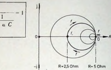
Bild 9. Ortskurve des komplexen Gesamt widerstandes der Schaltung nach Bild 8 bei R_1 = R_2 = 5 \text{ Ohm} , L_1 = L_2 = 0,8 \text{ mH} und C_1 = C_2 = 32 \mu\text{F}
