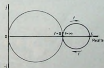
Bild 4 Allgemeine Ortskurve des Gesamtstromes für die Schaltungen nach Bild 2 und 8 bei R_1 = R_2
