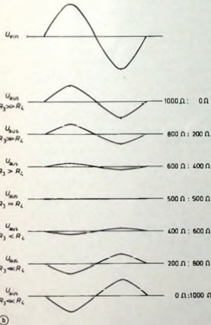
Bild 5 Veränderbare Brücke: a) (oben): Schaltung, b) (links): Verlauf der Ausgangsspannung bei verschiedenen Verhältnissen R_3 : R_4
