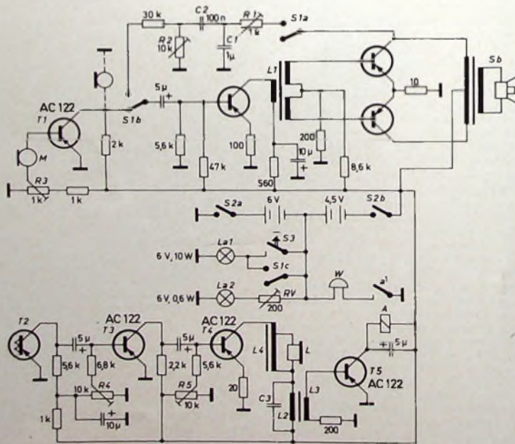
Bild 2 Schaltung des Lichtsprechgerätes ( L 2 : 1000 Wdg, 0,1 mm CuL, L 3 : 250 Wdg, 0,1 mm CuL, Kern M 30; L 4 : Übertrager 2:1, beispielsweise Gegenakt-Treiberübertrager, Relais A: Kammrelais 12 V, 20 mA)
