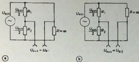
Bild 3 Extrem unabgeglichene Brücke: a) \varphi_{aus} = 0^\circ . b) \varphi_{aus} = 180^\circ
