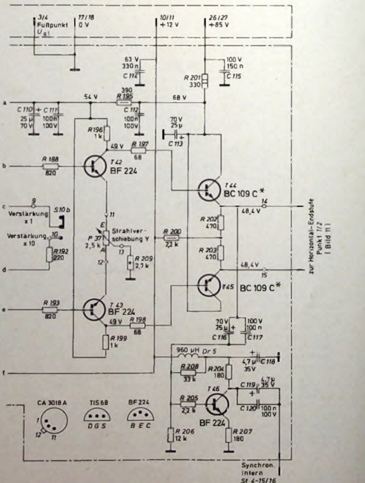
Bild 10 (oben und rechts). Schaltung des Vertikalverstärkers
