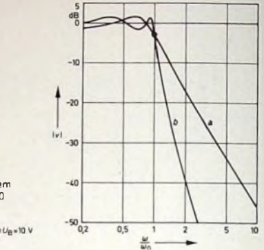
Bild 8 (oben) Tschebyscheff Tiefpaßcharakteristiken zweiter Ordnung (Kurve a) und vierter Ordnung (Kurve b) zur Sinusbildung aus Rechteckspannungen
