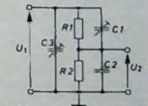
Bild 9b. Prinzip des frequenzkompensierten Abschwächers
