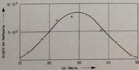
Bild 9. PDME: Ver- teilung der 1 \sigma -Werte (Gesamtzahl der Meß- werte: 37 679)
