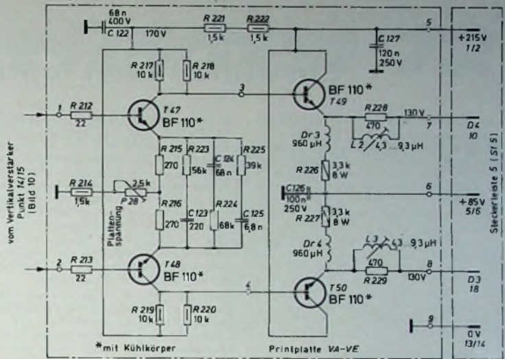
Bild 11 Schaltung der Vertikal-Endstufe
