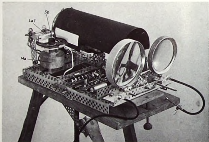
Bild 3. Modulationssystem im Versuchsaufbau (Sb Schwingblende, La 1 Lampe, Ma Metallklötzchen)
