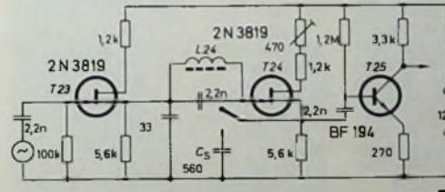
Bild 11. Schaltung zur Entdämpfungsmessung an der Schwingkreisanzordnung nach Bild 10
