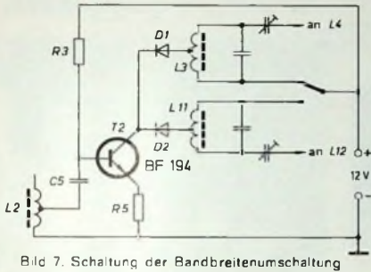
Bild 7. Schaltung der Bandbreitenumschaltung
