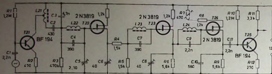
Bild 13. Einseitenbandfilter für 450...455 kHz mit drei entdämpften Kreisen.
