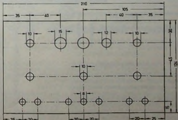
Bild 7. Bohrplan für die Frontplatte ▶
