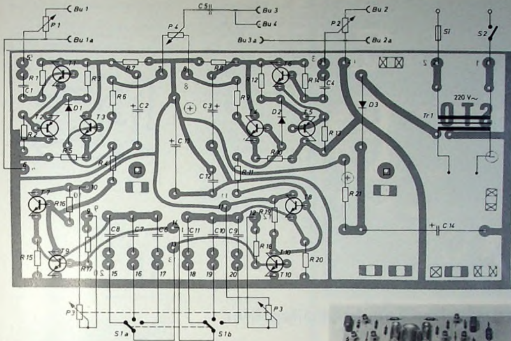
Bild 5 (oben). Bestückungs- und Verdrahtungsplan
