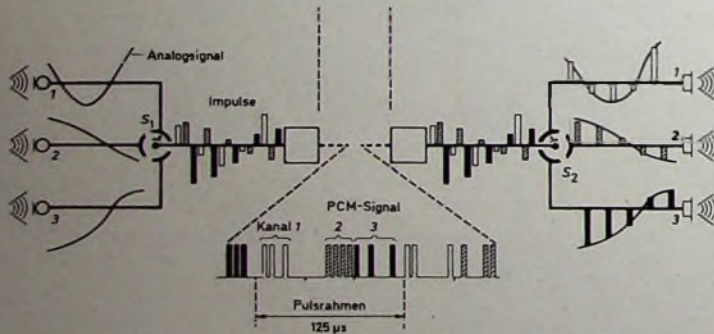
Bild 5 Prinzipschema eines PCM-Systems für drei Telefonkanäle (1, 2, 3) mit Zeitmultiplex-Bündelung. Die drei Signale werden mit Hilfe der synchron umlaufenden Schalter S_1 und S_2 nacheinander elektronisch abgetastet, quantisiert, codiert, gemischt, übertragen und auf der Empfangsseite wieder entsprechend aufgetrennt.
