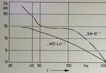
Bild 6. Relative Windgeräusch-Empfindlichkeit ohne Windschutzhauben, bezogen auf den gleichen Feldübertragungsfaktor bei 200 Hz
