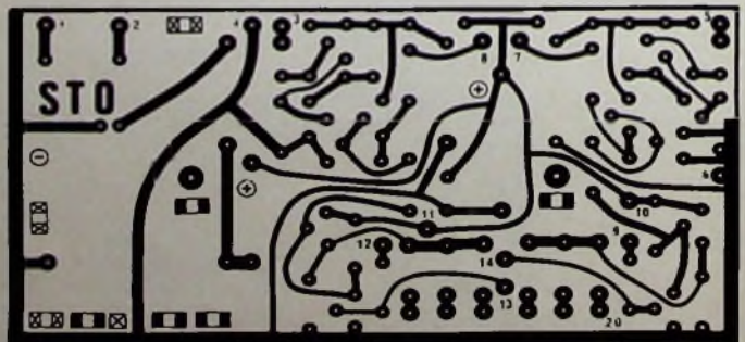
Bild 4. Printplatte des elektronischen Zweikanalschalters (Maßstab 1 : 2)
