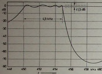
Bild 13. Einseitenbandfilter für 450...455 kHz mit drei entdämpften Kreisen.
