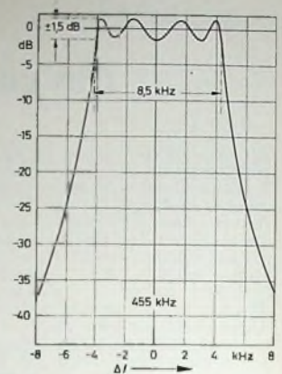
Bild 4 Durchlaßkurve der Filterschaltung nach Bild 3
