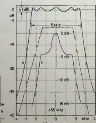
Bild 6 Gesamtdurchlaßkurve (a) des Filters nach Bild 5 sowie Durchlaßkurve (b) des dreikreisigen Koppelfilters L 11, L 12, L 13 der ersten Stufe
