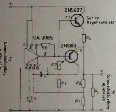
Bild 16 Spannungsregelachaltung mit Kurzschlußstrom-Rückregelung
