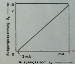
Bild 14 Ausgangskennlinie einer Spannungsregelschaltung nach Bild 15 mit Kurzschlußstrom-Rückregelung
