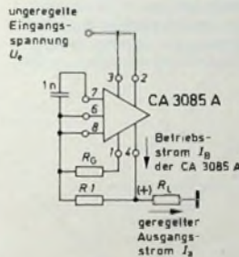
Bild 21. Stromreglerschaltung für Ströme bis zu 100 mA
