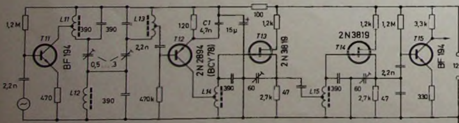
Bild 5 Fünfkreisbandfilter (455 ± 2,5 kHz) mit zwei frequenzversetzten und entdämpften Kreisen
