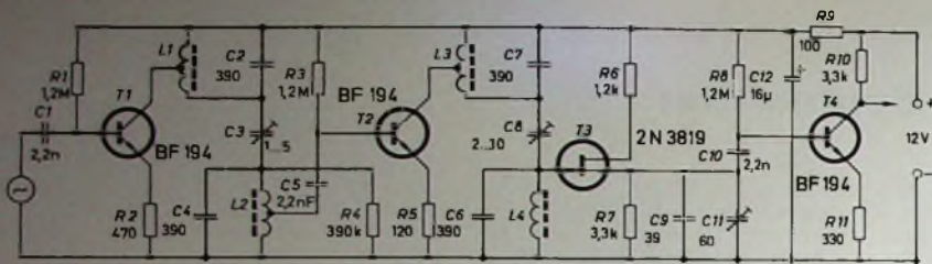
Bild 3 Vierkreisbandfilter (455 ± 4,25 kHz) mit Entdämpfung des zweiten Koppelkreises
