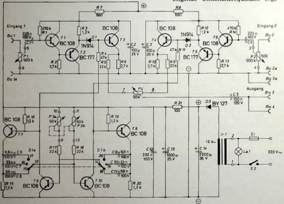
Bild 1 Elektronischer Zweikanalschalter
