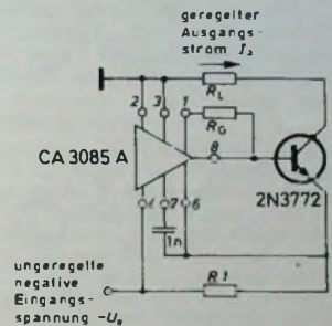
Bild 21. Stromreglerschaltung für Ströme bis zu 100 mA
