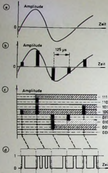
Bild 4 Prinzip der PCM: a) ursprüngliches analoges NF-Signal, b) mit 8 kHz Tastfrequenz abgetastetes Sprachsignal und Aufteilung in Impulse (Amplitudenproben), c) die Amplitude der Impulse wird gemessen (quantisiert), d) im Codierer werden die Amplituden in digitale Zeichen umgewandelt (je höher die Amplitude, um so mehr Zeichen)
