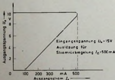
Bild 17. Ausgangskennlinie der Spannungsregelachaltung nach Bild 16 mit Kurzschlußstrom-Rückregelung
