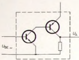
Bild 3 Nichtgegengekoppelter Verstärker ( U_{BE} = 1 \text{ mV} , U_A = 1 \text{ V} , Leerlaufverstärkung V_0 = 1000 )
