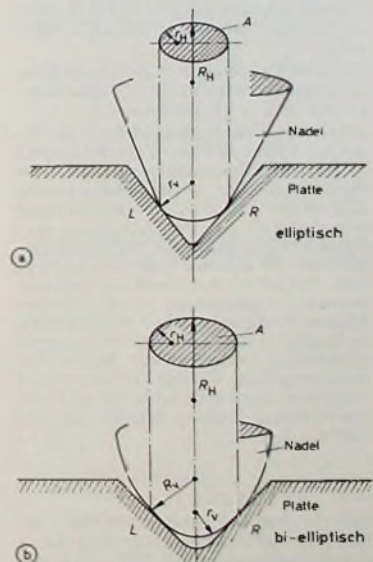
Bild 3 Vergleich der elliptisch (a) und bi-elliptisch (b) verrundeten Abtastnadelspitze ( R_H , r_H Radien des Nadelquerschnitts zwischen den Berührungspunkten; R_L , r_L Radien der Nadelprojektion im Rillenbereich)
