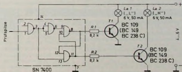
Bild 2. Schaltung des L-H-Anzeigers für Rechteck-Impuls-Folgefrequenzen bis zu 30\text{MHz}
