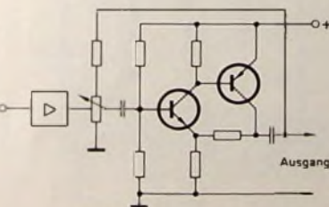
Bild 2. Verstärkerschaltung mit Signaleinspeisung
