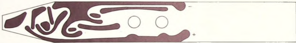
Bild 5. Printplatte des L-H-Anzeigers für die Schaltung nach Bild 2
