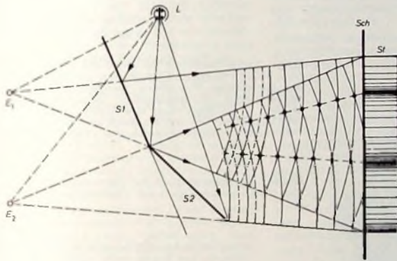
Bild 1. Entstehung von Interferenzstreifen (SI) auf einem Schirm (Sch) mit Hilfe zweier geneigter Spiegel (S1, S2) erzeugter (aber nicht vorhandener) „virtueller“ Lichtquellen ( E_1, E_2 ), die phasengleich schwingen (Prinzip des Fresnel'schen Spiegelversuchs)
