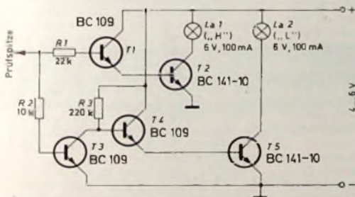
Bild 1. Schaltung des L-H-Anzeigers für Rechteck-Impuls-Folgefrequenzen bis zu 60\text{kHz}
