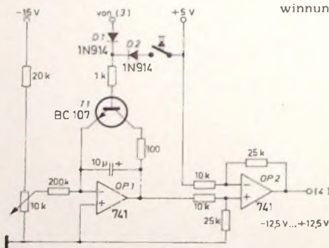
a) Sägezahn-generator
