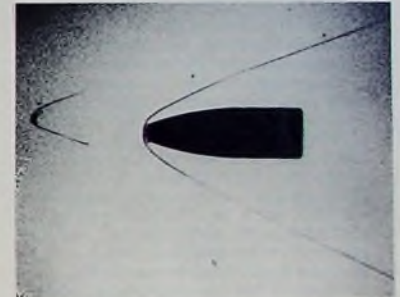
Bild 8. Beispiel eines Kurzeithologramms, das ein Geschöß – es fliegt mit einer Geschwindigkeit von 1 km/s – und eine Explosionswelle zeigt (aufgenommen mit Q-switch-Laser und Holokamera der TRW Inc.)
