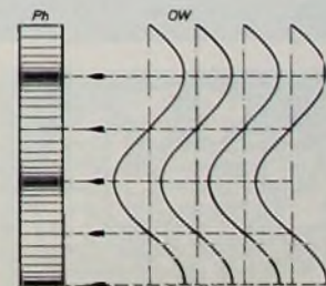
Bild 3. Reflektierte und entsprechend dem beleuchteten Gegenstand deformierte Objektwelle (OW) (zusammen mit der – hier nicht eingezeichneten – Referenzwelle gleicher Frequenz) ergeben auf der Fotoplatteinterferenzmuster, die – je nach Form des Gegenstandes – sehr komplexe Formen annehmen können
