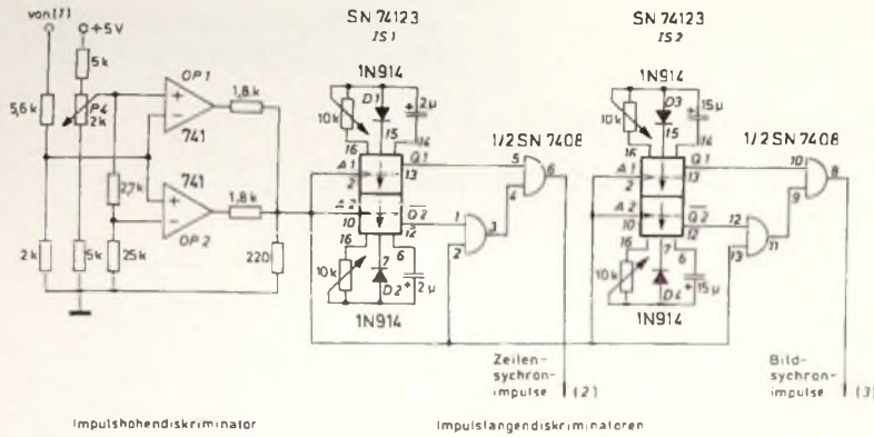
Bild 3 Schaltung der Synchronsignalgewinnung
