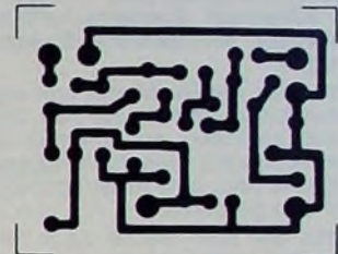
Bild 1. Schaltung des Mithörverstärker-Bausteins
