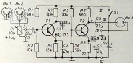
Bild 1. Schaltung des Mithörverstärker-Bausteins
