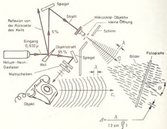
Bild 5 Versuchsaufbau eines 3-D-Bildes mit Gaslaser ( \lambda = Entfernung zweier Knotenstellen, \lambda = Wellenlänge des Laserlichtes, \theta = Winkel zwischen reflektiertem Objektstrahl C_1 und gespiegeltem Referenzstrahl C_2 ). Im Falle \lambda \sim \lambda ergibt sich eine Auflösung von etwa 2000 Zeilen/mm, die sich allerdings nur mit Fotoemulsionen sehr hoher Auflösung erreichen lässt
