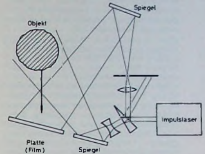
Bild 7. Prinzipanordnung zur Herstellung von Auflichthologrammen mit RiesenimpulsLasern [5]
