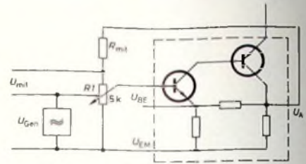
Bild 5 Verstärker mit Emitttergegenkopplung und Basismitkopplung ( U_{BE} = 1 \text{ mV} , U_{EM} = 99 \text{ mV} , U_{BM} = 100 \text{ mV} , U_A = 1 \text{ V} , U_{Gen} = 1 \text{ mV} , U_{R1} = 99 \text{ mV} , V = 1000 )
