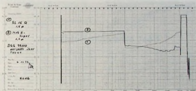
Bild 8. Übertragungsbereich und Frequenzgang: Kurve 2 Stereo-Abtaster „M15E-Super“ bei 1 p, Kurve 1 Quadro-Tonabnehmer „SL15Q“ bei 1,5 p, Stereo-Meßplatte nach DIN 45 541 (Lautwerk Dual „701“)
