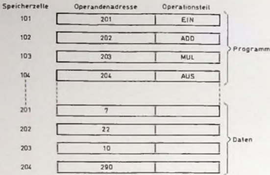
Bild 2. Programmbeispiel
