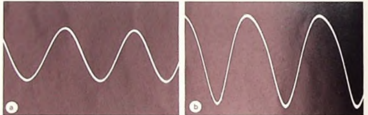
Bild 4. Oszillogramme der Ausgangsspannung des Quadro-Tonabnehmers „SL15Q“ mit „STM-72“ bei Überpegel (Abtasticherheit): a) 315-Hz Tiefenschrift 56 µm (+ 6 dB), b) 315-Hz-Seitenschrift 90 µm (+ 10 dB)
