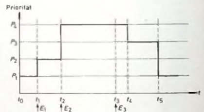
Bild 4. Beispiel für einen zeitlichen Ablauf bei prioritätsgesteuerten Programmabläufen
