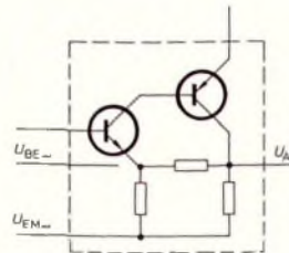
Bild 3 Nichtgegengekoppelter Verstärker ( U_{BE} = 1 \text{ mV} , U_A = 1 \text{ V} , Leerlaufverstärkung V_0 = 1000 )
