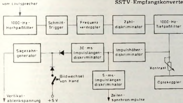
Bild 1: Blockschaltung des SSTV-Konverters
