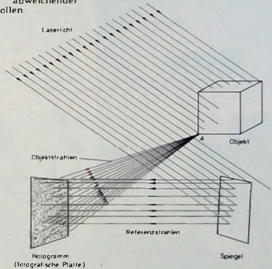
Bild 2. Aufnahme eines Hologramms mit Laserlicht und Spiegeloptik
