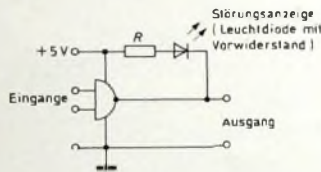
Bild 1. Leuchtdiode zur Überwachung eines TTL-Gatters. Die verfügbare Ausgangsverzweigung ist um einen gewissen Betrag herabgesetzt, der vom Leuchtdiodenstrom abhängt.
