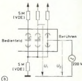
Bild 4 Einfügung von Schutzwiderständen nach VDE bei einem Gerätechassis, das auf Phasen-spannung liegt; a) Zustand beim Berühren einer Sensorelektrode, b) Zustand beim gleichzeitigen Berühren von Sensorelektrode und Sensorgegenelektrode
