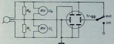
Bild 1. Vorschlag für den Meßgeräteaufbau zum Tonabnehmertest mit der TTR 102
