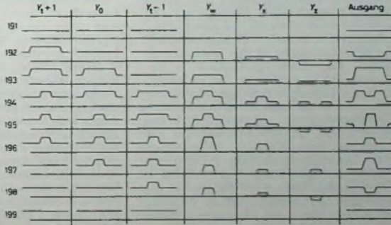
Bild 2 Wirkung des Konturverstärkungssignals bei Aufnahme nebeneinanderliegender horizontaler und vertikaler Rechtecke (oben)
