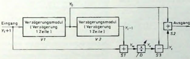
Bild 1 Blockschema für die senkrechte Konturverstärkung
