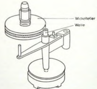
Bild 4. Antrieb des Wickeltellers durch eine auf der Achse des Permanentmagneten aufgesetzte Andruckrolle.
