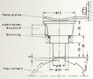
Bild 6 (unten) Einbauskitze des Abreißoszillatorgebers mit Impulsstern
