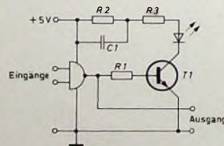
Bild 2. Ein zusätzlicher Transistor T_1 gestattet die Verwendung von Leuchtdioden mit höherem Stromverbrauch. Bei niedrigem Tastverhältnis der Impulsfolge sorgt der Kondensator C_1 für einen höheren mittleren Durchlaßstrom. R_2 begrenzt den Dauerstrom, wenn das Gatter bei hohem Ausgangspegel stehenbleibt.
