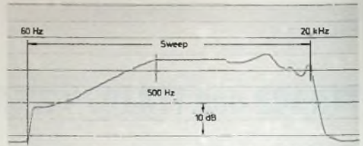
Bild 3. Schnelleproportionale Ausgangsspannung beim Abtasten des Sweep Teiles der TTR 102 in den Bändern 3 und 6
