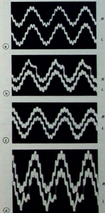
Bild 2. Tonabnehmertest mit Testplatte Shure TTR 102, Band 7 ... 13; a) Phasenlage und Übertragungsmaß stimmen, keine Verzerrungen, Auflagekraft nicht zu gering (1 D); b) wie a), jedoch mit auf 0,6 p verringerter Auflagekraft, Verzerrungseinsatz im rechten Kanal; c) wie b), jedoch mit optimaler Antiskating-Einstellung, dadurch Rillen-Nadel-Kontakt an rechter Rillenflanke verbessert; d) wie a), jedoch mit doppeltem Pegel und Antiskating-Überkompensation, dadurch Verzerrungen im linken Kanal
