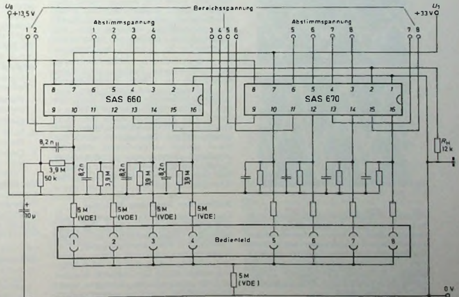
Bild 6. Zusätzliche externe Maßnahmen zur Sicherung der Bevorrechtigungsschaltung der ersten Stufe der SAS 660
