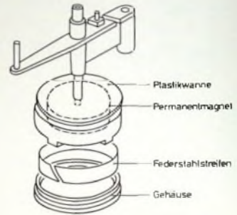
Bild 3. Prinzipielle Ausführung der Hysterese-Friction.
