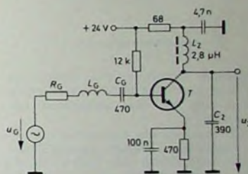
Bild 5. Schaltung eines Verstärkers
