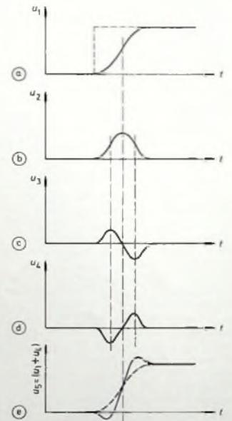
Bild 4 Wirkungsweise des Differenzentzerrers
