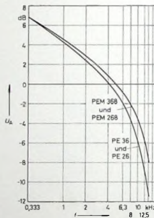
Bild 2 Aussteuerbarkeit der Professional-Tonbänder „PEM 368“ und „PEM 268“ sowie der Low-Noise-Bänder „PE 36“ und „PE 26“ ( v = 9,5 \text{ cm/s} , \tau = 90 \text{ µs} , 0 \text{ dB} = 250 \text{ nWb/m} , S_a = 7 \text{ m} , S_r = 3 \text{ m} , \Delta p = 0,8 \text{ dB} = \text{const.} \pm k_3(0,333) = 3\% )
