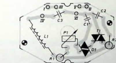
Bild 4: Ansicht der bestückten Printplatte des Lichtdimmers
