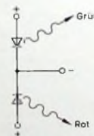
Bild 2. Ansteuerung der Lumineszenzdiode
