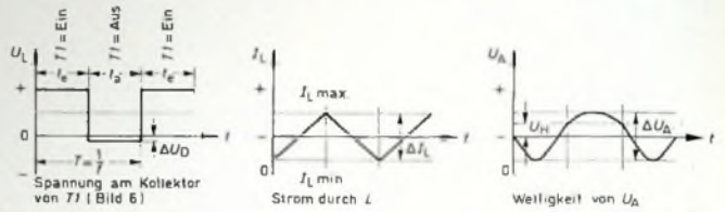
Bild 7. Schaltvorgänge im getasteten Regler; t_e Einschaltzeit, t_s Ausschaltzeit, T Impulsdauer, U_A Hysteresespannung
