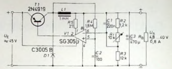
Bild 6. Getasteter Gleichspannungsregler
