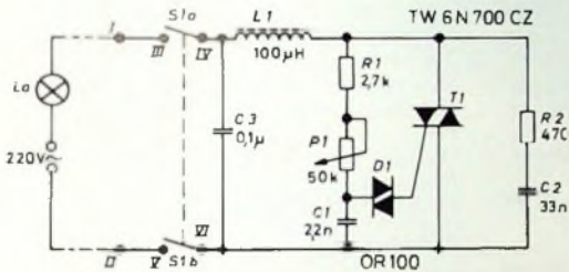
Bild 1: Schaltung des Lichtdimmers
