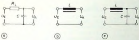
Bild 4. Mögliche Filterkombinationen: a) kapazitive Schaltung mit R_f und C , b) induktive Schaltung mit L , c) induktiv-kapazitive Schaltung mit L und C .
