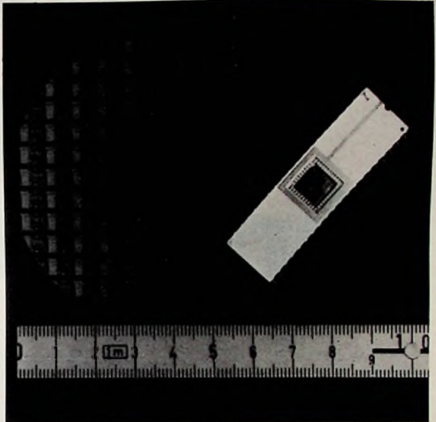
Bild 2. Ein MOS-Großschaltkreis, der auf Siliziumscheiben mit einem Durchmesser von 3 Zoll hergestellt wird und je Schaltung (rechts im Bild) 10 000 Transistorstrukturen enthält. Auf einer Scheibe sind 100 einzelne Schaltungen untergebracht.
