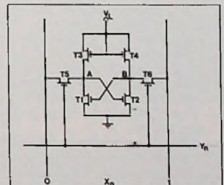
Bild 1. Schaltung einer 6-Transistor-Zelle
