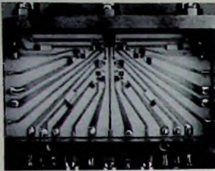
Bild 4. Substrat des Speicherschaltiodenmultiplexers
