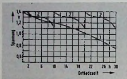
Bild 3. Vergleich der Entladekurven einer Trockenbatterie (alkalische Mignonzelle, R 6, Kurve 1) und eines maßgleichen Nickel-Cadmium-Akkumulators (KR 15/51, Kurve 2). Die Belastung beträgt in beiden Fällen 50 mA
