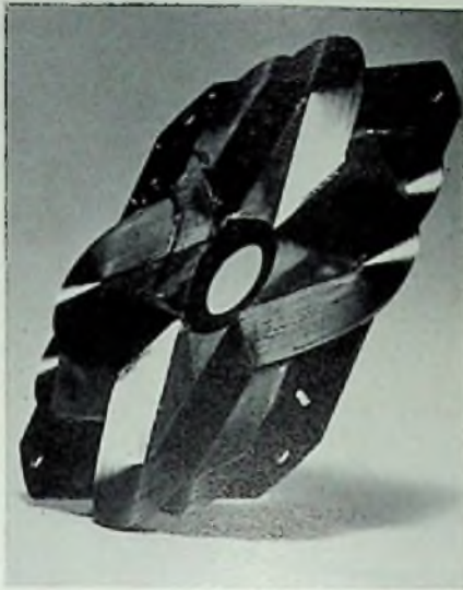
Bild 3. Unteransicht der Isolierstoff-Trägerplatte mit den beiden um 22,5° gegenüber versetzten, etwa sternförmigen Statorwicklungen
