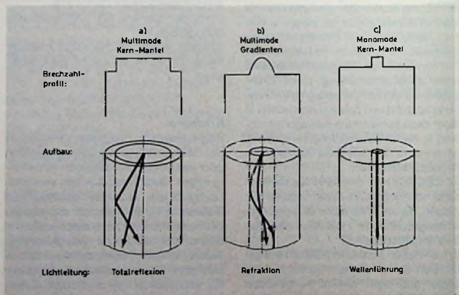
Bild 1. Lichtleitfaser-Typen
