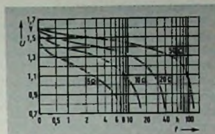
Bild 2. Gemessene Benutzungsdauer einer Braunstein-Trockenbatterie »Baby 1,5 V« (IEC-Größe R 14) in Stunden (h) bei einer Belastung von 2 Stunden je Tag (h/d)
