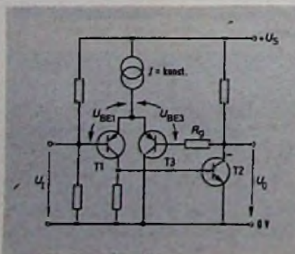
Bild 6. Grundschialtung des Differenzverstärkers
