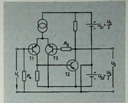
Bild 7. Differenzverstärker mit symmetrischer Spannungsversorgung
