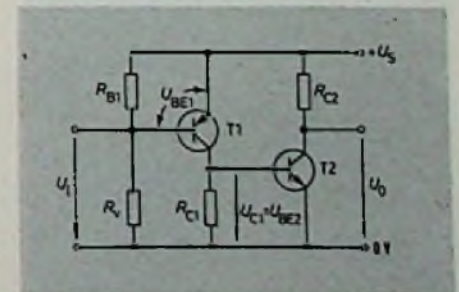
Bild 2. Gleichspannungskopplung zweier Transistoren von verschiedenem Leittyp
