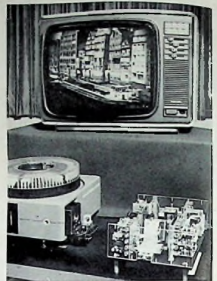
Diapositiv-Abtaster mit P 2 CCD-Zeilensensoren zu je 500 Bildpunkten (Valvo)
