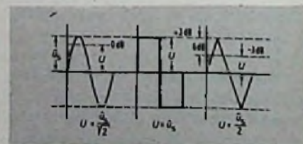
Bild 1. Gleiche Spitzenwerte, aber unterschiedliche Effektivwerte haben diese drei Signale.
