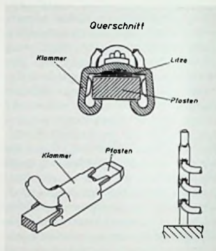
Bild 23. Termi-Point der Firma AMP
