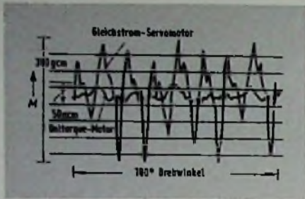
Bild 5. Vergleich der Drehmoment-schwankungen zwischen einem herkömmlichen, hochwertigen Gleichstrom-Servomotor mit 8 Polen und 24 Nuten sowie einem Uitorque-Motor. Der Uitorque-Motor zeigt eine um etwa den Faktor 6 . . . 7 bessere Laufruhe
