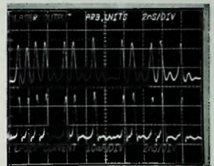
Bild 8. Modulationsstrom (unten) und Ausgangssignal des Lasers (oben)
