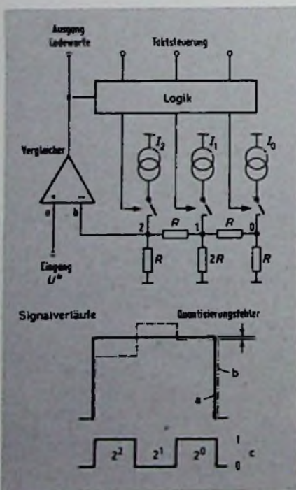
Bild 3. Bewertungscodierer mit Rückkopplung
