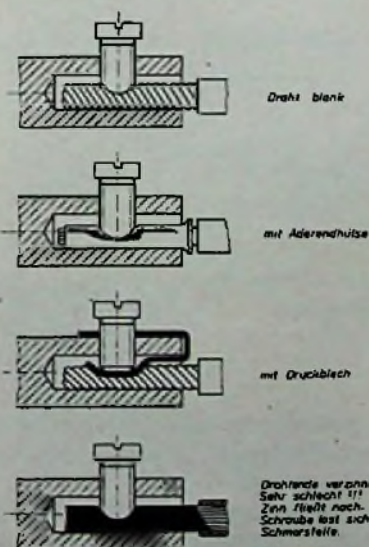
Bild 19. Drahtanschlüsse in Buchsenschaubklemmen
