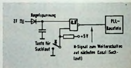
Bild 8.2. Vereinfachung der Schaltung von Bild 8.1. durch Zusammenfassen eines Inverters und ODER-Gliedes zu einem NAND-Glied
