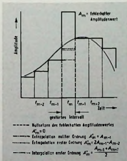
Bild 7. Fehlerüberdeckungsverfahren
