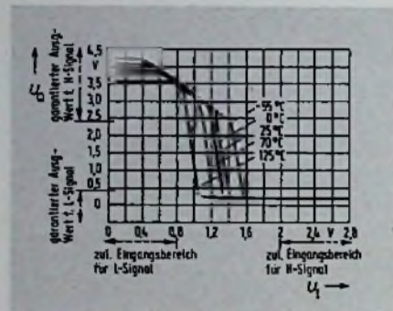
Bild 9.1.2. Charakteristisches Eingangs-Ausgangskennlinienfeld eines TTL-NAND-Gatters
