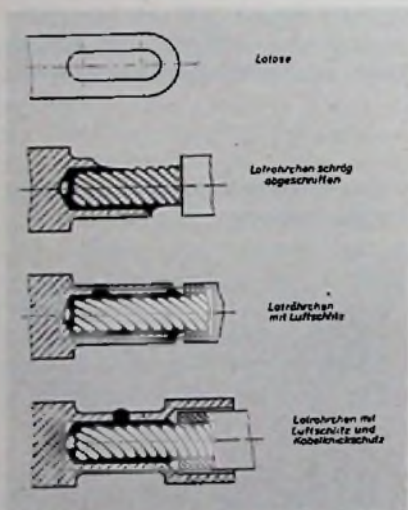
Bild 21. Lötanschluß mit Lötöse oder Lötrohrchen
