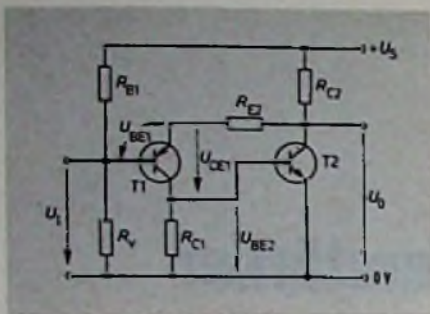
Bild 3. Gleichspannungskopplung zweier Transistoren von verschiedenem Leitwerttyp mit starker Gleichspannungsgegenkopplung
