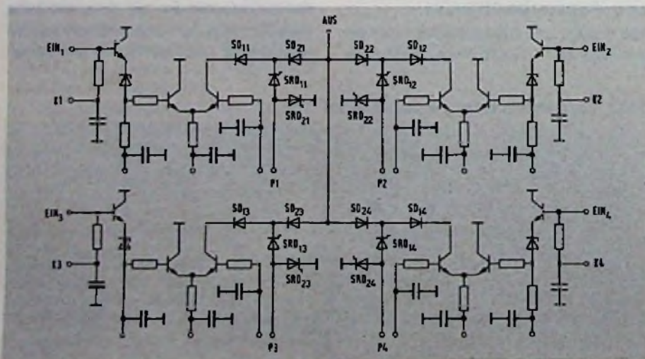
Bild 5. Schaltbild des Speicherschaltiodenmultiplexers
