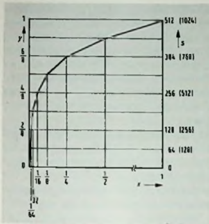
Bild 4. Logarithmische 13-Segment-Kennlinie
