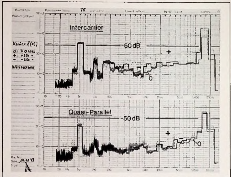
Bild 6. Vergleich der frequenzabhängigen Störspannung bei der Darstellung des Kreis-Testbildes abhängig von einer Tuner-Verstimmung um \pm 350 kHz. IC Intercarrier, QP Quasi-Parallelton
