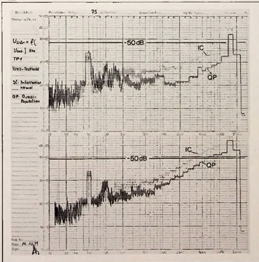
Bild 5. Terzanalyse des Störgeräusches bei der Darstellung des Kreis-Testbildes abhängig vom Wert der Antennenspannung. Oben: U_{Ant.} = 3 \text{ mV} . Unten: U_{Ant.} = 30 \text{ } \mu\text{V} . Bezugston für 0 dB mit 27 kHz Hub (1 kHz)
