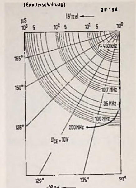
Bild 61. Rückwärtsleitwert y_{12e} nach Betrag und Phase für den HF-Transistor BF 194 (Siemens)
