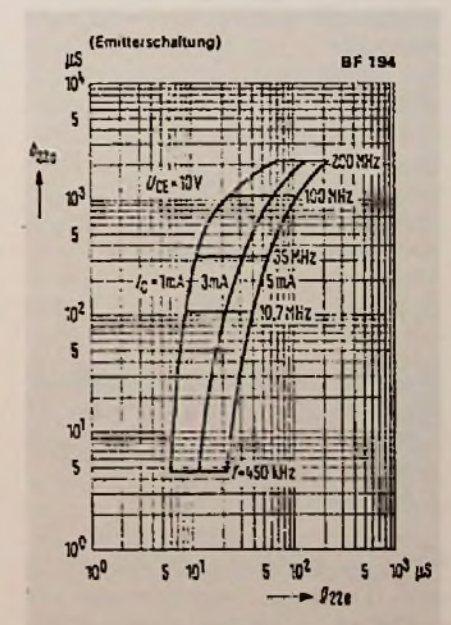
Bild 63. Ausgangsleitwert y_{22e} = g_{22e} + jb_{22e} für den HF-Transistor BF 194 (Siemens)
