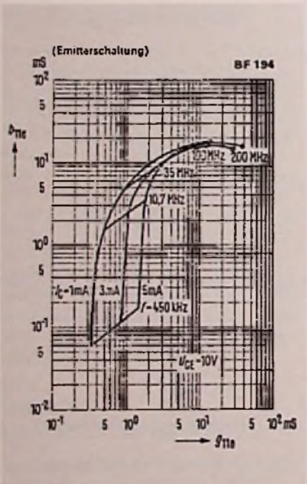
Bild 60. Eingangsleitwert y_{11e} = g_{11e} + jb_{11e} für den HF-Transistor BF 194 (Siemens)
