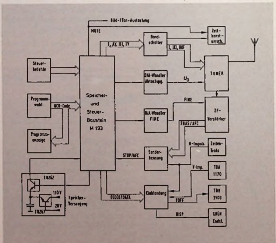
Bild 1. Blockschaltung und Signalfuß des Abstimmsystems
