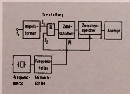
Bild 24.1. Blockschaltbild eines digitalen Frequenzmessers
