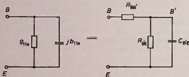
Bild 65. Ersatzschaltung des Transistoreinganges zur Berechnung des Basisbahnwiderstandes
