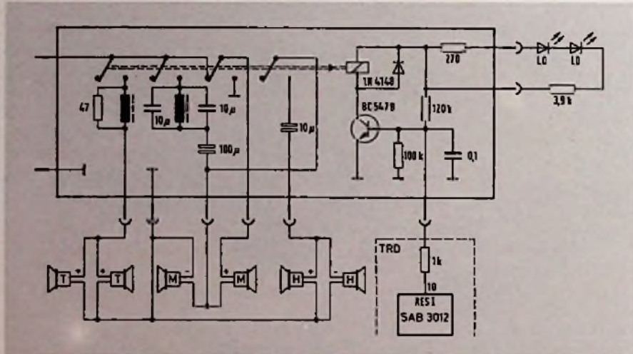
Bild 9. Stromlauf der Supradyn-Lautsprechermatrix und der Einrichtung zum elektronischen Umschalten von Normal- auf Raumton
