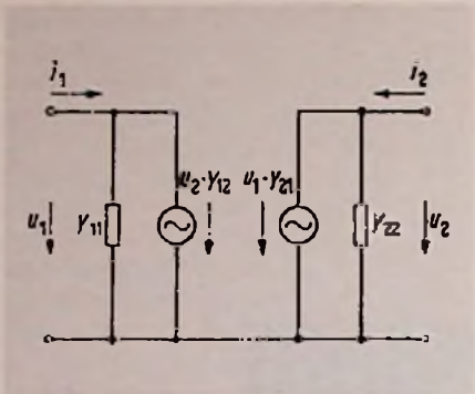
Bild 59. Leitwert-Ersatzschaltbild eines Transistors (Siemens)
