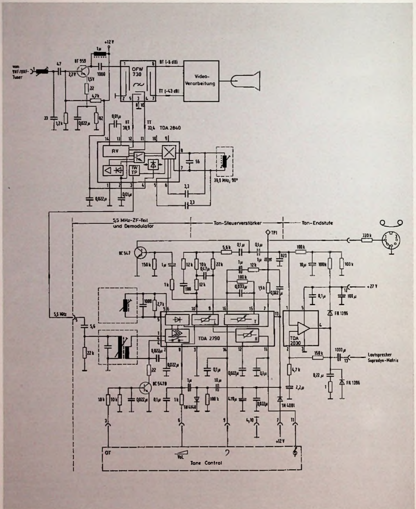
Bild 3. Stromlauf des ZF/NF-Teils von Supradyn-Fernsehempfängern. Ein Aufzeichnen des Fernsehtons oder die Wiedergabe über einen getrennten Verstärker ermöglicht die 5polige Normbuchse
