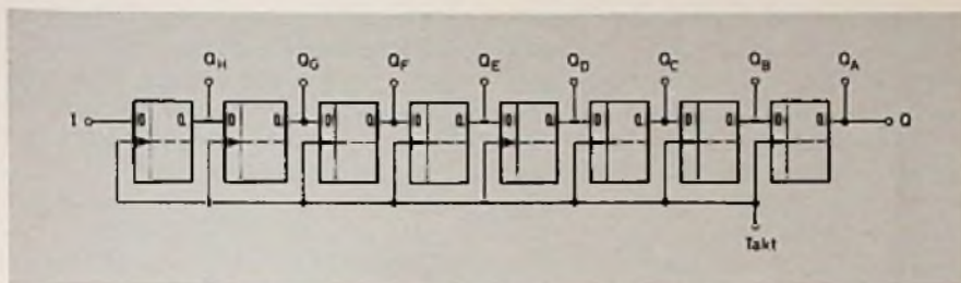
Bild 25.1. Durch die Reihenschaltung von 8 D-Flip-Flops entsteht ein 8-bit-Schieberegister
