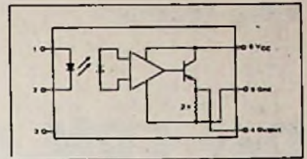
Blockschaltung des linearen Optokopplers MOC 5010 (Motorola GmbH)
