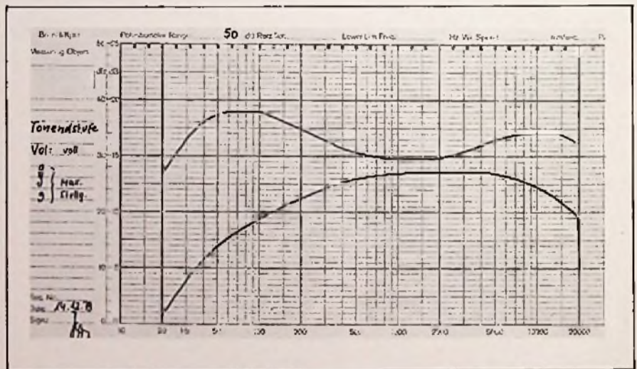
Bild 7. Stellbereich des Höhen- und Tiefenstellers in Supradyn-Fernsehempfängern
