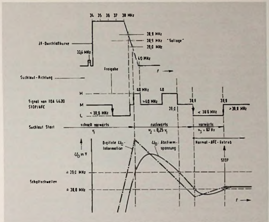
Bild 2. Oben: Fest vorgegebene ZF-Kurve. Mitte und unten: Signale beim „Stoppen“ auf einen Fernsehsender. Die Suchlaufrichtung gibt an, daß ein Sender in den niederfrequenten Teil der ZF-Kurve „einläuft“. Daraus resultieren die übrigen Signalverläufe
