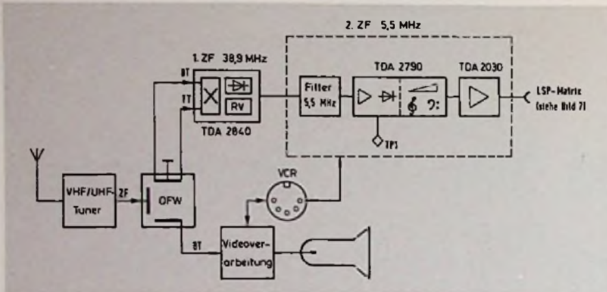
Bild 1. Stark vereinfachte Blockschaltung eines Supradyn-Fernsehempfängers mit Quasi-Parallelton. RV Regelverstärker, OFW Oberflächenwellenfilter, VCR normgerechter Aufnahme- und Wiedergabeanschluß für Videorecorder.
