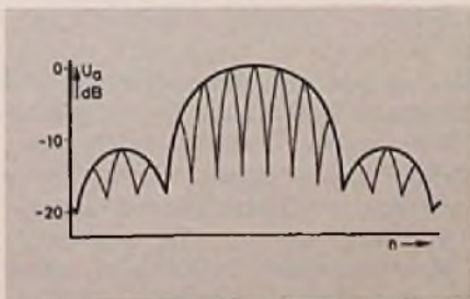
Bild 3. Beim „taumeln“ des Wiedergabekopfes muß auf das Hauptmaximum der Ausgangsspannung eingestellt werden
