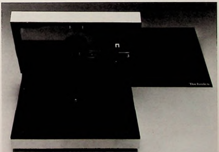
Technics-Plattenspieler „SL-10“ in geöffnetem Zustand
