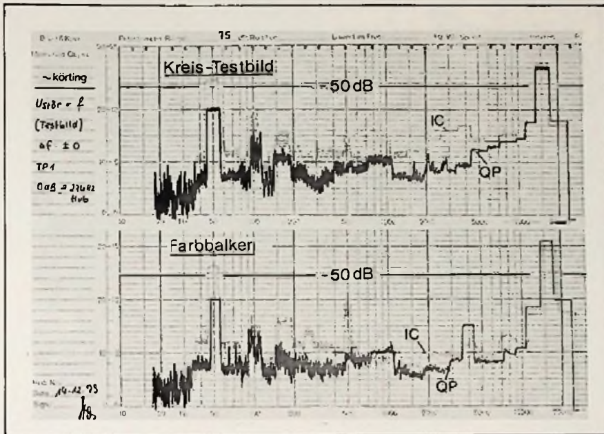
Bild 4. Terzanalyse des testbildabhängigen Störgeräusches beim Intercarrier- und Parallelton-Verfahren. U_{Ant.} = 10 \text{ mV} , Bezugston 27 kHz Hub, Messung am Testpunkt TP1
