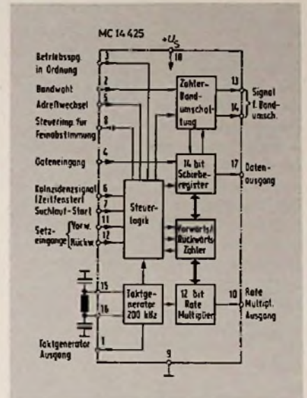
Bild 26.4. Blockschtung des ICs MC 14425
