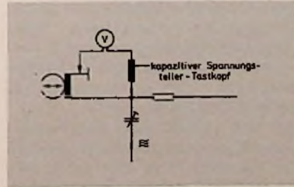
Bild 4. So wird der Wert des Vormagnetisierungsstroms mit dem kapazitiven Spannungsteiler-Tastkopf ermittelt
