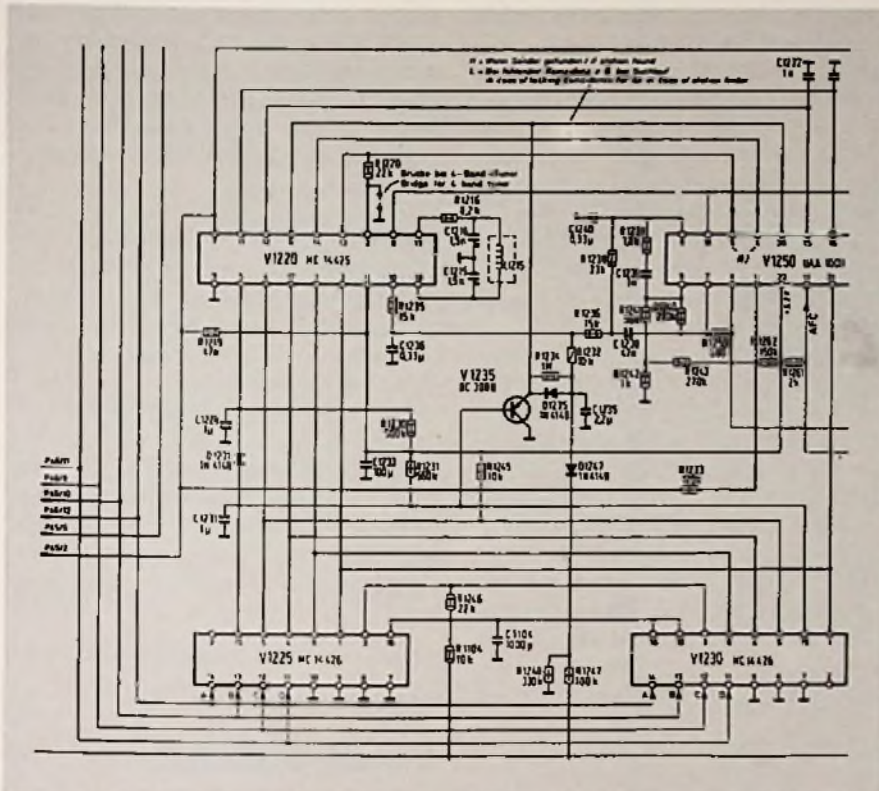
Bild 26.3. Schaltungsauszug aus dem Siemens-Farbfemsehempfänger Bildmeister FC 442
