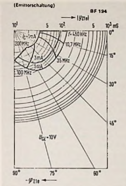
Bild 62. Vorwärtssteilheit y_{21e} nach Betrag und Phase für den HF-Transistor BF 194 (Siemens)
