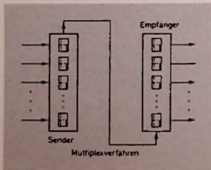
Bild 26.2. Mit dem Multiplexverfahren und einem als Parallel-Serien-Wandler arbeitenden Schieberegister genügt eine Leitung zwischen Sender und Empfänger
