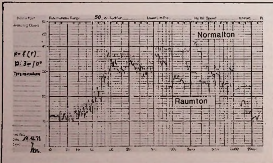
Bild 10. Schalldruck als Funktion der Tonfrequenz in den Betriebsarten Normal- und Raumton. Das Meßmikrofon befand sich 3 m vor dem Bildschirm
