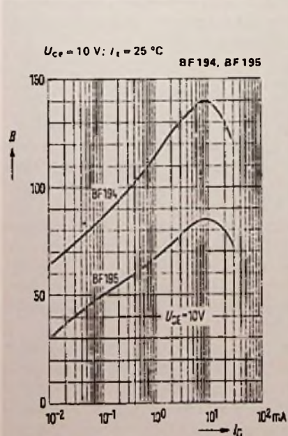
Bild 66. Stromverstärkung B = f(I_C) für den HF-Transistor BF 194 (Siemens)
