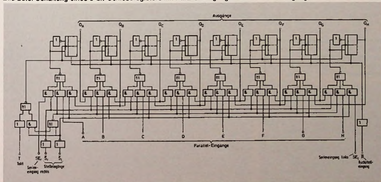
Bild 25.3. Schaltung eines 8-bit-Schieberegisters mit Parallel-Eingängen und Parallel-Ausgängen
