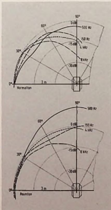
Bild 11. Richtcharakteristik des Schalldrucks abhängig von der Tonfrequenz in den Betriebsarten Normal- und Raumton. Das Meßmikrofon befand sich 3 m vor dem Bildschirm
