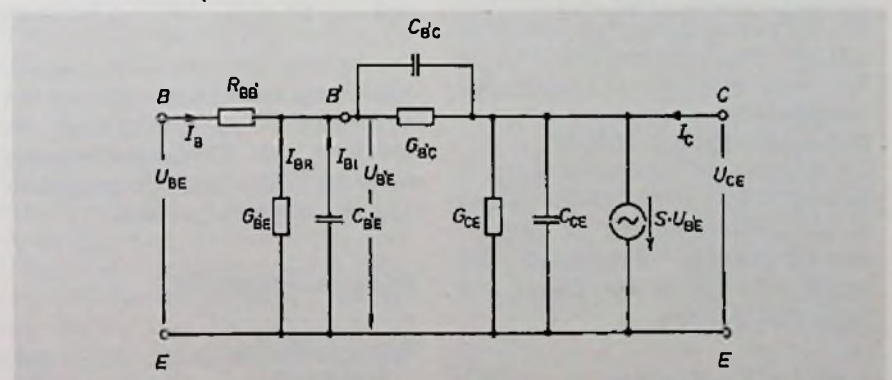
Bild 58. Hochfrequenzersatzschaltbild eines Transistors nach Giacoletto
