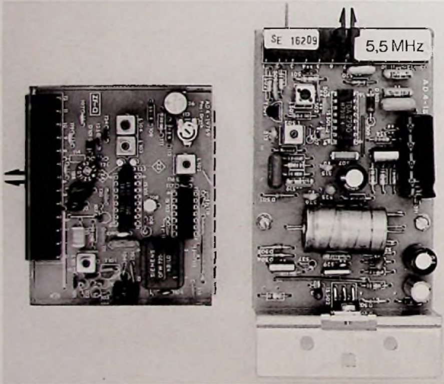
Bild 2. Links: ZF-Modul (ZF-Q) für Quasi-Parallelton. Rechts: 5,5-MHz-ZF-Modul mit monolithisch integrierter 15-W-Tonendstufe
