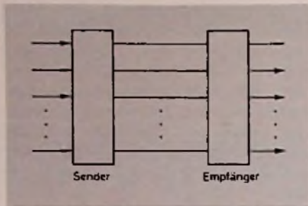
Bild 26.1. Bei der parallelen Übertragung eines Datenwortes mit einer Wortlänge von 32 bit sind zwischen Sender und Empfänger auch 32 Leitungen notwendig
