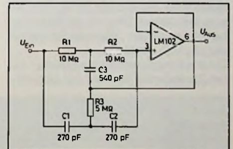
Bild 1: Kerbfiler für 60 Hz
