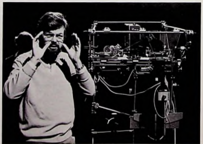
Bild 2: Fernseh-Doppelkamera für die 3-D-Fernsehsendung (Foto: NDR/v. Estor)
