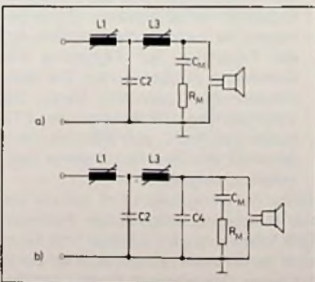
Bild 7. Filterschaltungen für D-Verstärker
