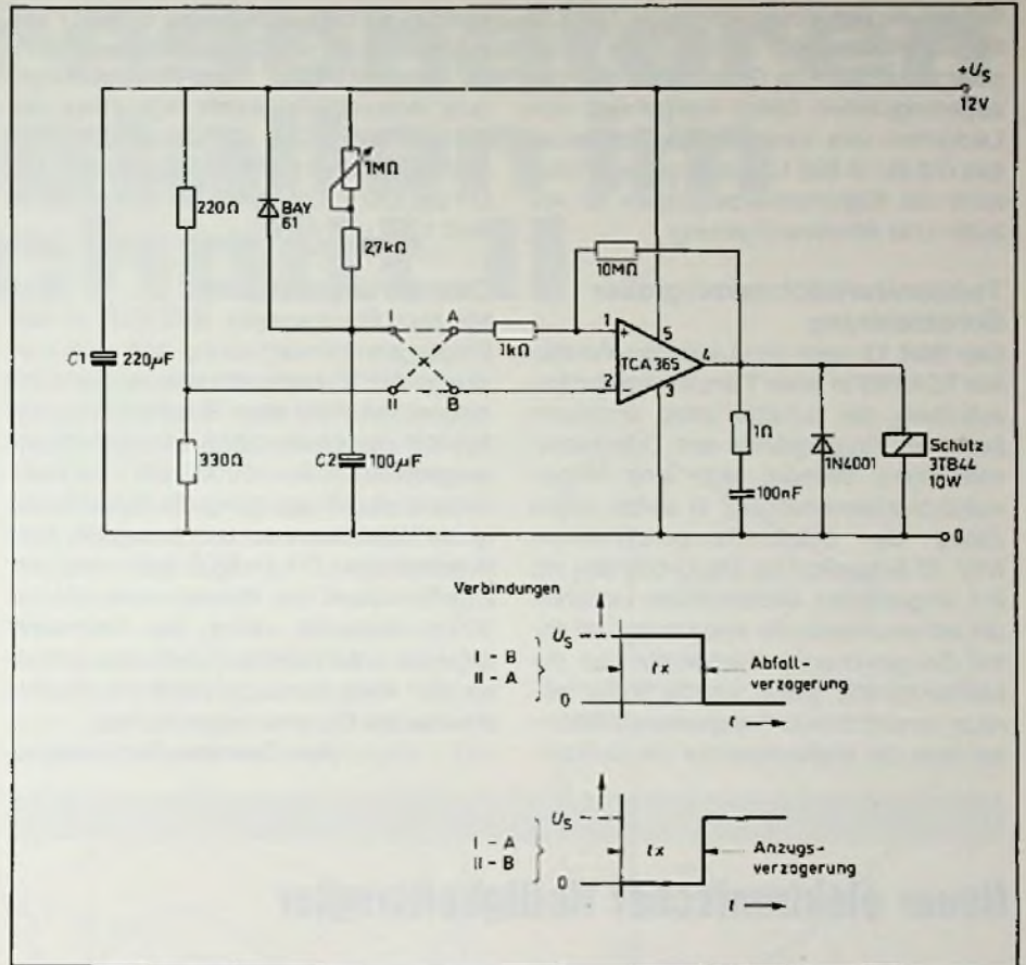
Bild 12: Verzögerungsschaltung für 0,2 bis 100 s mit TCA 365
