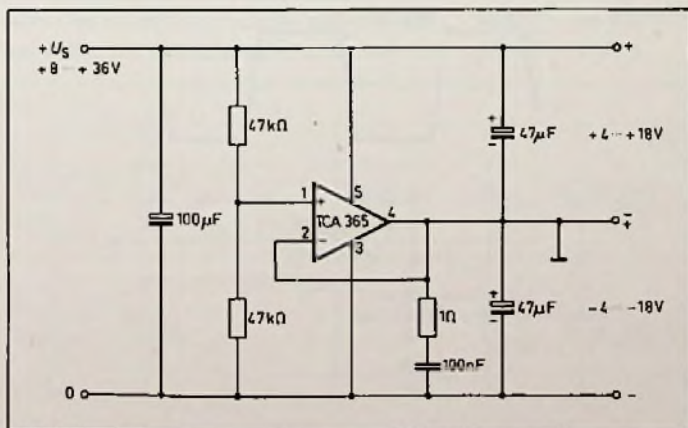
Bild 7: Symmetrische Spannungsversorgung
