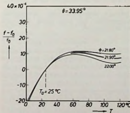
Bild 9: a) Berechnete Temperaturgänge für \phi = 21,90^\circ und eine Reihe von \Theta -Werten. b) Berechnete Temperaturgänge für \Theta = 33,93^\circ\text{C} bei drei Werten von \phi .
