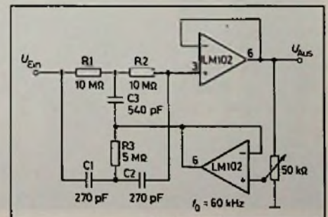
Bild 2: Kerbfiler mit variabler Güte
