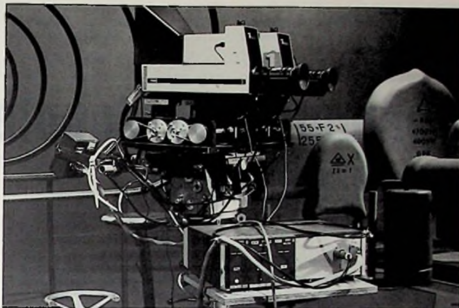
Bild 3: Versuchsmuster einer aus zwei Einzelkameras bestehenden 3-D-Kamera
