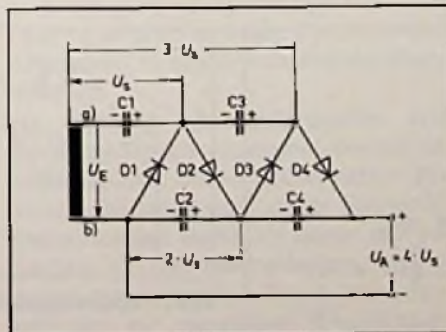
Bild 5. Spannungsvervielfacher nach Villard
