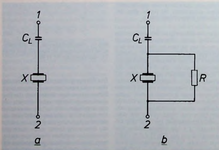
Bild 15: Der Resonanzteil einer Oszillatorschaltung.
