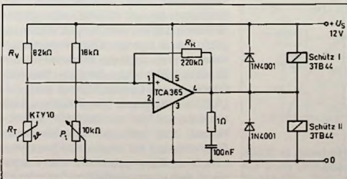
Bild 13: Temperaturwächterschaltung
