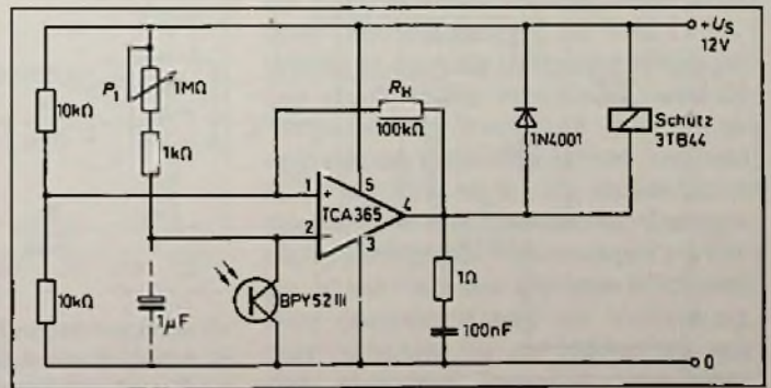
Bild 14: Dämmerungsschalter für 10 bis 10 4 s
