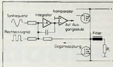
Bild 8. D-Verstärker, Gesamtanordnung
