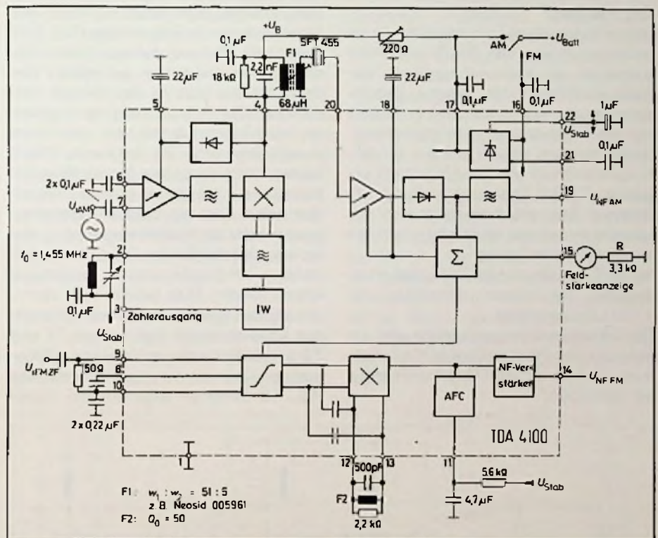
Bild 1: Blockschaltbild des integrierten AM/FM-Schaltkreises TDA 4100
