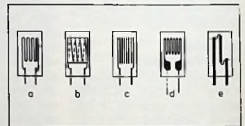
Bild 7: Ausführungsformen von Dehnungsmeßstreifen. a) Mäander b) Wendel c) Gitter mit niederohmigen Querstegen d) Folien- oder Schicht-DMS mit niederohmigen Querstücken e) Halbleiter-DMS
