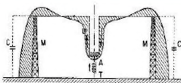
Fig. 3. — Le fonctionnement du réseau des antennes (Coupe schématique en diagonale).
