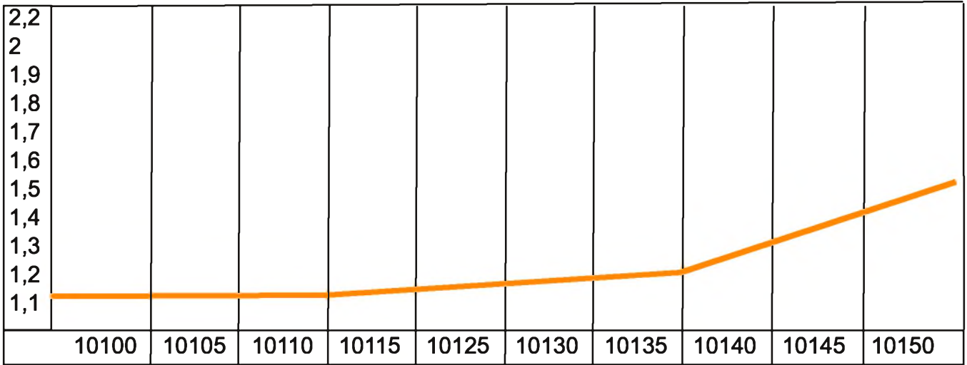
COURBE DU ROS SUR LA BANDE DES 10 MHZ ANTENNE 7 BANDES MONTEE EN V INVERSE
