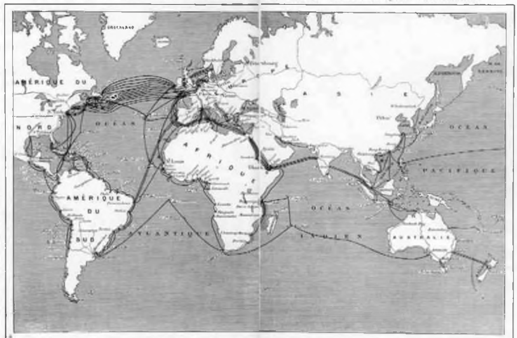
CARTE COMPLETE DU RESEAU INTERNATIONAL DES CABLES TELEGRAPHIQUES SOUS-MARINS
