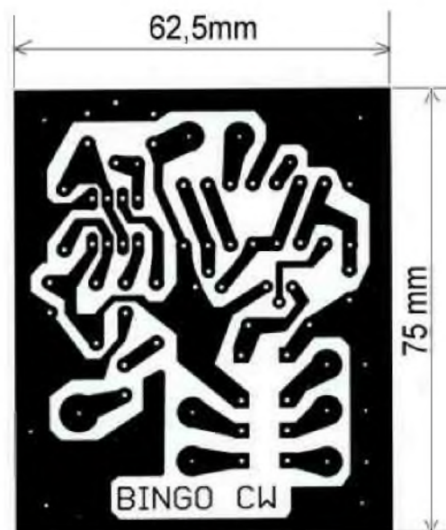
circuit commande côté cuivre
