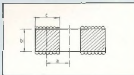
Vue en coupe du bobinage.
