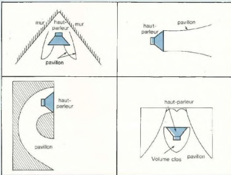
Enceintes à pavillon.
