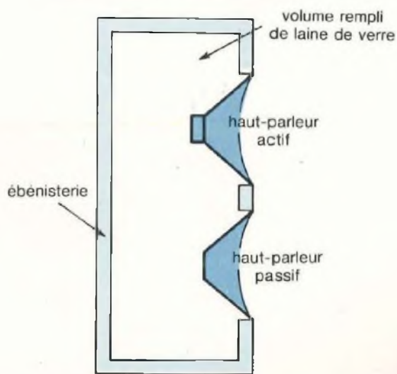
Coupe d'une enceinte actif-passif.
