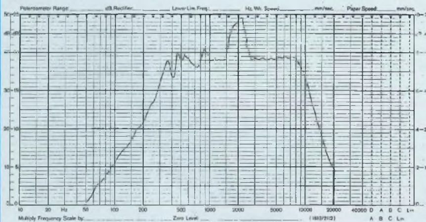
Courbe d'un haut-parleur.
