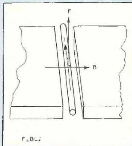
Fonctionnement électro-magnéto-mécanique.
