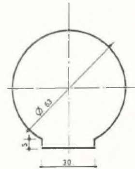
PLAN DE PERCAGE DU TWEETER
