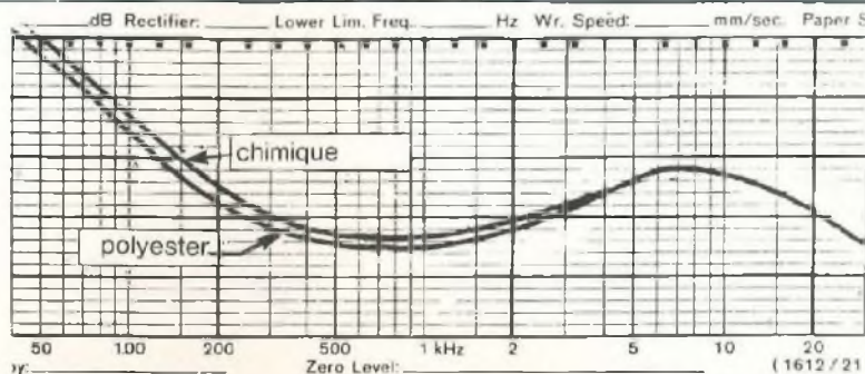
La courbe d'impédance présentée est celle d'un tweeter seul ou filtré par un condensateur de 10 \mu\text{F} polyester, puis bipolarisé. Noter la perte d'insertion différente entre 3 000 Hz et 30 000 Hz.
