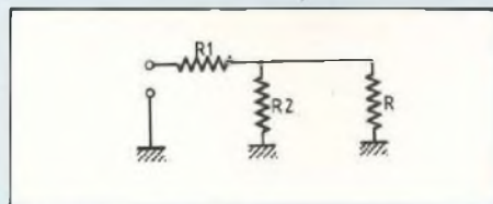
Réseau d'atténuation.
