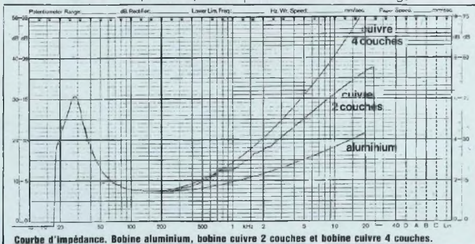
Courbe d'impédance. Bobine aluminium, bobine cuivre 2 couches et bobine cuivre 4 couches.
