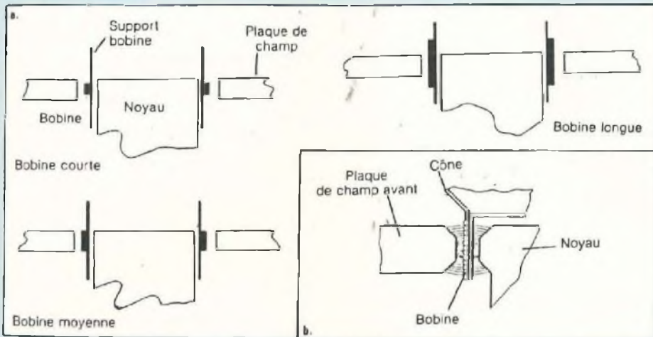
a) Les trois types de bobines
