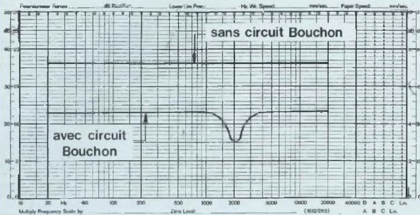
Courbe amplitude-fréquence d'un circuit bouchon-série.
