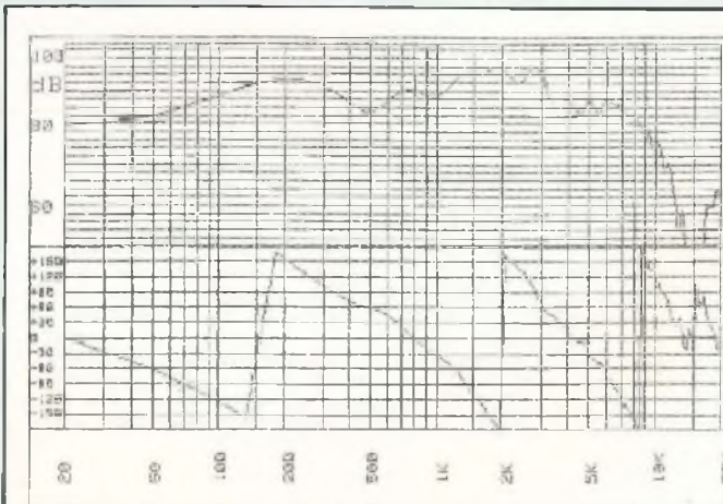
Fig. 1 : Courbes amplitude-fréquence et phase fréquence réalisées à partir d'un ordinateur. La courbe est obtenue par transformée de Fourier d'un signal impulsionnel (signal carré de 10 \mu s).
