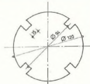
PLAN DE PERCAGE D'UN BASSE
