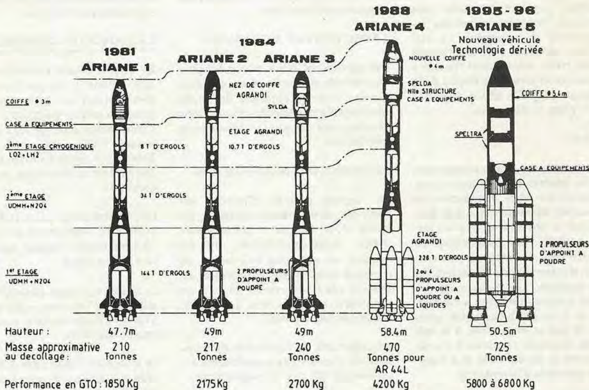
Evolution des lanceurs : d'ARIANE 1 à ARIANE 5
