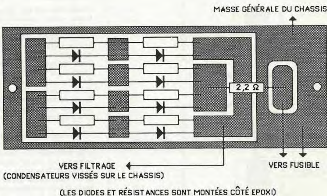
Figure 4 : Implantation des composants sur le circuit imprimé de l'alimentation
