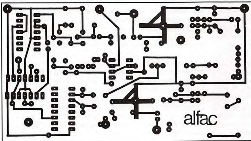
Figure 11 : Oscillateurs.
