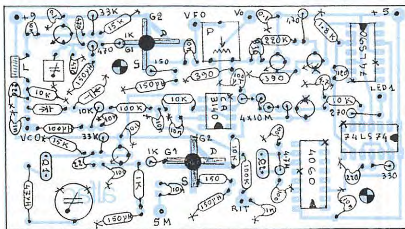
Figure 13 : Implantation Oscillateurs.
