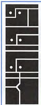
Face cuivre côté composants sauf 3 LED.
