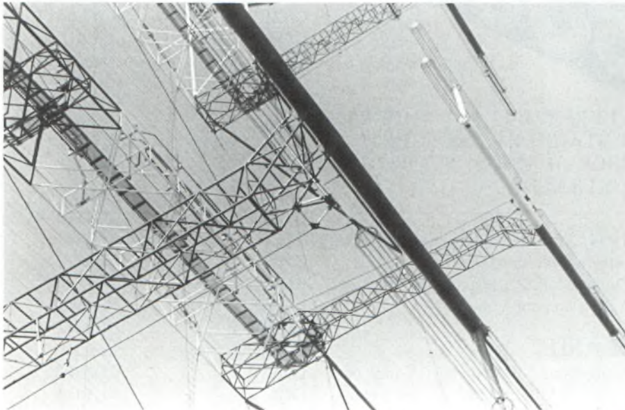
Détail sur les dipôles
