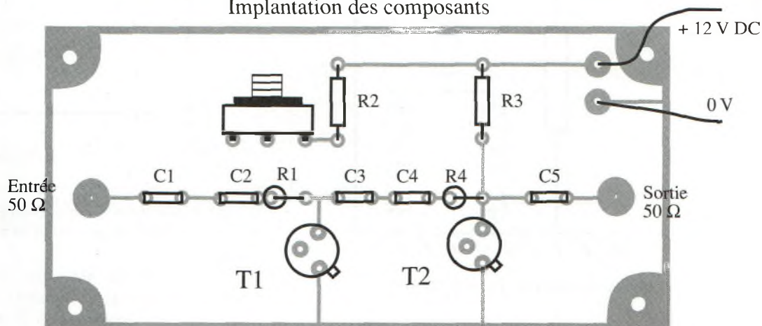
Implantation des composants
