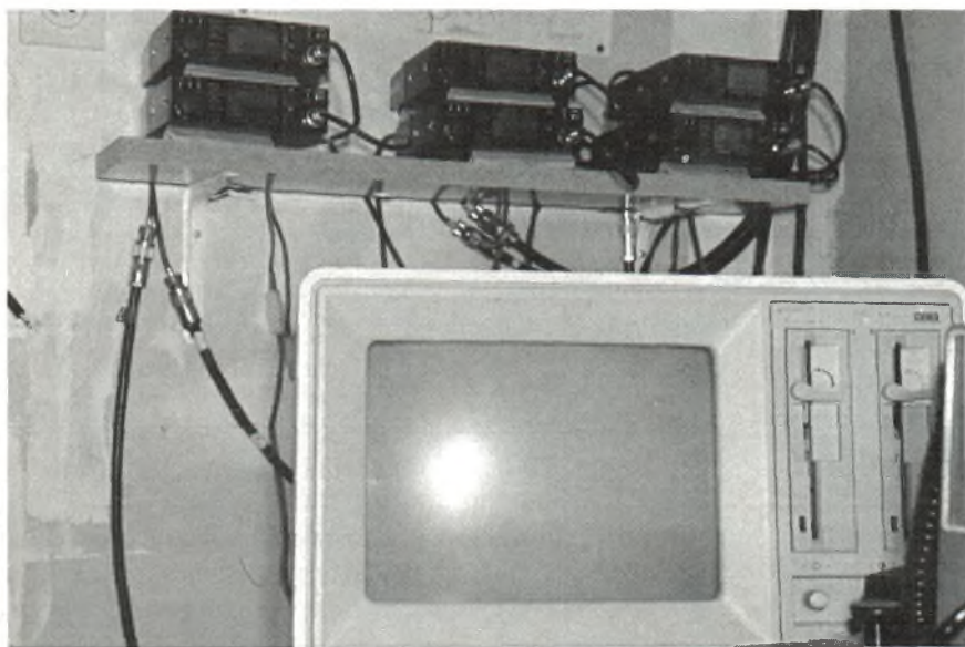
Un node Fpac à six voies. (photo JG)
