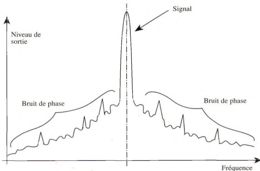
Bruit de phase d'un synthétiseur PLL
