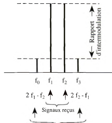
Signaux générés par intermodulation du 3 e ordre
