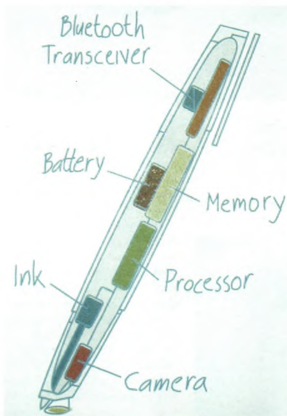
Un synoptique « très allégé » de ce stylo sans fil.
