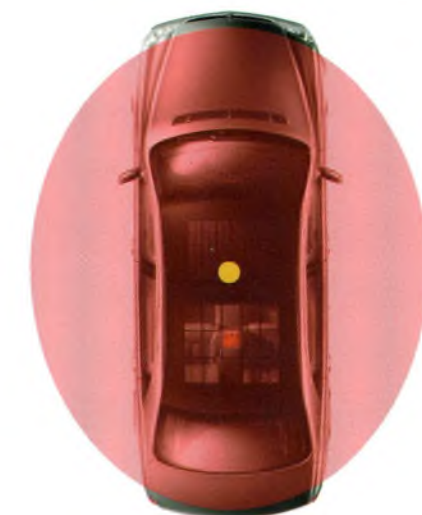
Antenne au centre : le diagramme est presque omnidirectionnel.
