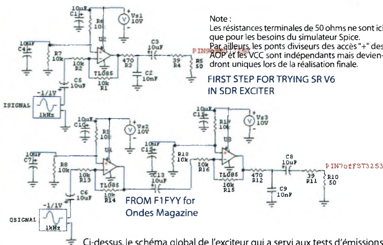
Ci-dessus, le schéma global de l'excitateur qui a servi aux tests d'émissions avec le SRV6. Nous y reviendrons dans la troisième partie de cette série consacrée à la revitalisation des transceivers
