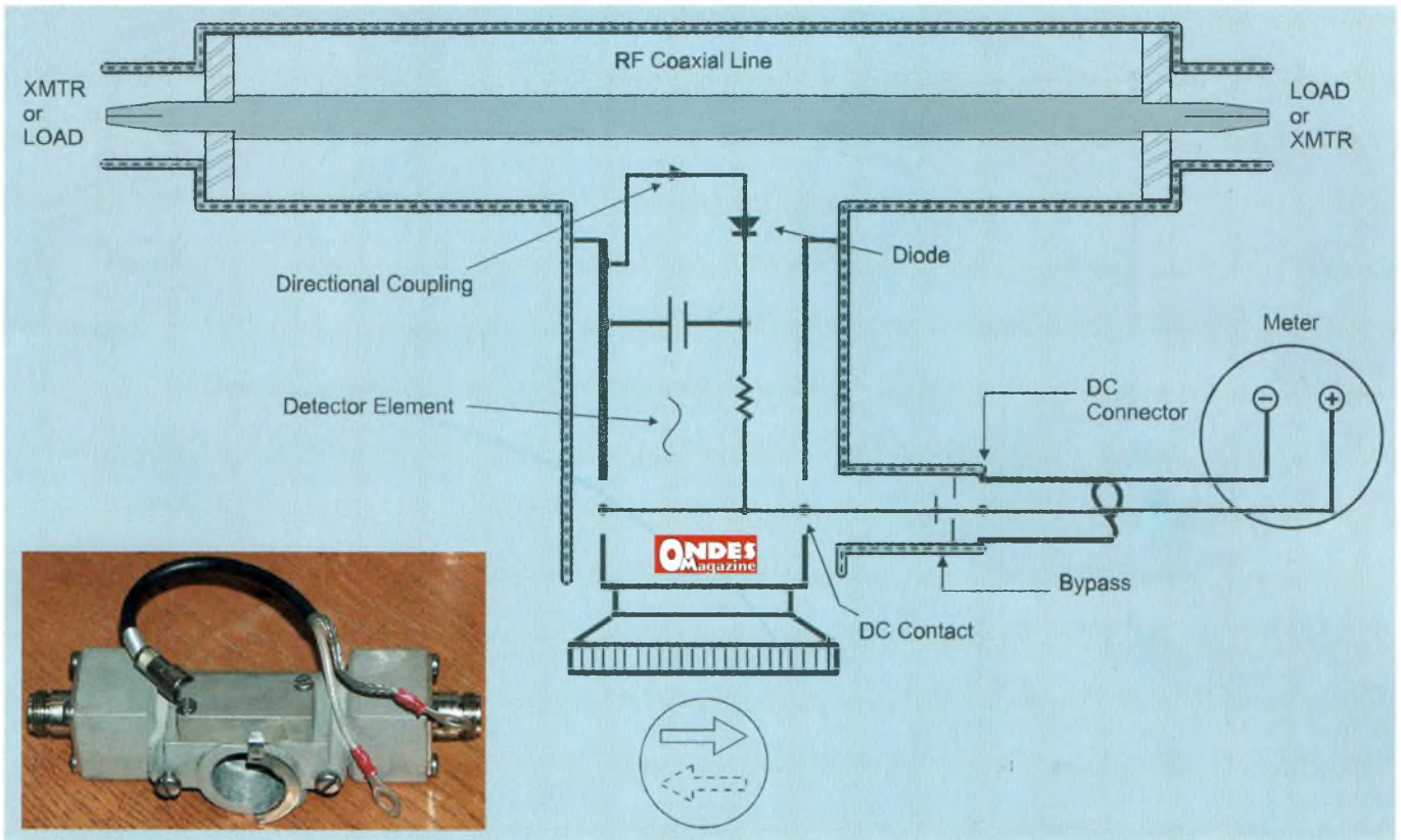
On voit ici le principe sur lequel repose l'acquisition des valeurs directes ou réfléchies. Il s'agit d'un échantillonnage des tensions et courants traversant la ligne principale de 50 ohms par l'intermédiaire d'une ligne de faible longueur. Les tensions directe et inverse détectées sont en fait le reflet des courants circulant dans la ligne. Selon les phases, ils se composent soit des différences pour les valeurs réfléchies, soit des sommes pour celles incidentes.
