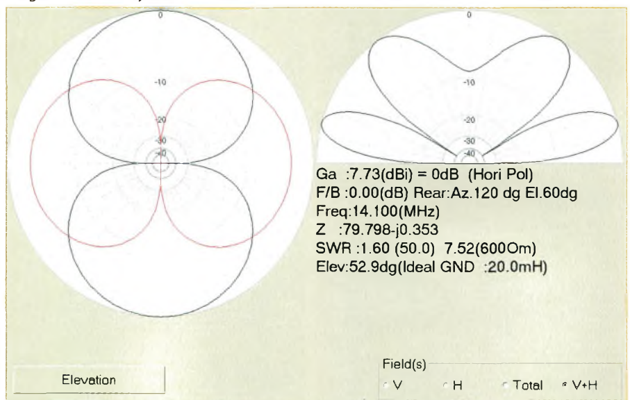
Doublet à 20 mètres - \lambda -
