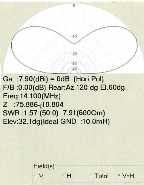
Ci-dessous : Doublet à 10 mètres -λ/2-
