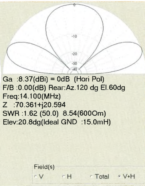
Ci-dessus : Doublet à 15 mètres -3λ/4-
