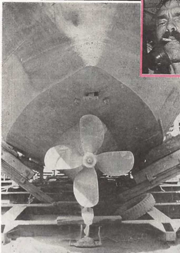
Lors du dernier passage en dock du LITTLE GIANT la nouvelle hélice. Diamètre 1,46 m - Poids 300 ou 400 kg le safran n'est pas encore remontée.
