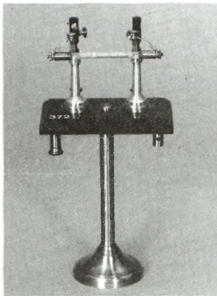
Le fameux cohéreur de Branly (1895)
