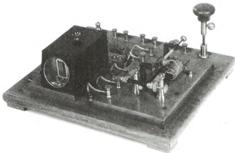
Récepteur télégraphique Ducretet avec cohéreur (1899)
