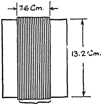
53 turns 20 D.C.C.
