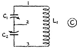
FIG 9A—HARTLEY & COLPITS
