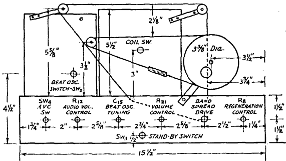
FIG. 2—FRONT LAYOUT-SKETCH
