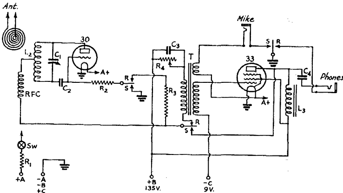
FIG. 1—"MINUTE MAN" TRANSCIEVER
