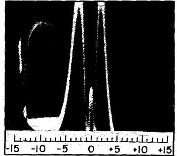
(f) REJECTION AT -0.5 KC. AND +0.5 KC.
