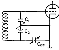
Fig. 3—Fundamental r.f. amplifier circuit.
