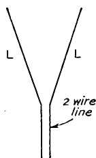
Fig. 4 — The V antenna.
