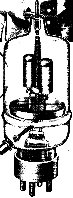
EIMAC 152T POWER TRIODE
