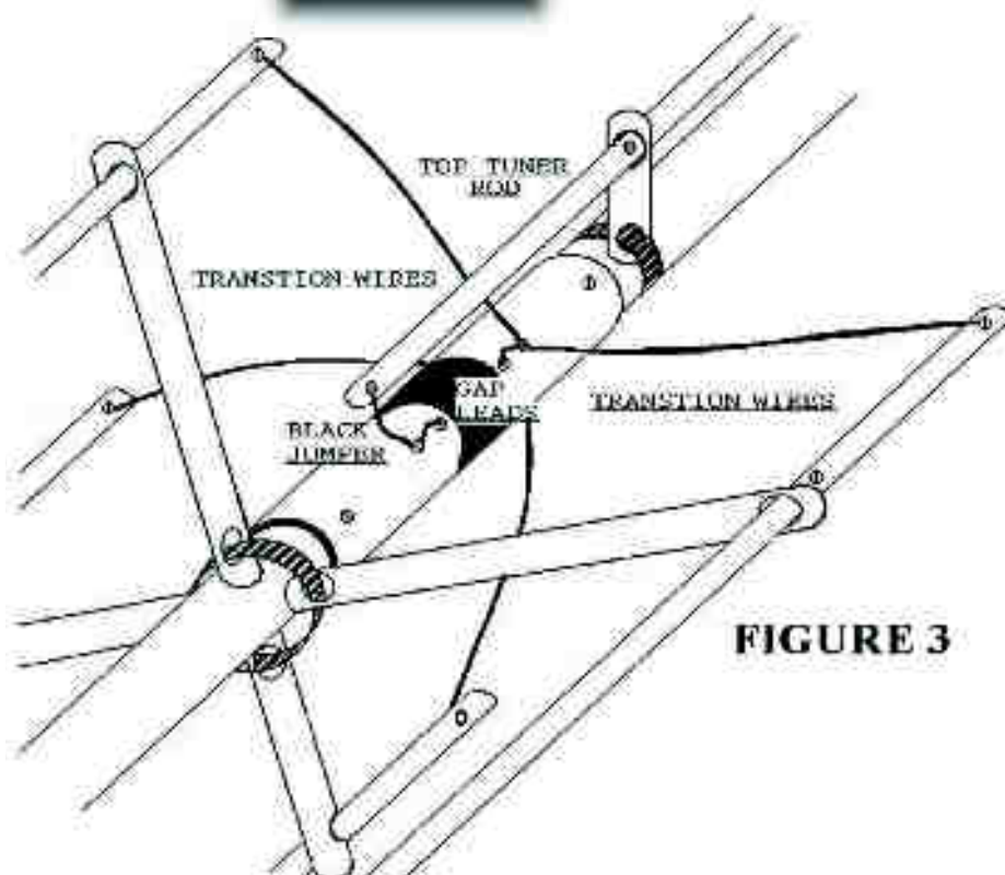
Une fois le boom principal assemblé on vient y fixer les tubes en plastique qui recevront ceux en aluminium. Ci-dessous, l'un des dessins de la notice.
