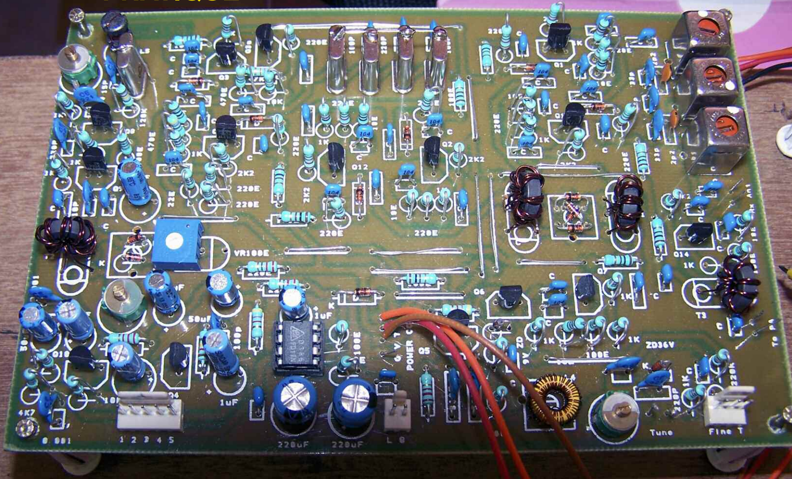
La platine générateur BLU terminée.
