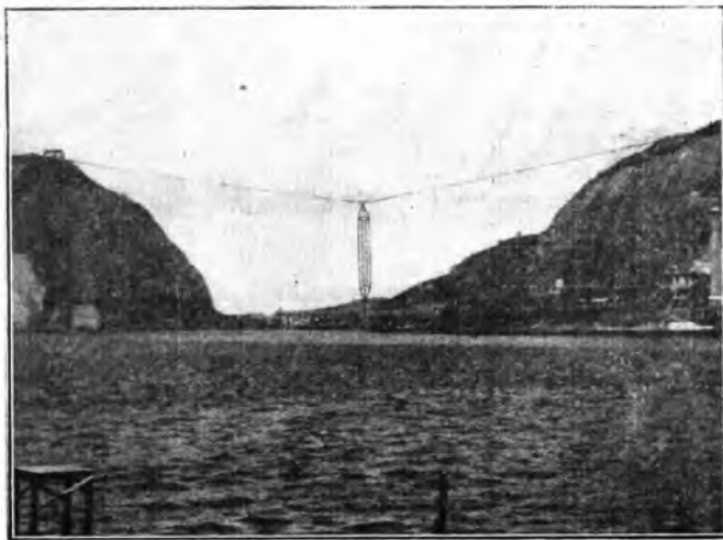
Ecco l'originale antenna della stazione radiofonica brasiliana di Praia Vermelha a Rio De Janeiro. E' tesa fra la montagna di Urca (a sinistra) e quella di Babilonia (a destra), senza alcun palo di sostegno. La parte dell'antenna a forma di gabbia verticale, misura 100 metri d'altezza. ( Radio et Sciences )
