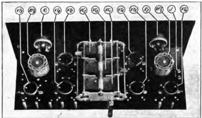
Interno Apparecchio ATLAS 6 volv.
