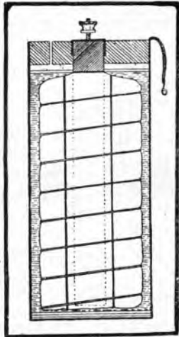
Fig. 8. — La pila a secco: il recipiente di zinco costituisce l'elemento positivo o polo negativo.
