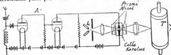
Fig. 4. — Dispositivo ricevitore: A amplificatore a B.F. — L lampada ad arco — T tamburo portante la carta fotografica.
