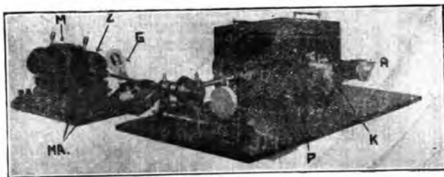
Fig. 5. — Complesso ricevente: M motore a corr. cont. — Z ruota a denti — L lampada al neon — P Nicol polarizzatore (interno al tubo) — K cella Karolus — A Nicol analizzatore e prisma a riflessione totale.
