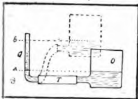
Fig. 6. — Paragono idraulico del potenziale elettrico.
